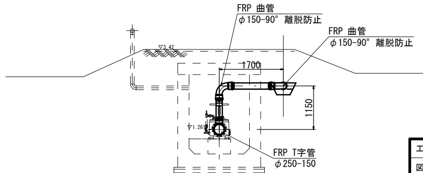
C-C断面 S=1:50
