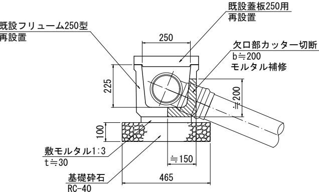
既設フリーム再設置
