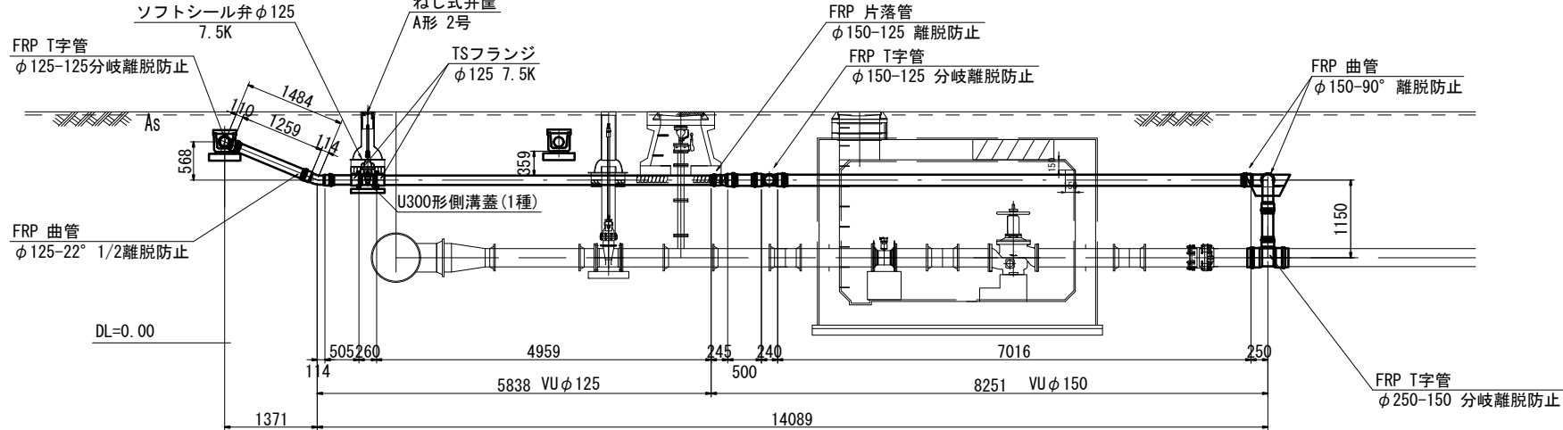
A-A断面 S=1:50
