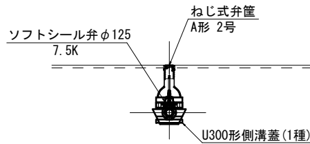
E-E断面 S=1:50
