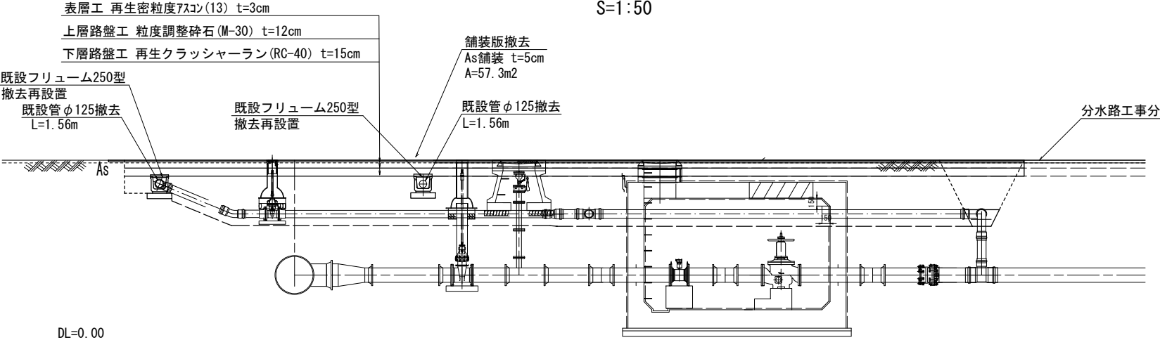
A-A断面
