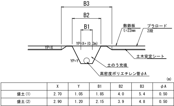
暗渠排水路横断部断面図
