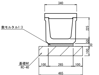
フリューム250撤去 S=1:10
