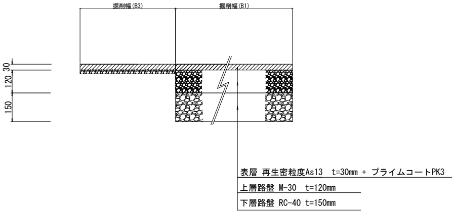
アスファルト舗装仮復旧幅員
