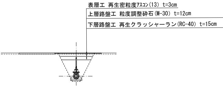
C-C断面
