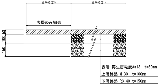
アスファルト舗装撤去幅員
