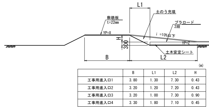
土工用進入口 道路横断面断面図
