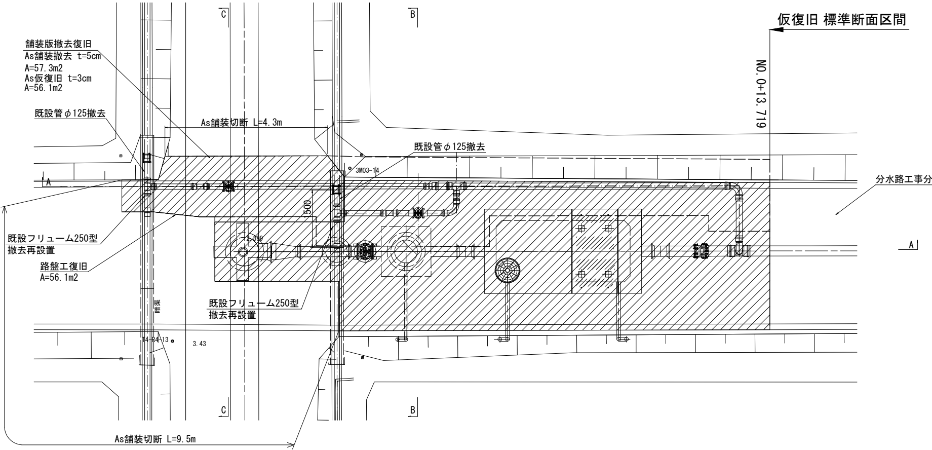
平面図
