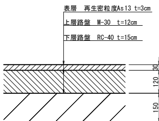
アスファルト舗装仮復旧 S=1:10
