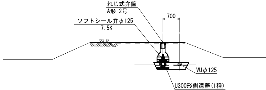
D-D断面 S=1:50
