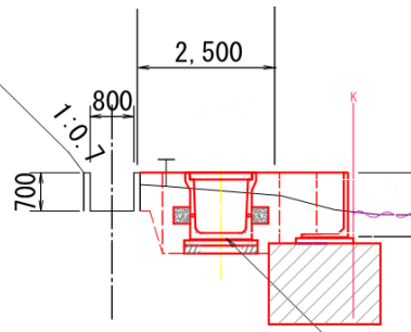
区間② 構想設計断面図
