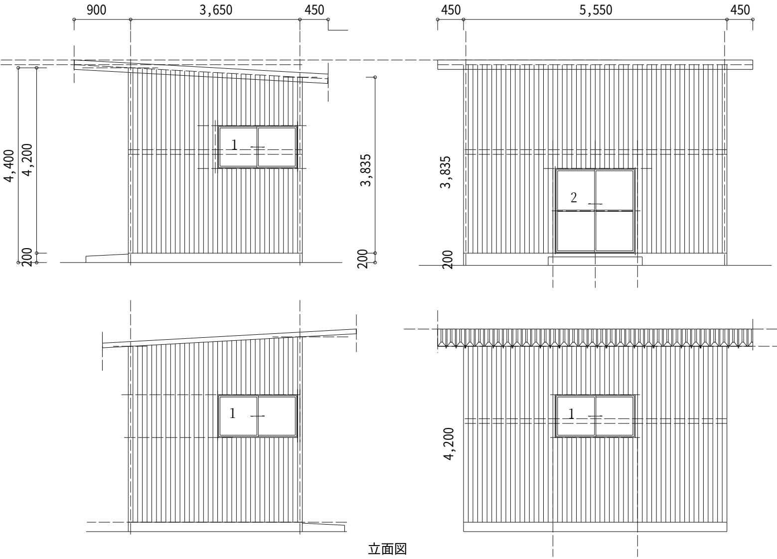
鉄骨倉庫(片流屋根)
