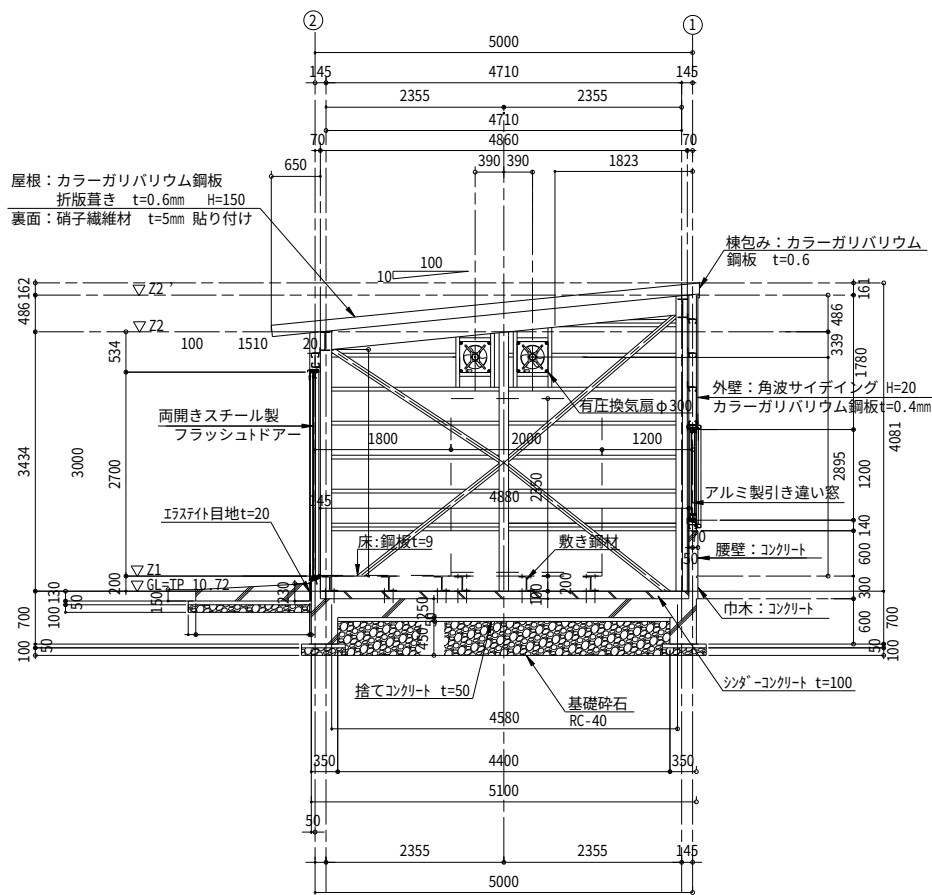
A-A 断面図
