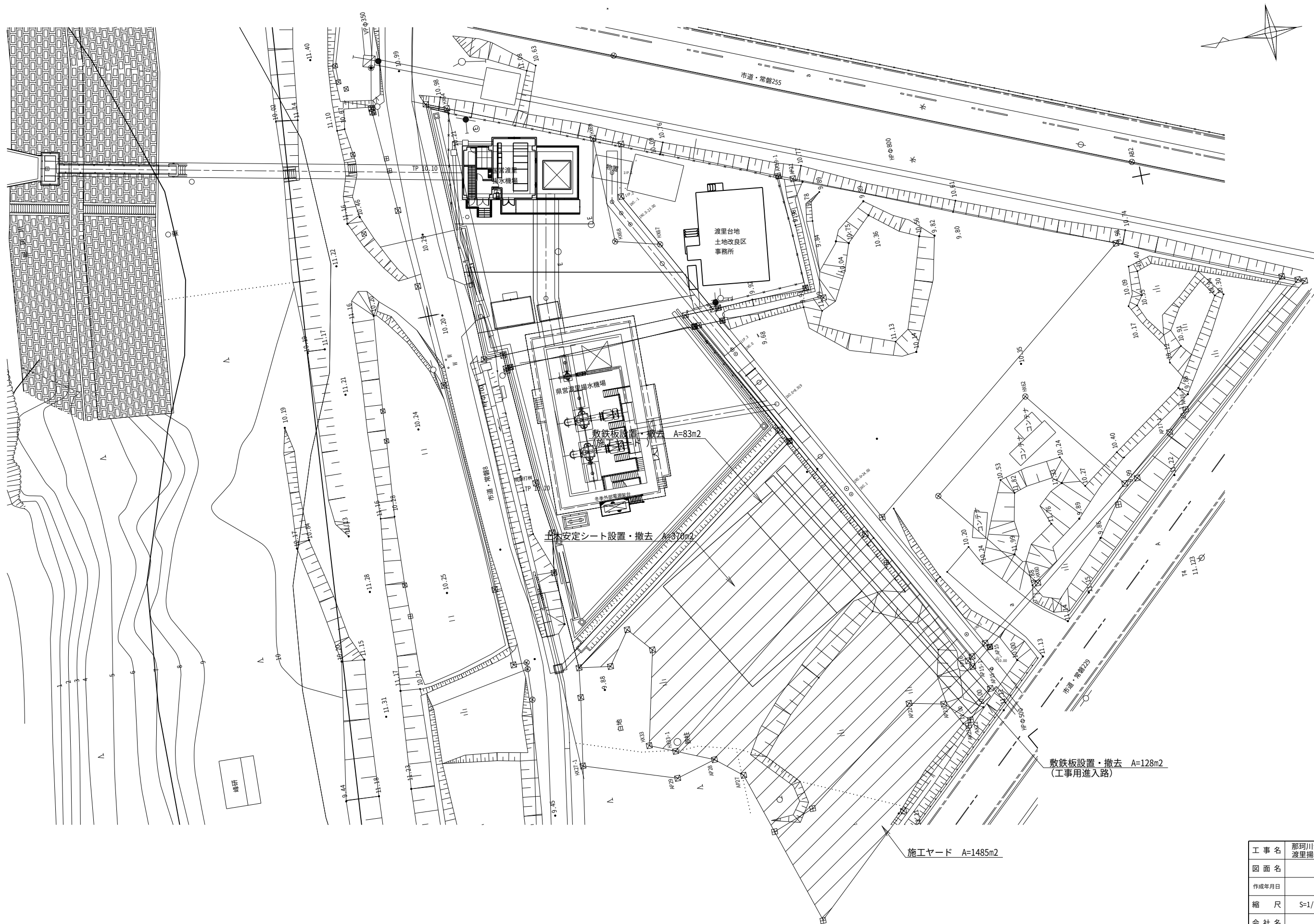
仮設工平面図
