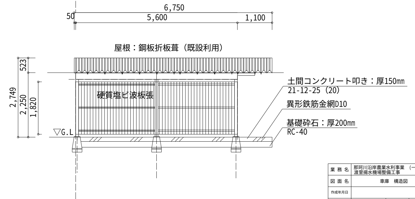
C面立面図
