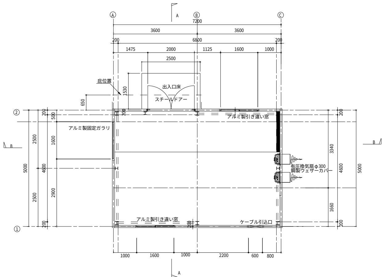
仮設電気室1F平面図
