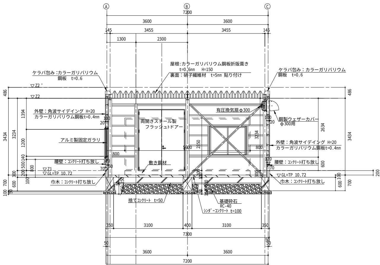
B-B 断面図
