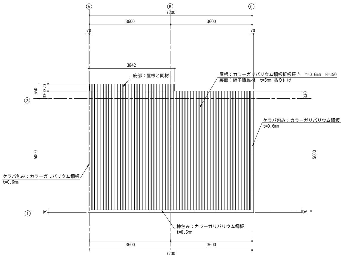
仮設電気室屋根平面図
