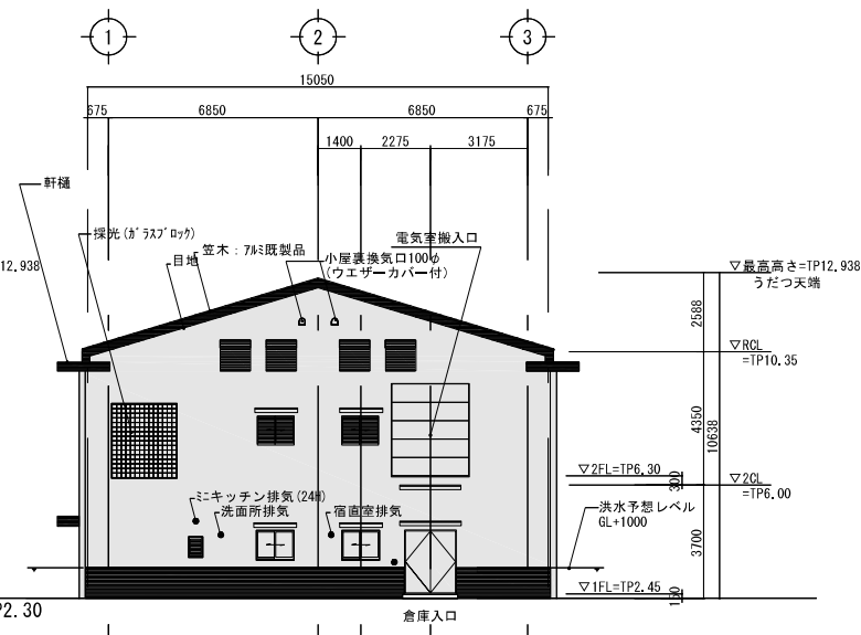
北立面図 1 / 200
