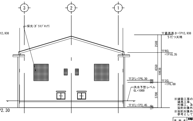
南立面図 1 / 200
