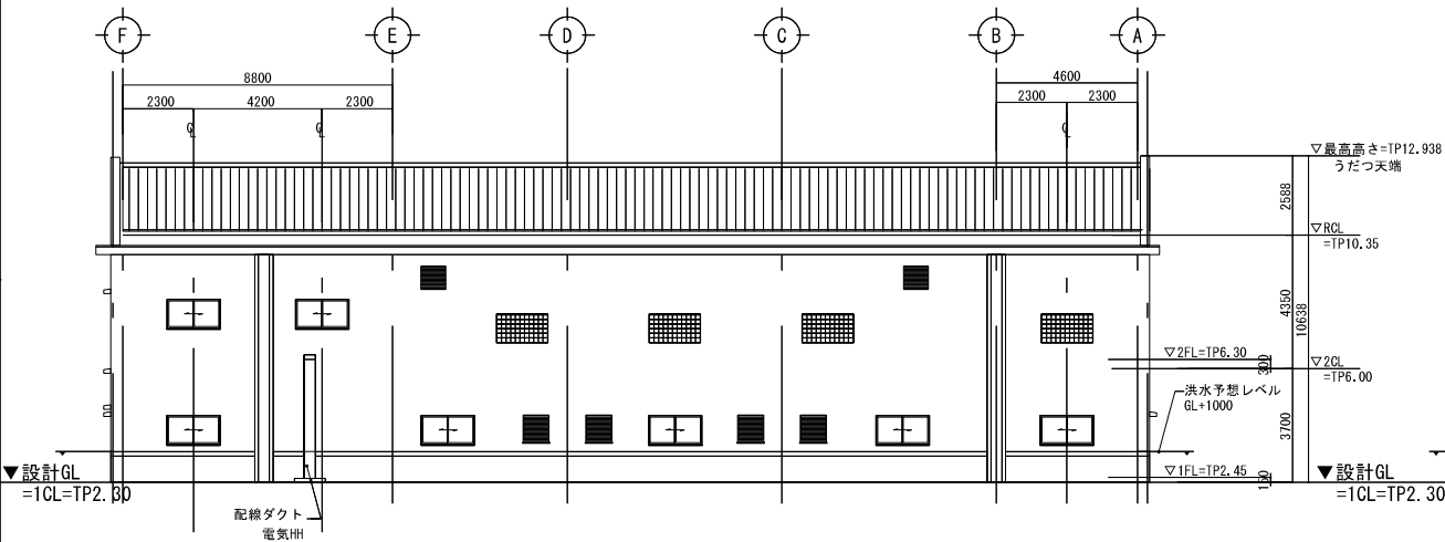
西立面図 1 / 200
