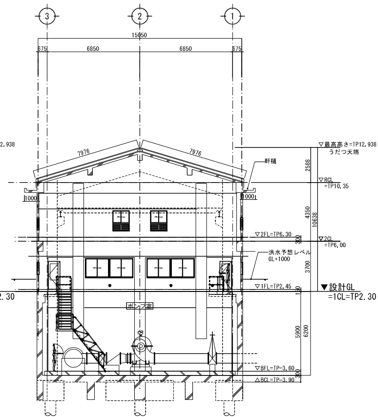
D通り断面図 1 / 200
