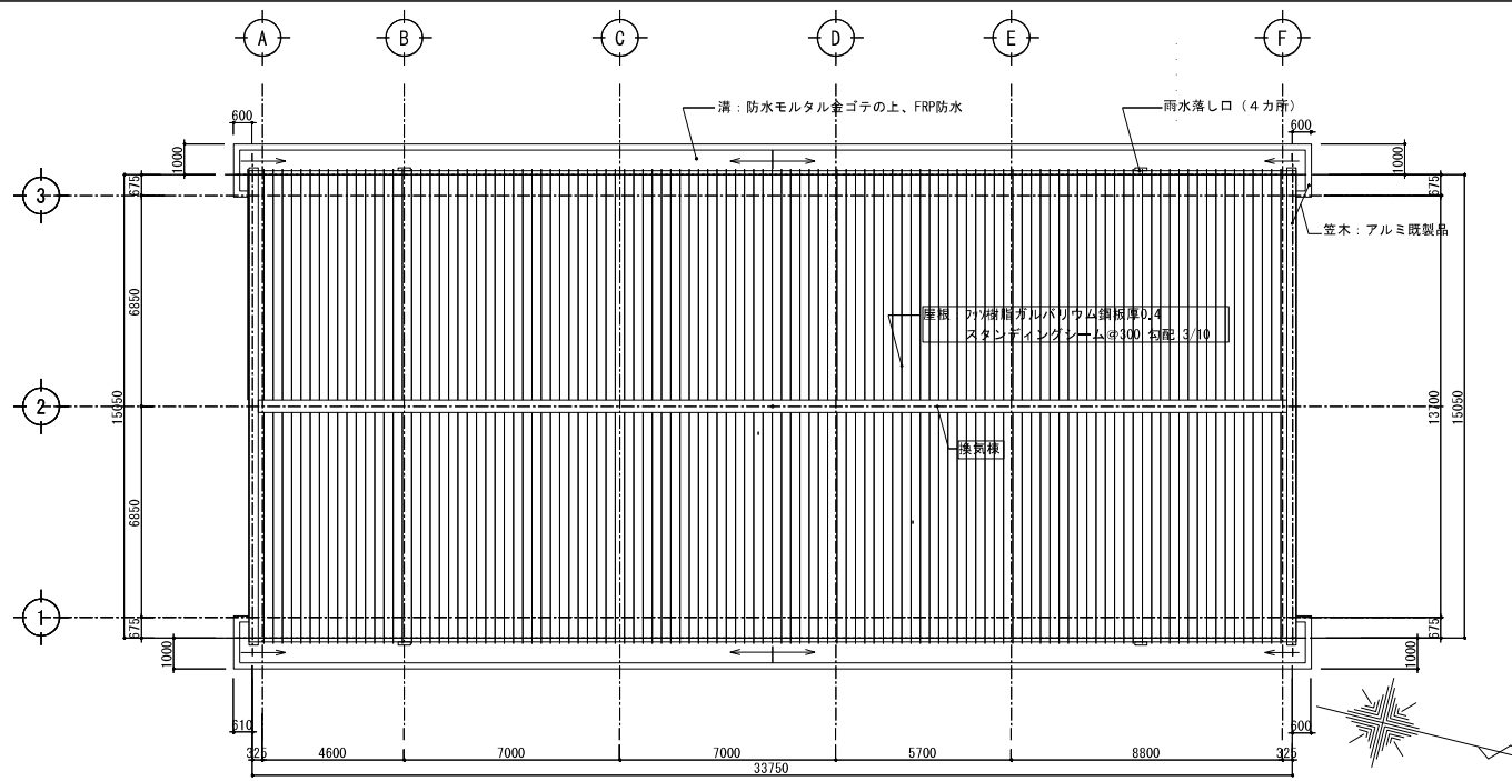
屋根伏図 1 / 200
