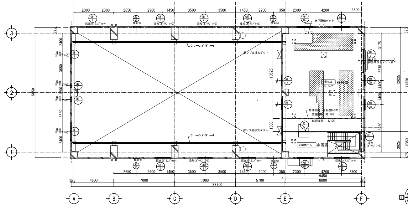
2階平面図 1 / 200
