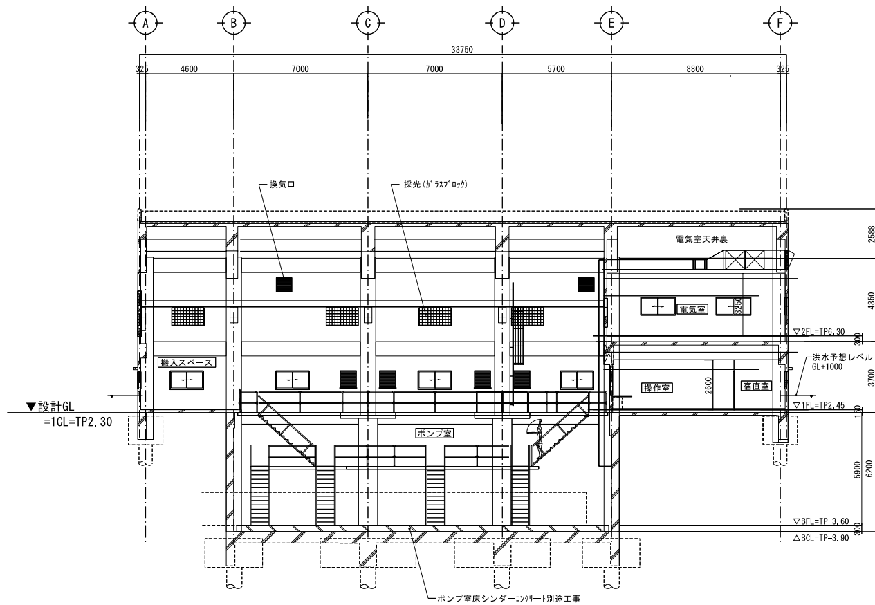
2通り断面図 1 / 200
