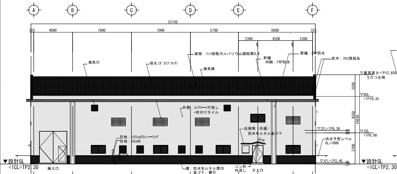
東立面図 1 / 200
