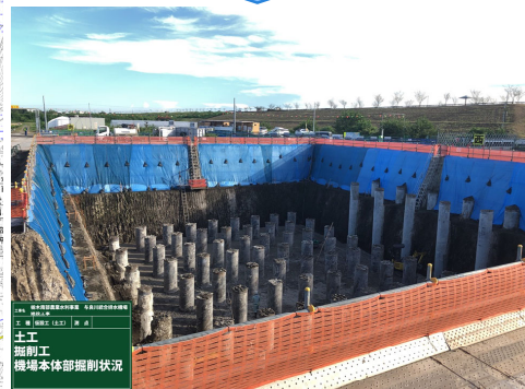
令和2年9月（機場本体部掘削）
