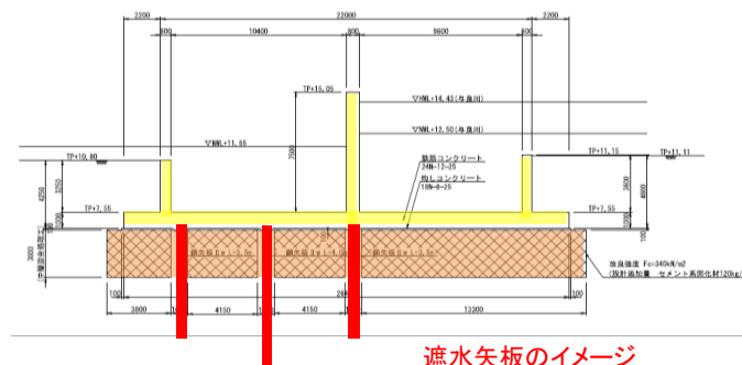
遮水矢板のイメージ
