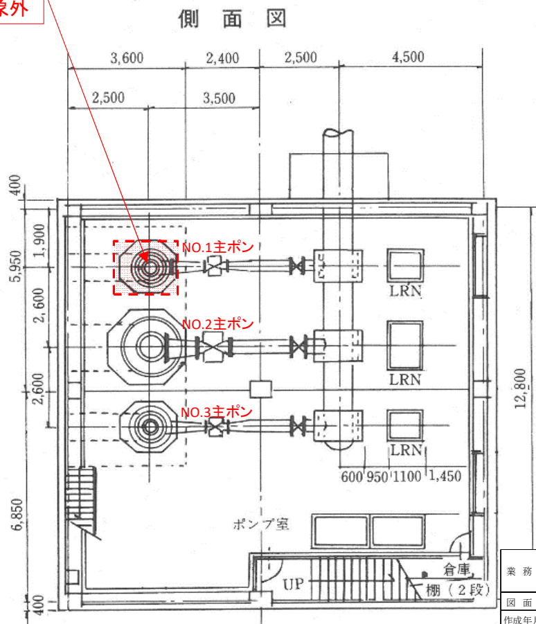
B1階平面図
