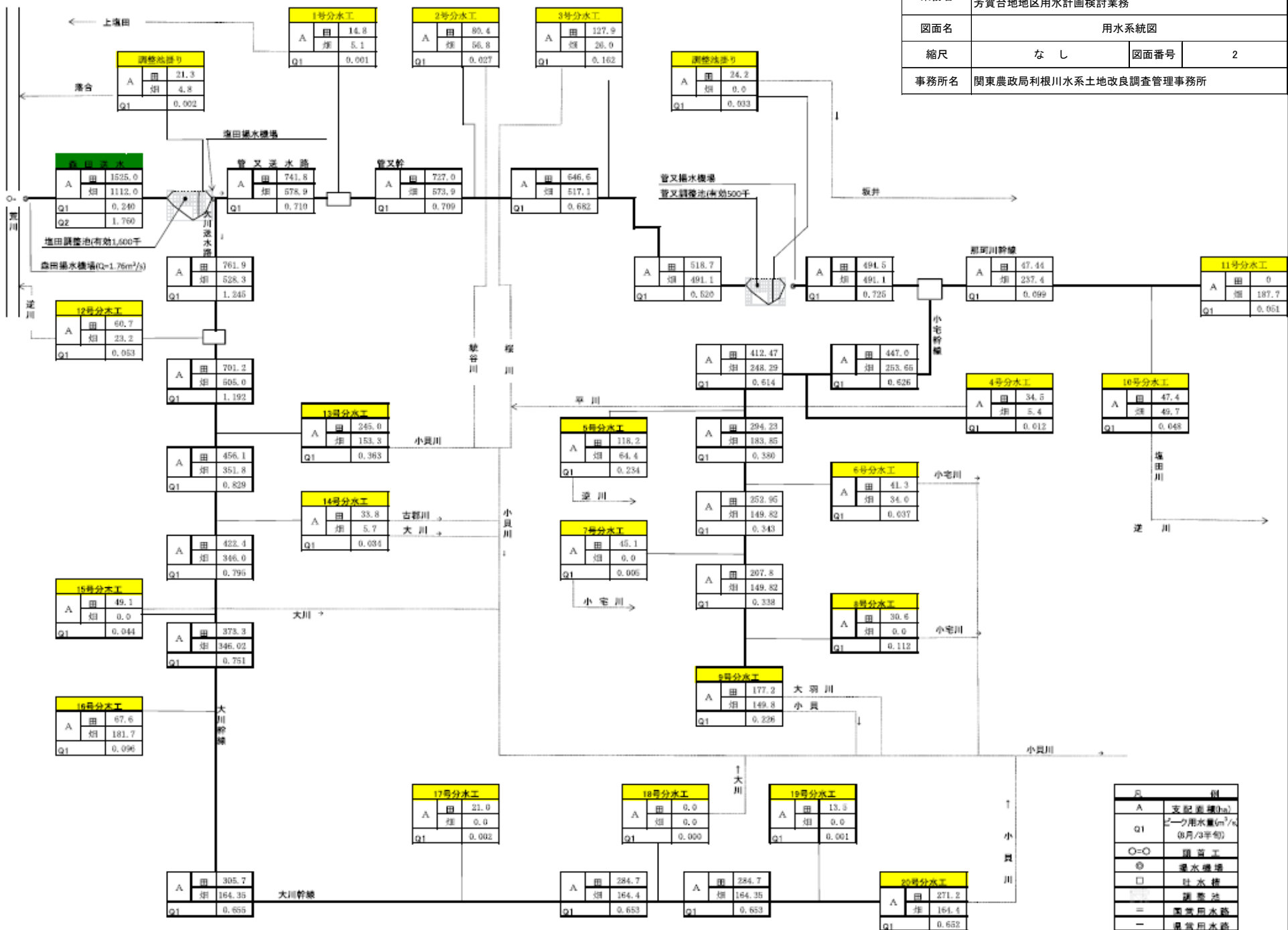
計画用水系統模式図
