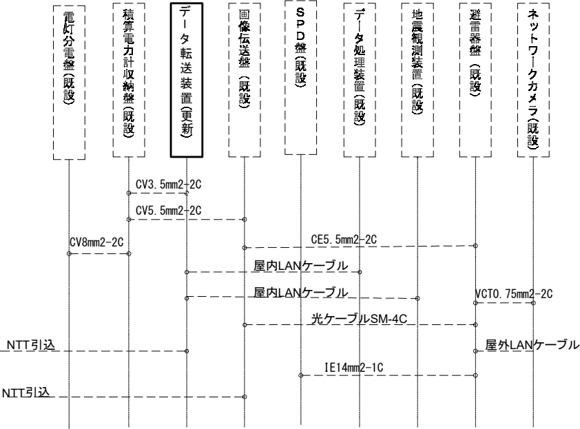
配線系統図 NON SCALE
