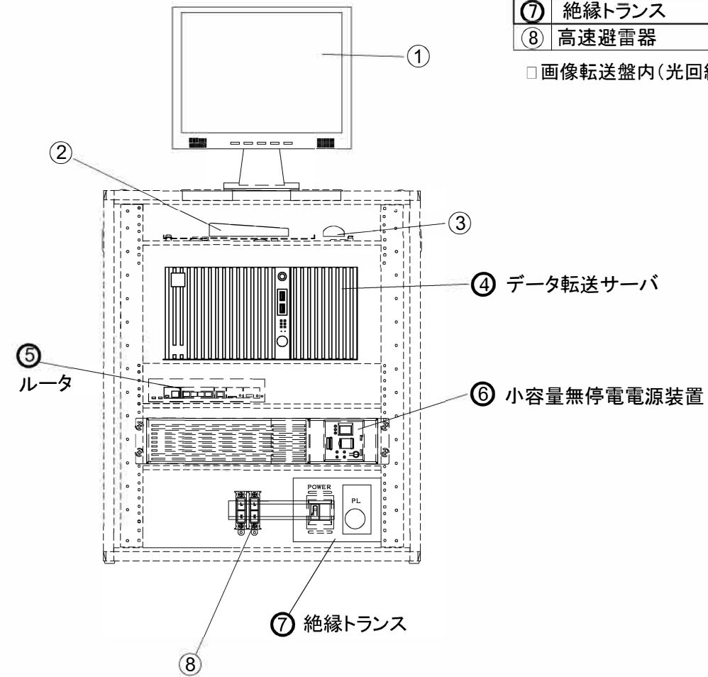
<前面内面図>
