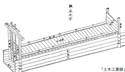
坎樋全体図（関東流）
