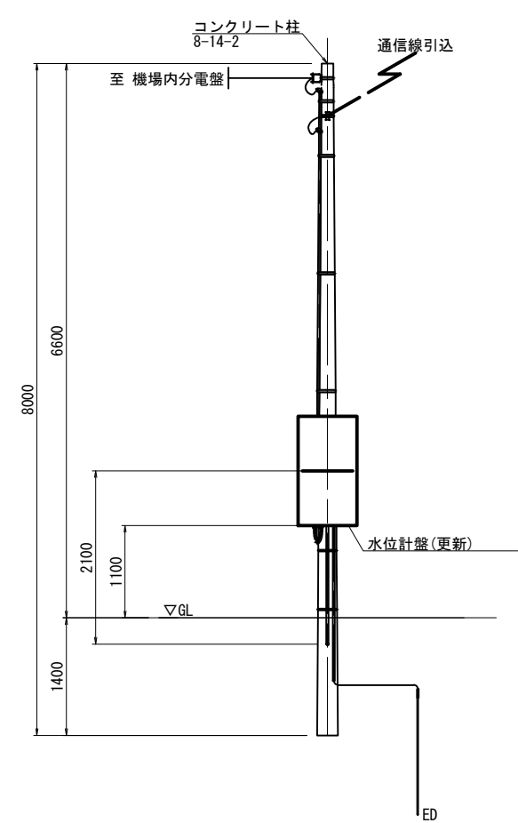
配線系統図
