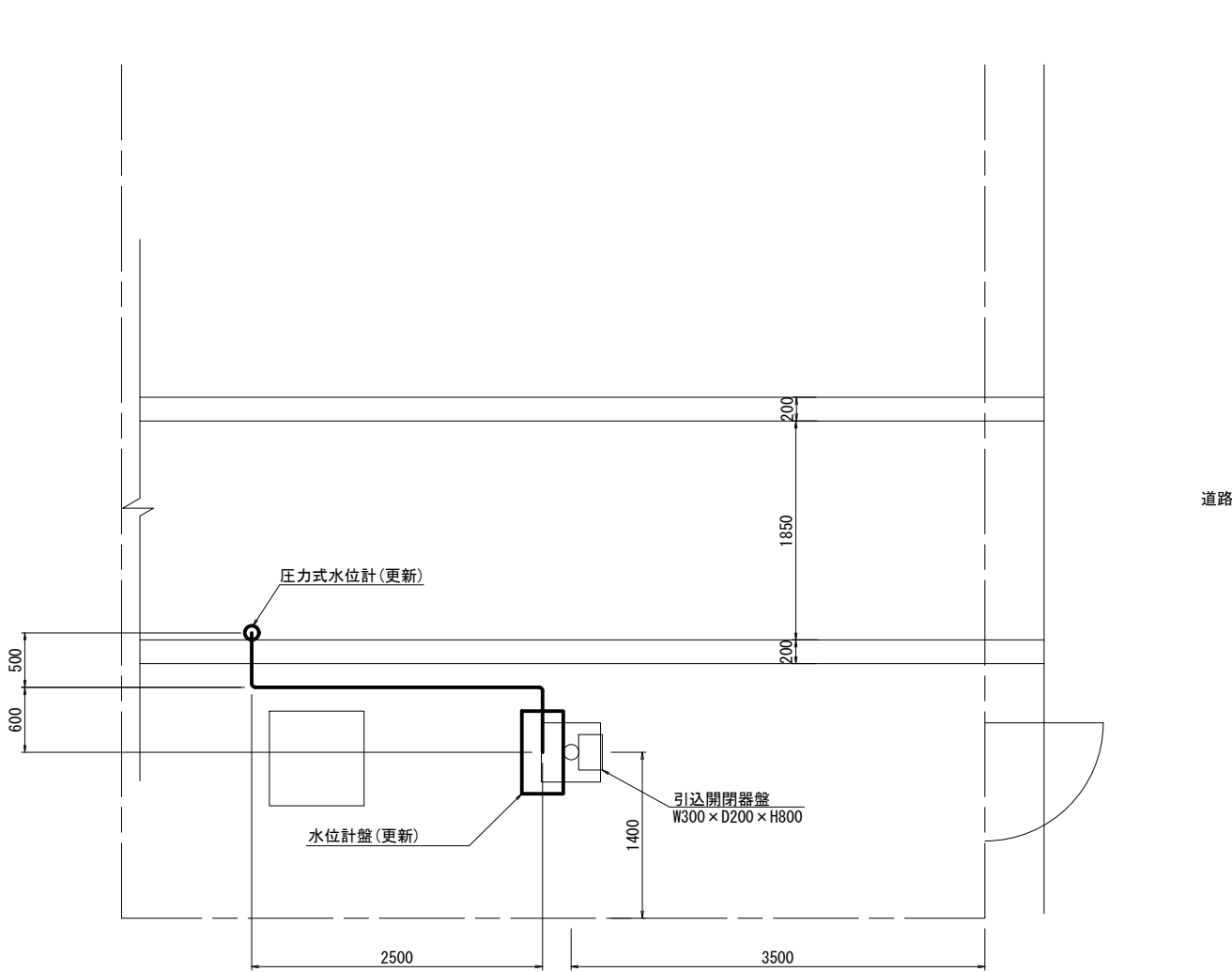
平面図
