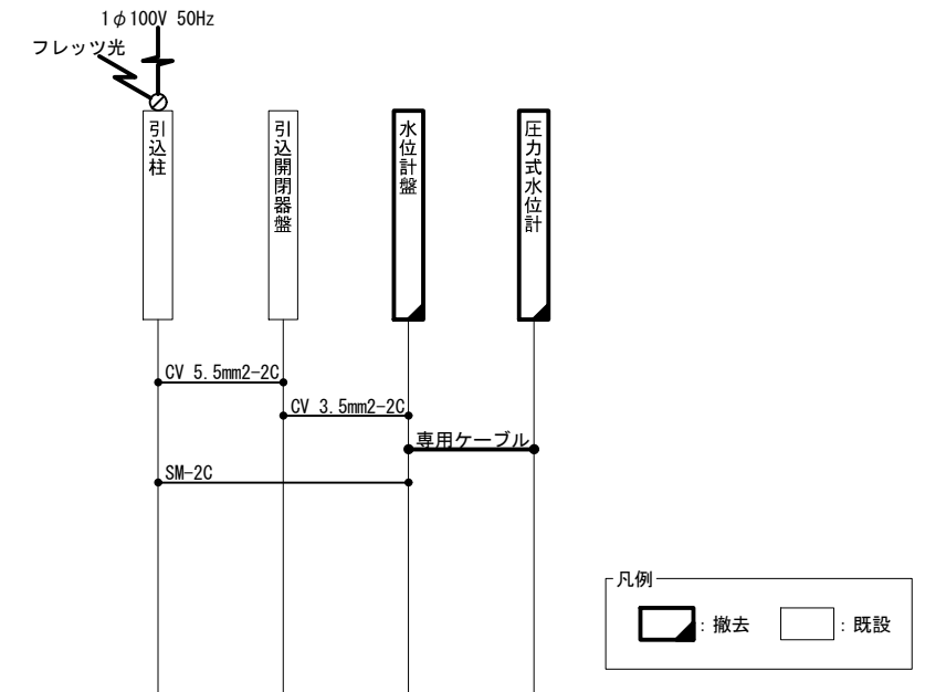
配線系統図
