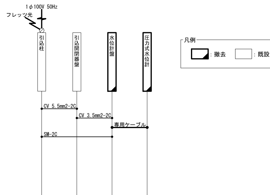
配線系統図
