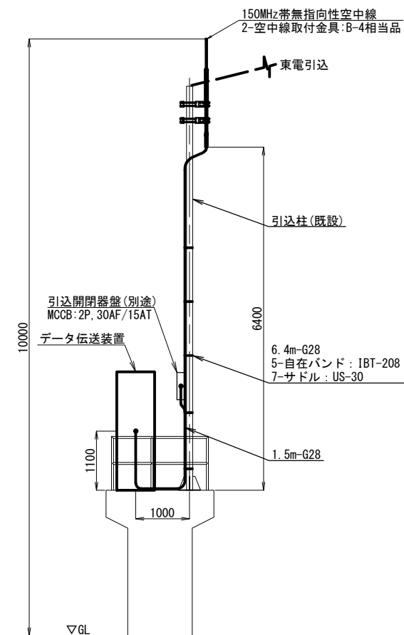
引込柱装柱図
