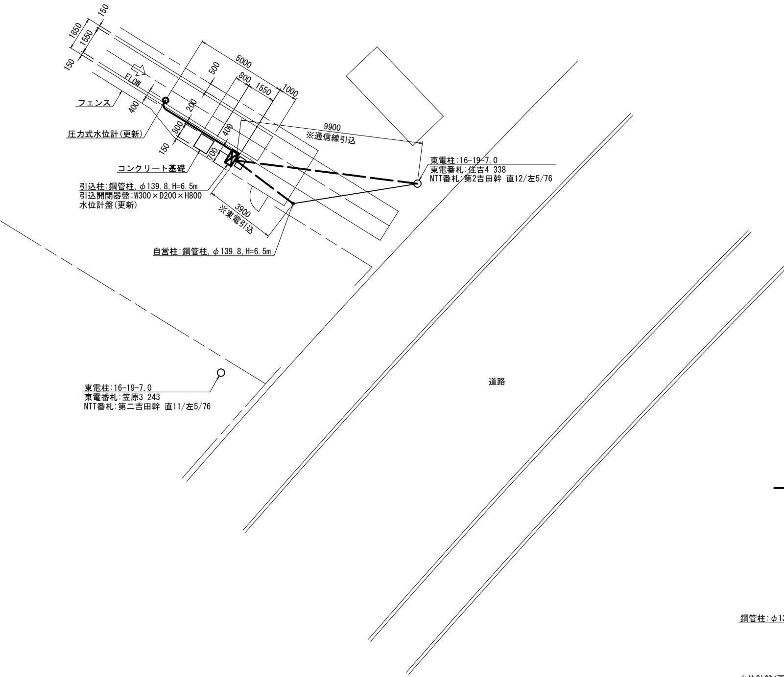
平面図
