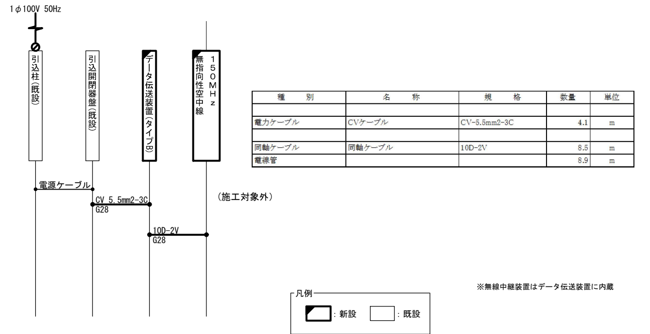
配線系統図
