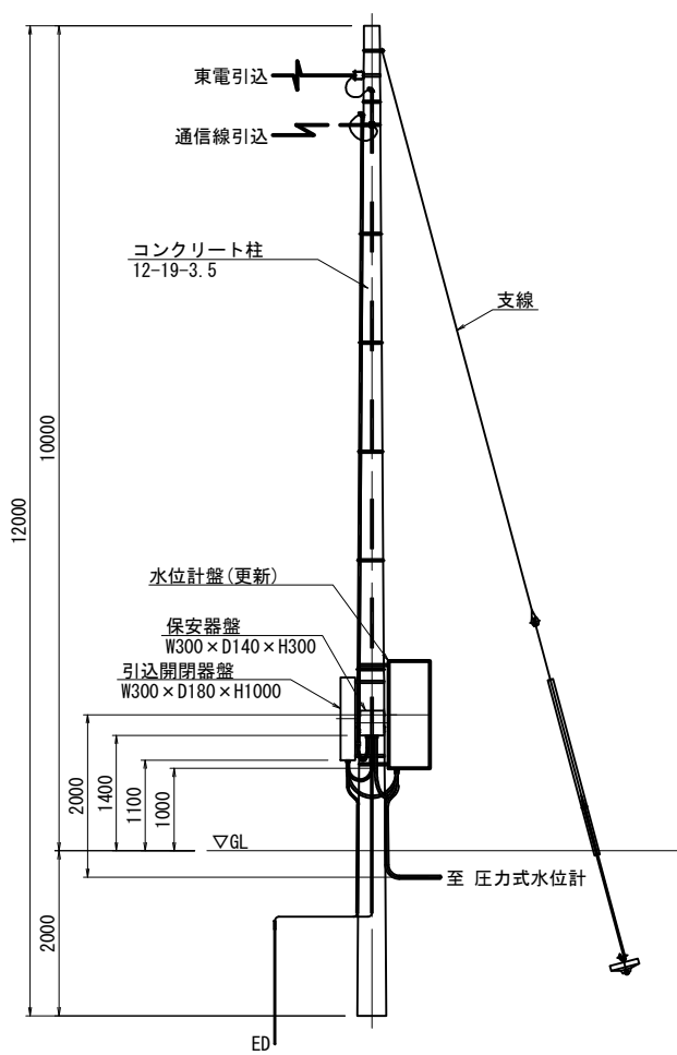
引込柱装柱図
