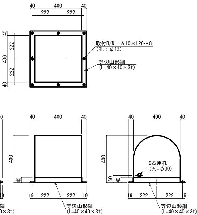
水位計箱詳細図
