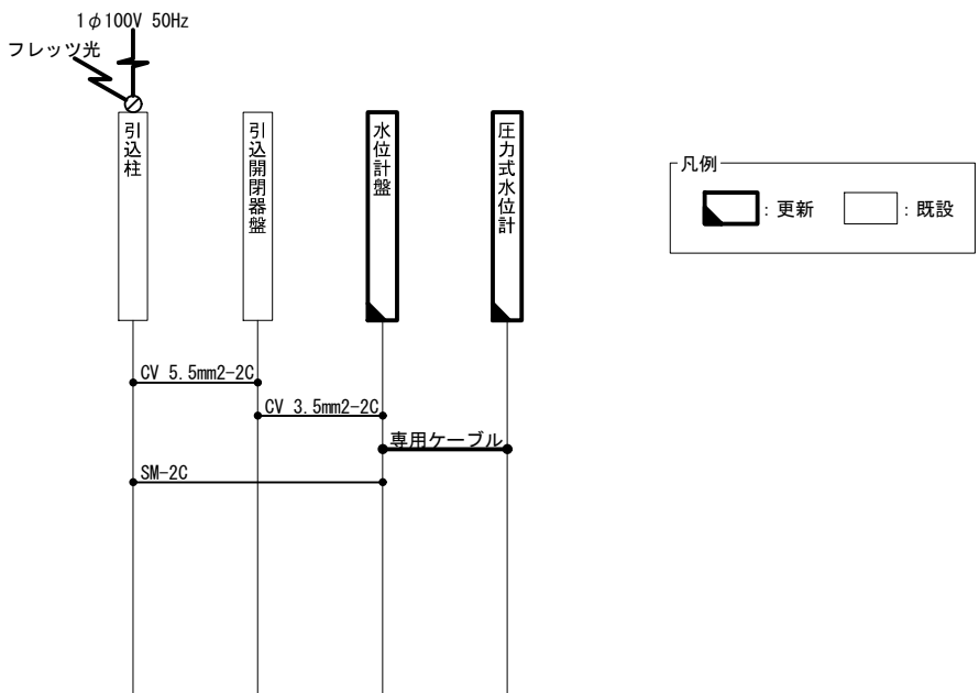
配線系統図
