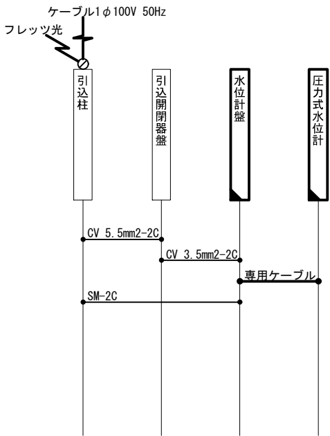
配線系統図
