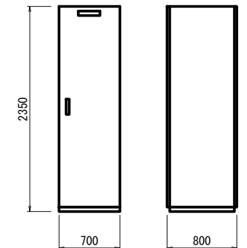
屋内自立型
