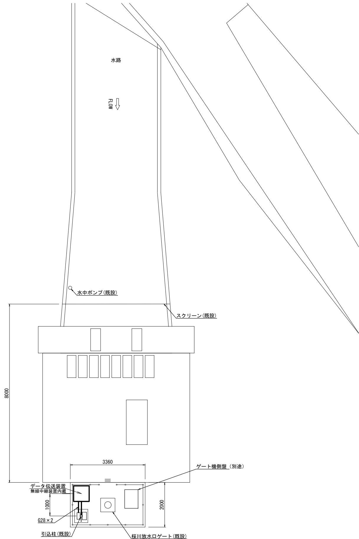
平面図
