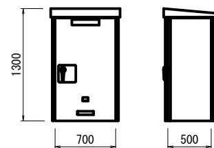
屋外装柱型
