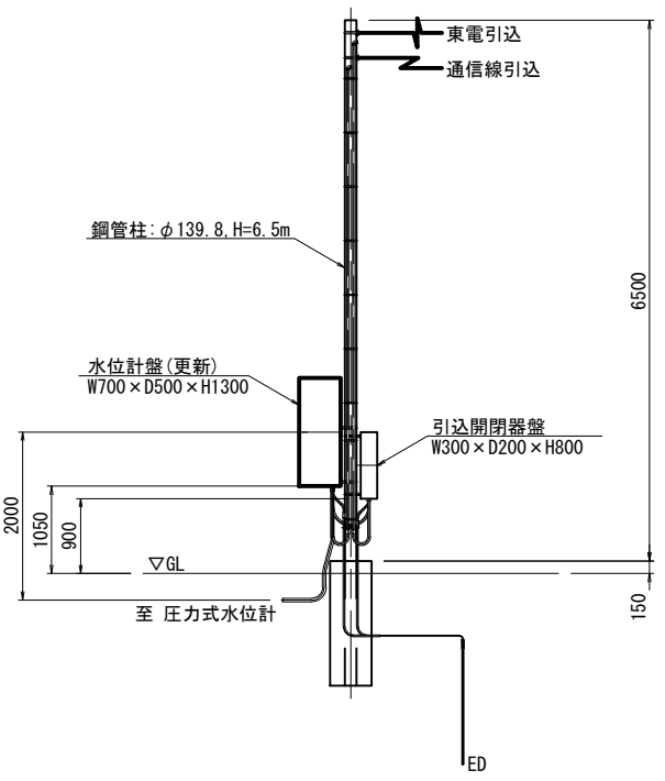
引込柱装柱図
