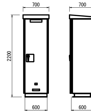
屋外自立型
