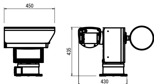
カメラ装置 ※
