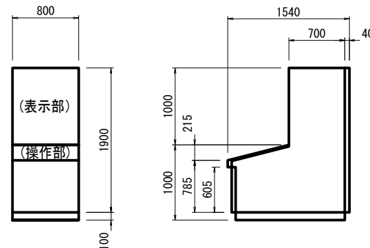
監視操作机(備前堀) ※
