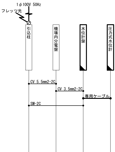
配線系統図
