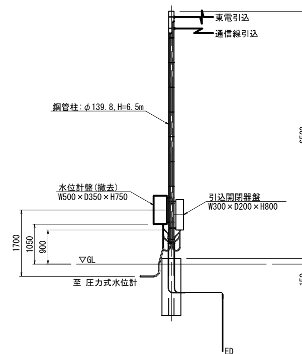
引入柱装柱图
