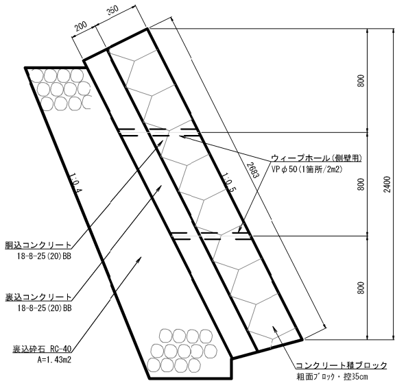
コンクリートブロック積工詳細図
