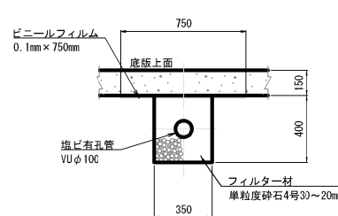
アンダードレーン詳細図
