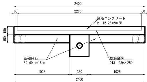
底板コンクリート詳細図
