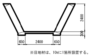
張コンクリート詳細図
