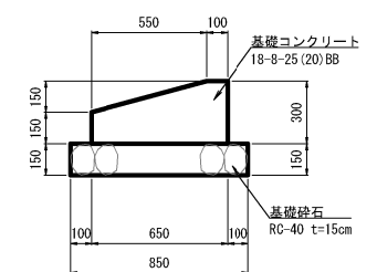
基礎コンクリート詳細図
