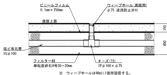
アンダードレーン詳細図
