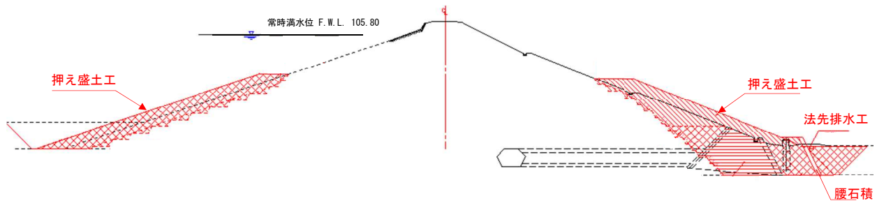
図2 施設の断面図（改修）
