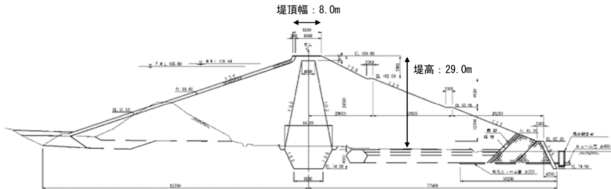
図1 施設の現況断面図
