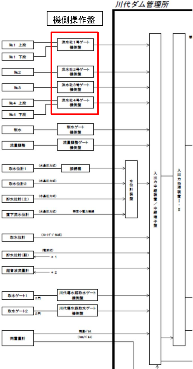
【システム図】
