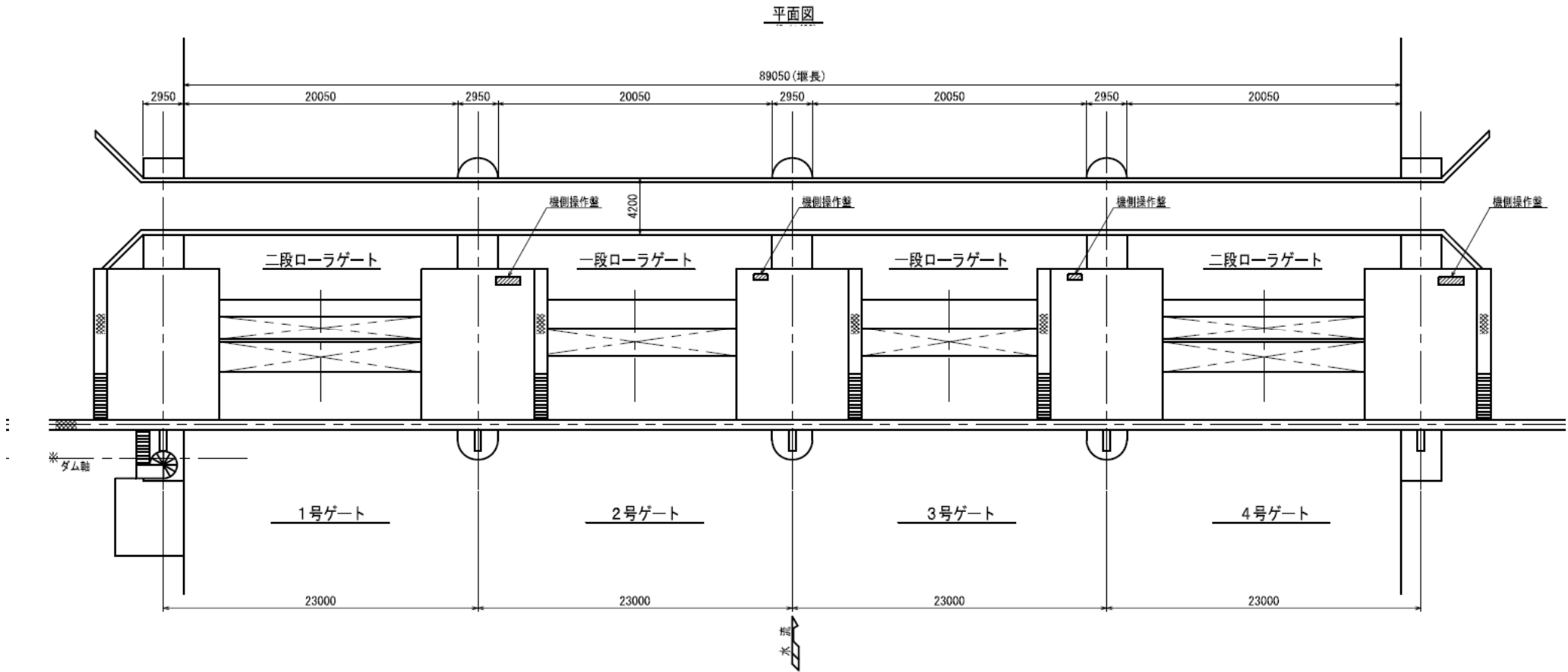
洪水吐設備構造図 (洪水吐設備全体)
