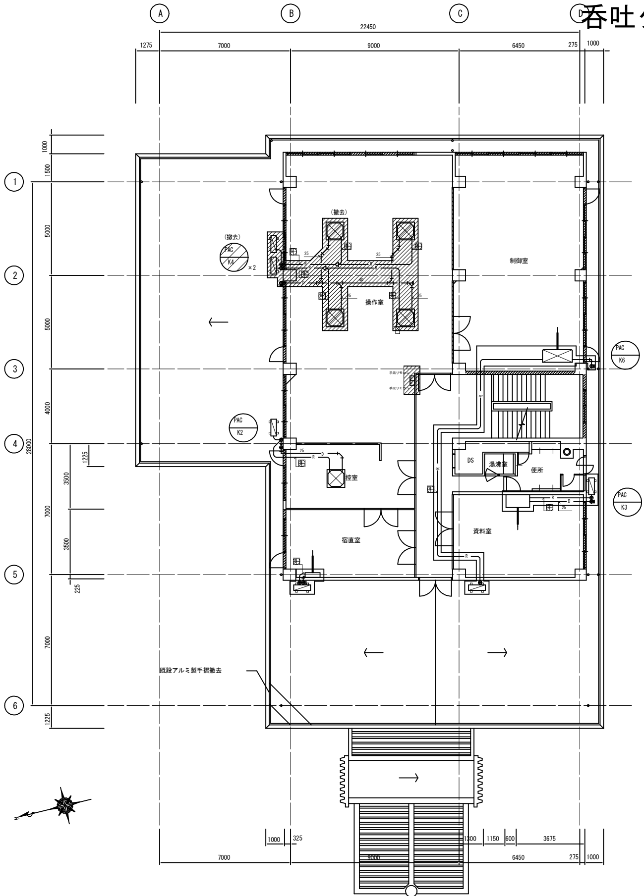
2階平面図 1:100
