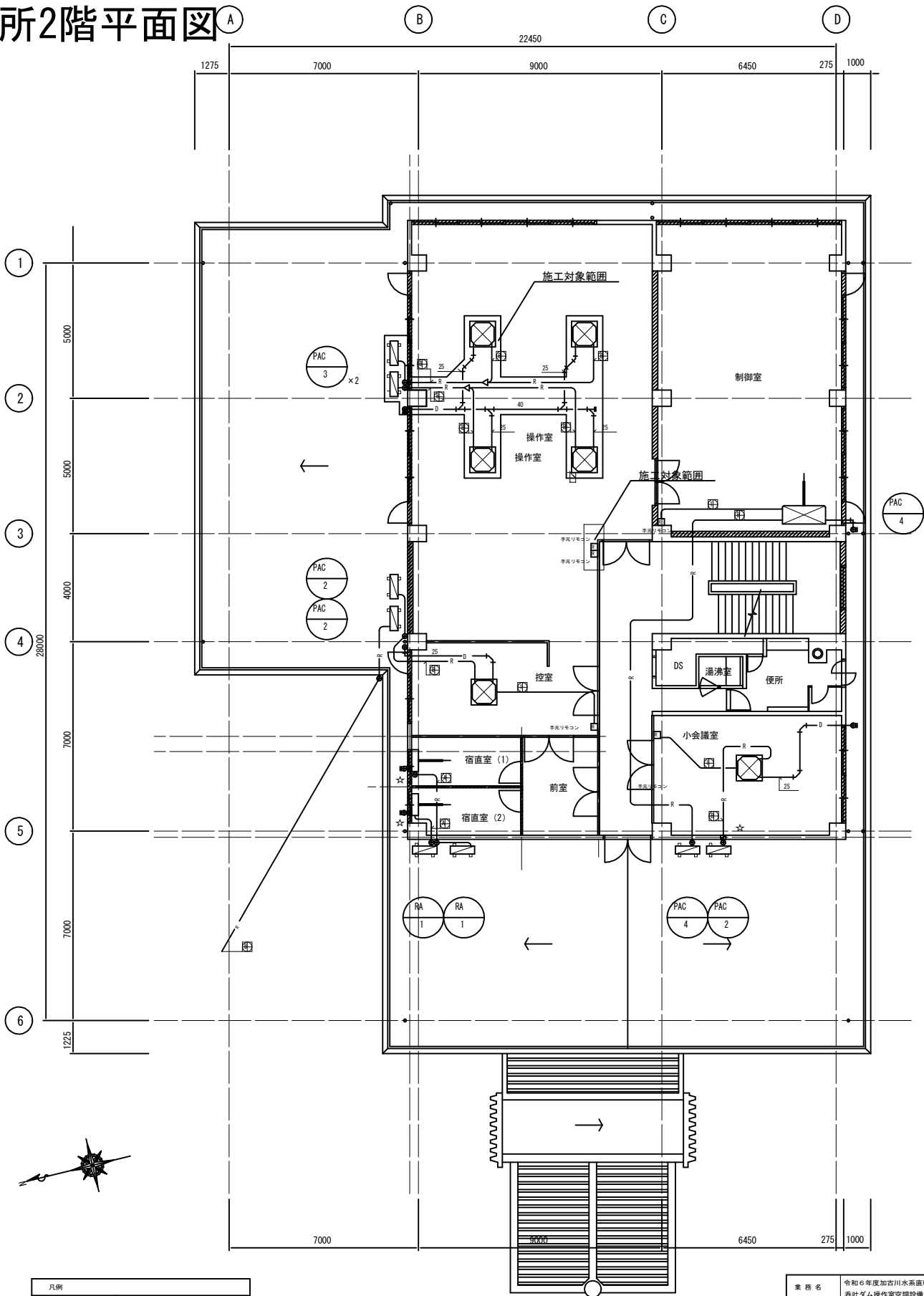
2階平面図 1:100
