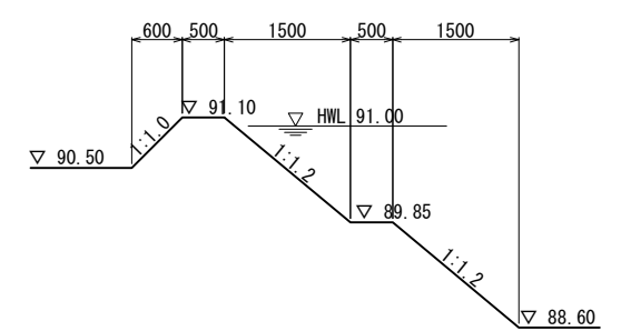
D-D断面图 S=1:50
