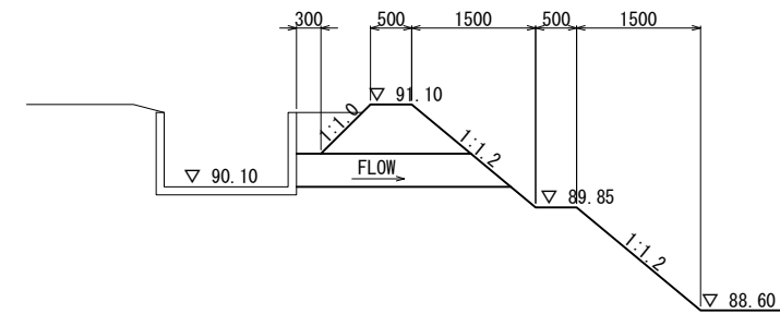
C-C断面图 S=1:50
