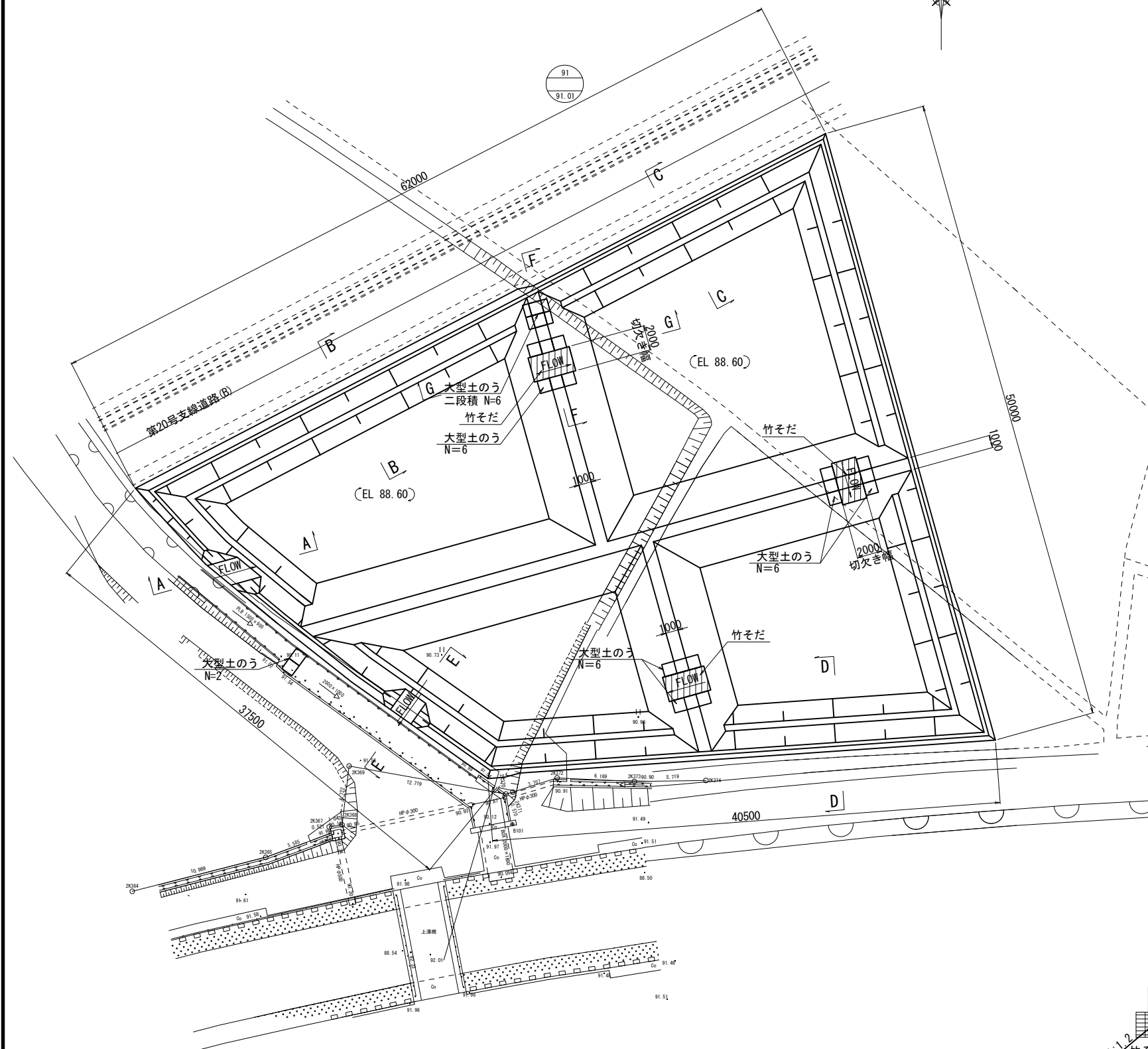
平面图 S=1:200
