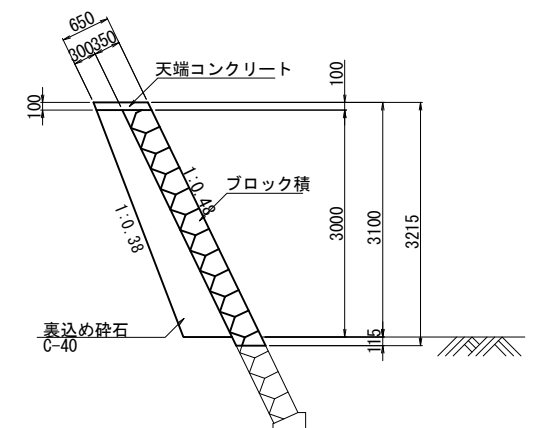
ブロック積護岸
