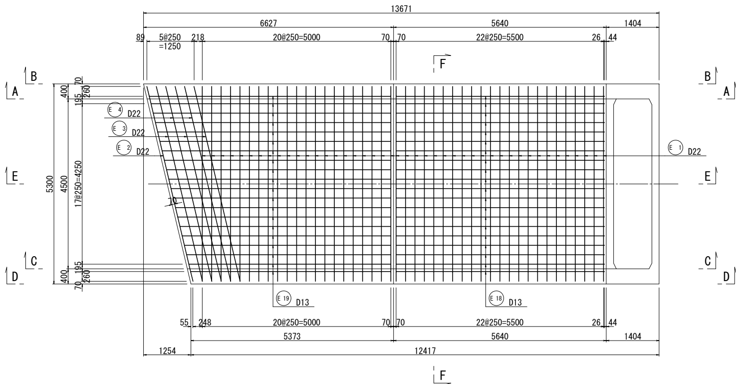
頂版下面
