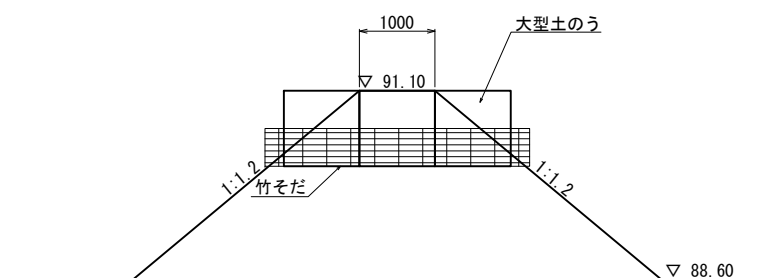
G-G断面图 S=1:50
