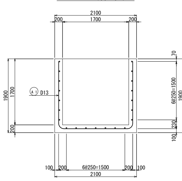
E - E断面図
