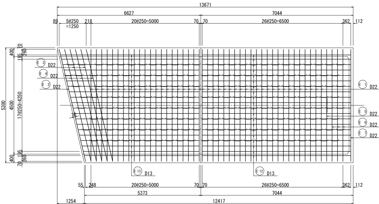
底版下面
