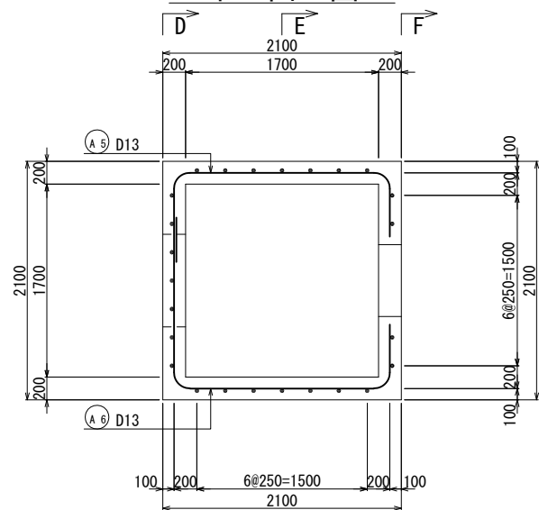
平面図
