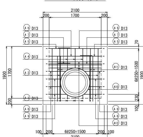
D - D断面図
