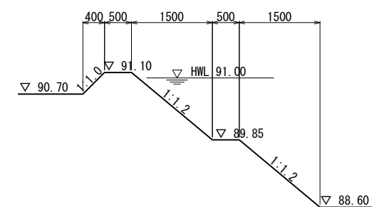
D-D断面图 S=1:50
