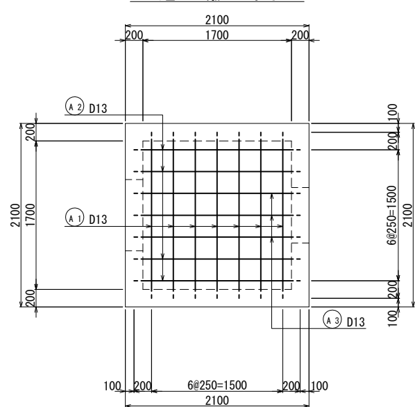
底版図
