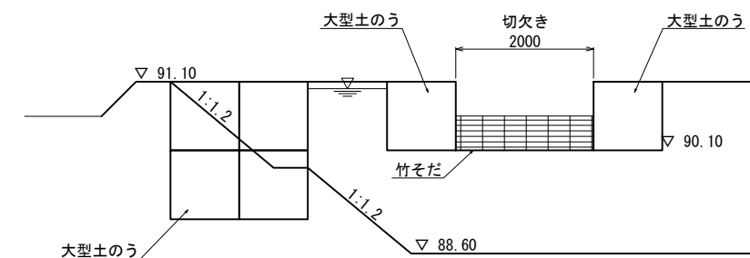
F-F断面图 S=1:50
