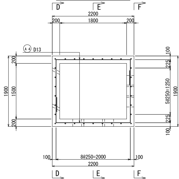
底版配筋図
