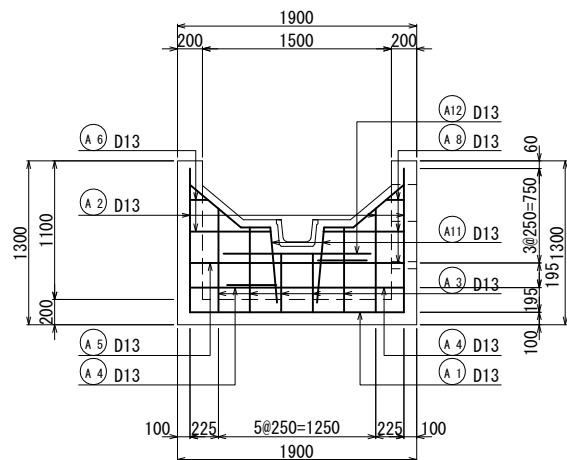
F - F断面図
