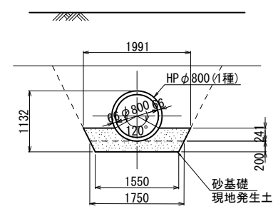
横 断 図
