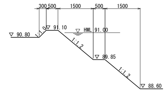
E-E断面图 S=1:50
