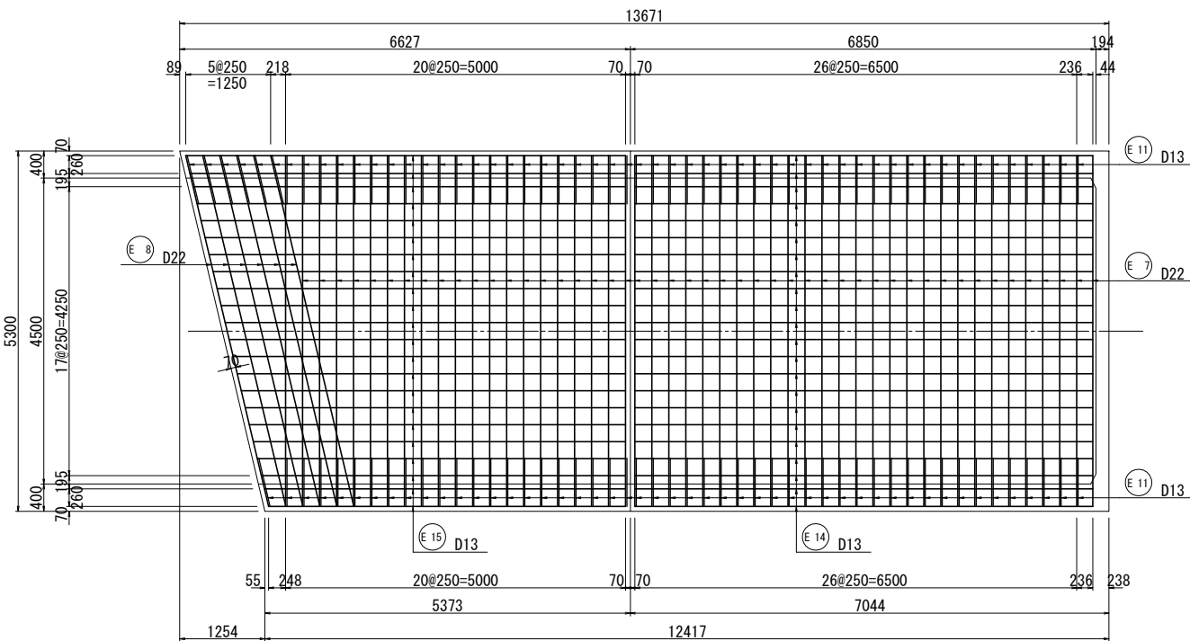
底版上面
