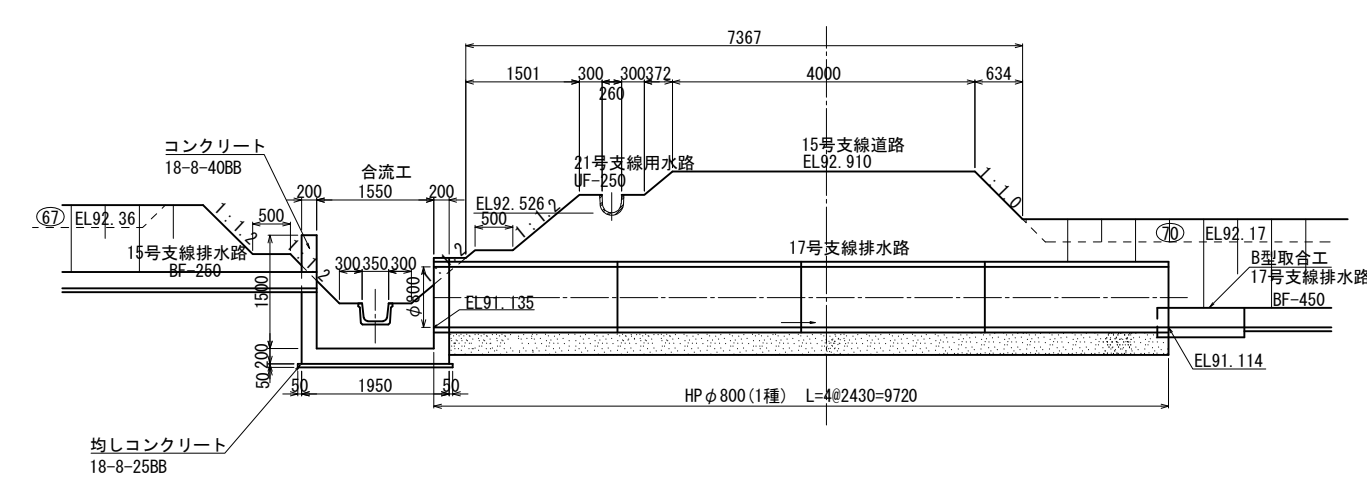
縦 断 図
