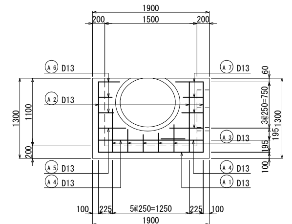
D - D断面図
