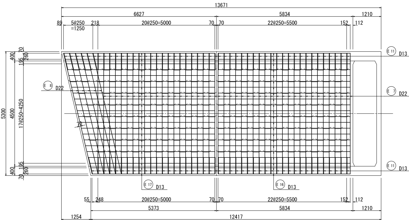
頂版下面
