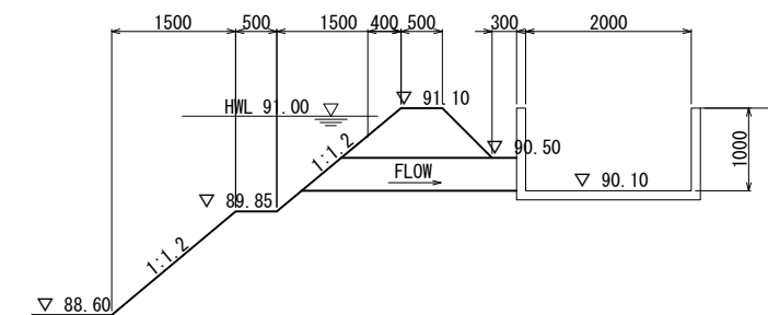
F-F断面图 S=1:50
