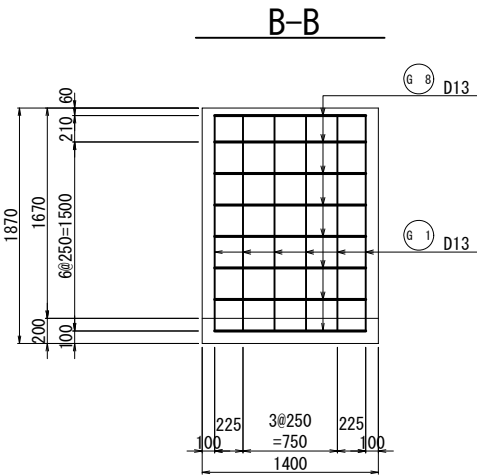
分土工配筋図
