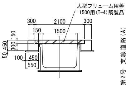
進入路蓋部詳細図
