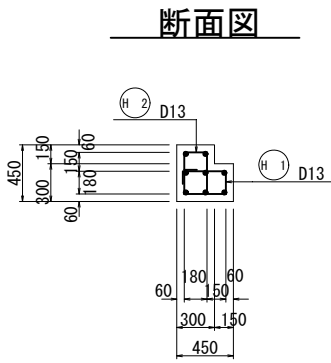
進入路工蓋受梁配筋図
