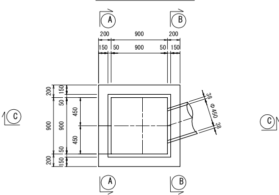
平面図
