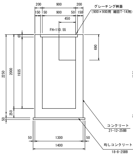
A-A 断面図
