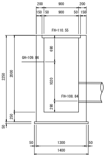
C-C 断面図
