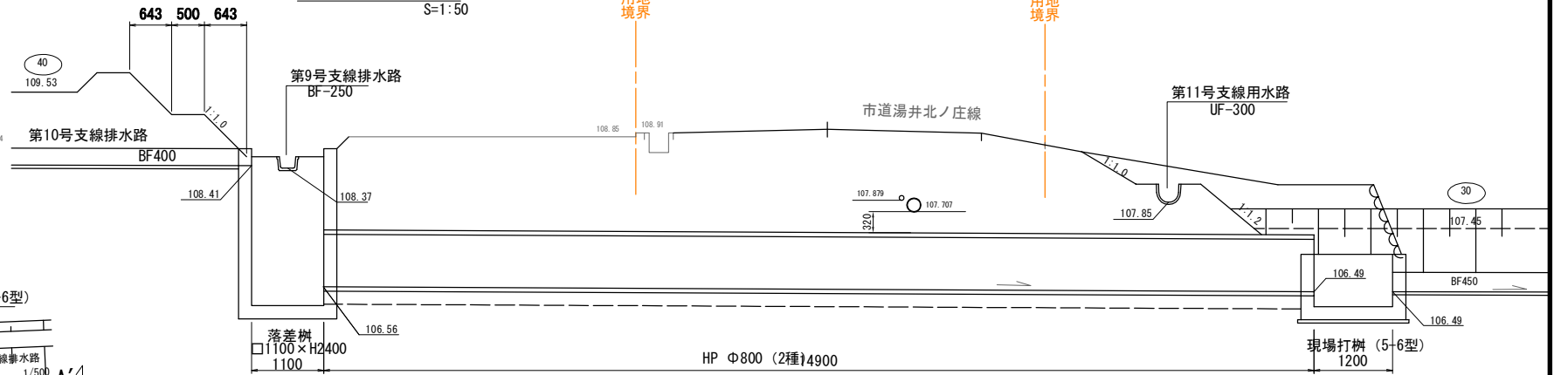
A-A' 断面図
