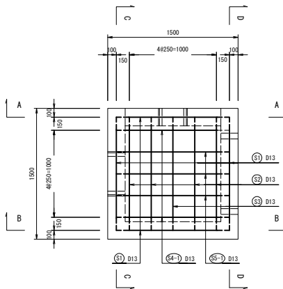
平面図(底板)
