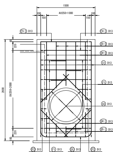
D-D断面図
