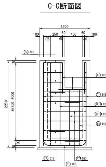
接続桷配筋図
