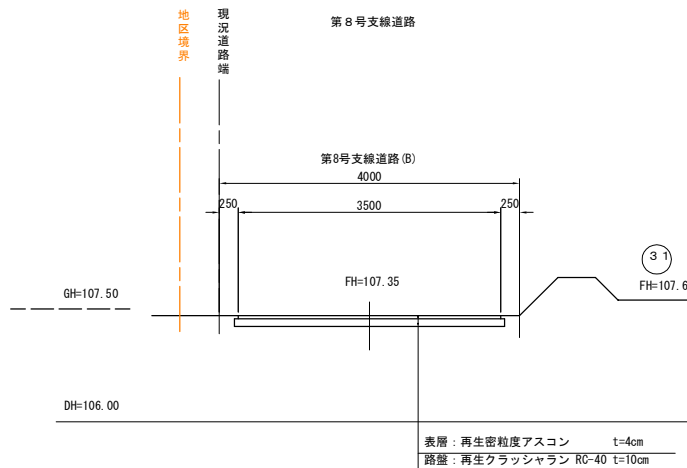
横断面図
