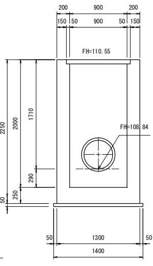
B-B 断面図
