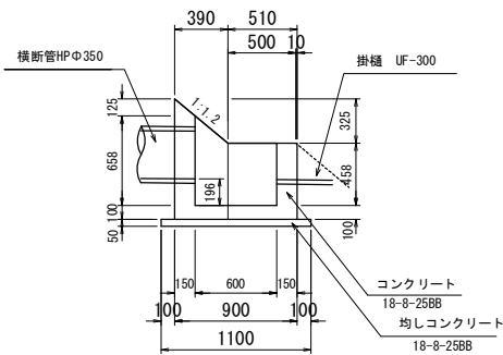
縦断面図
