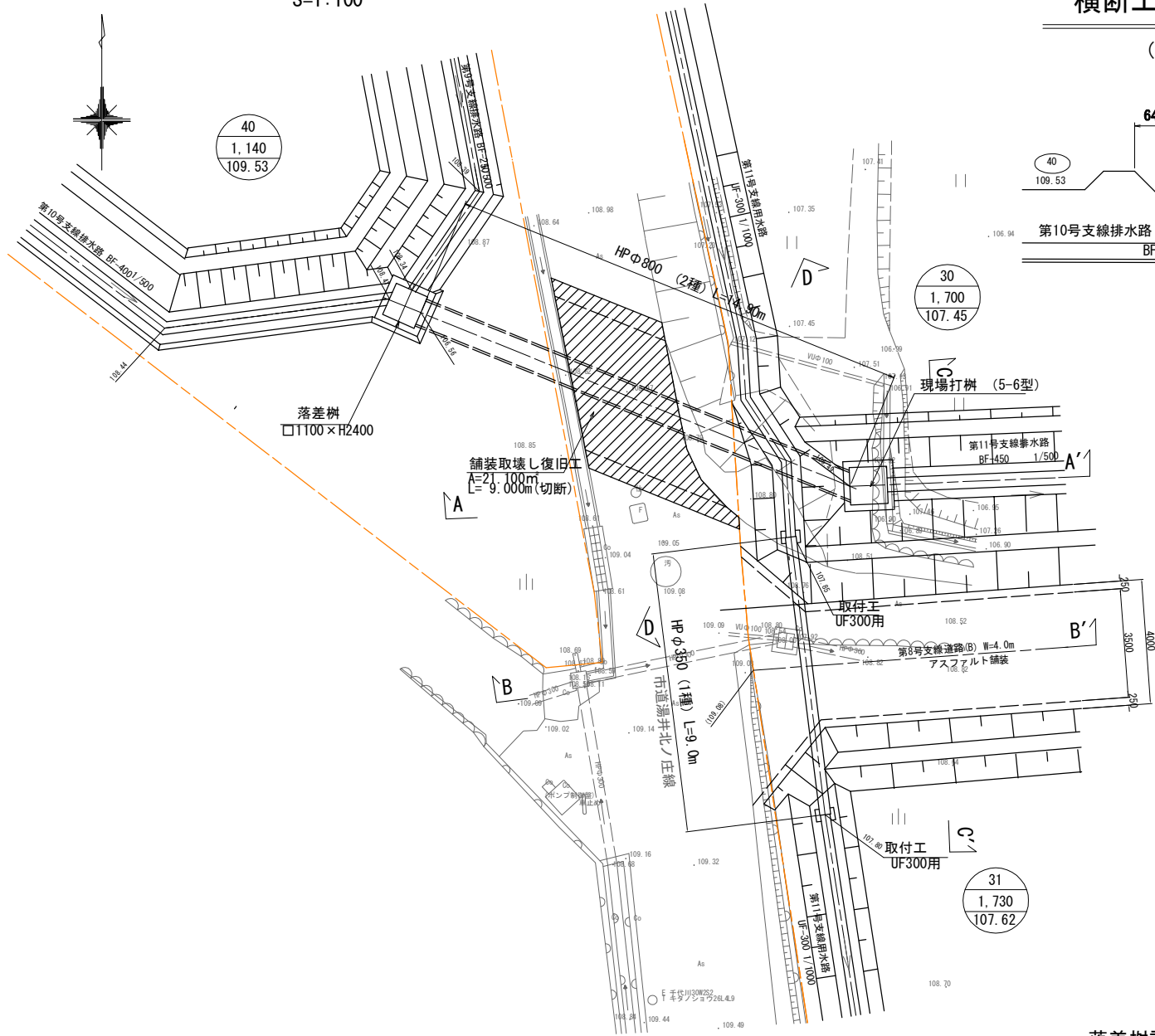
落差樹詳細図
