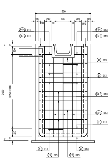
C-C断面図
