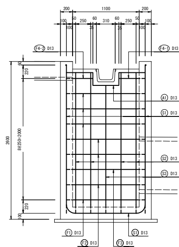
A-A断面図
