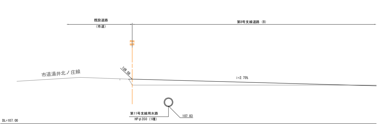
道路横断管標準図
