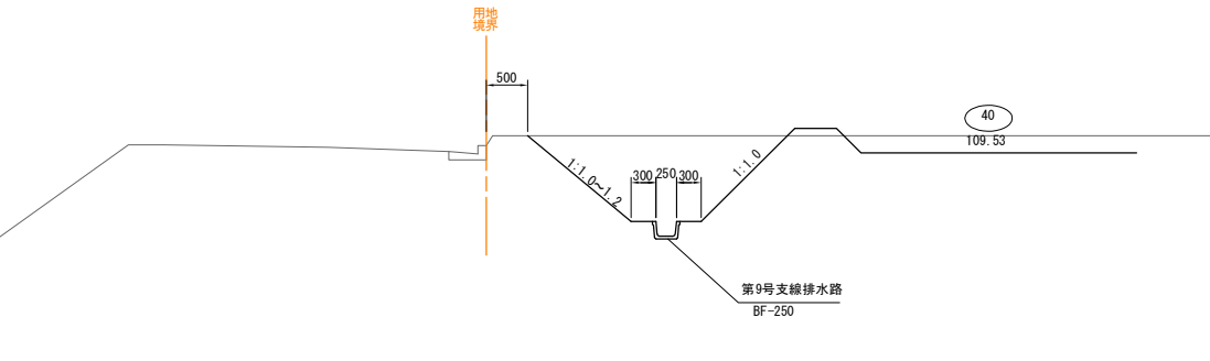
道路横断管標準図
