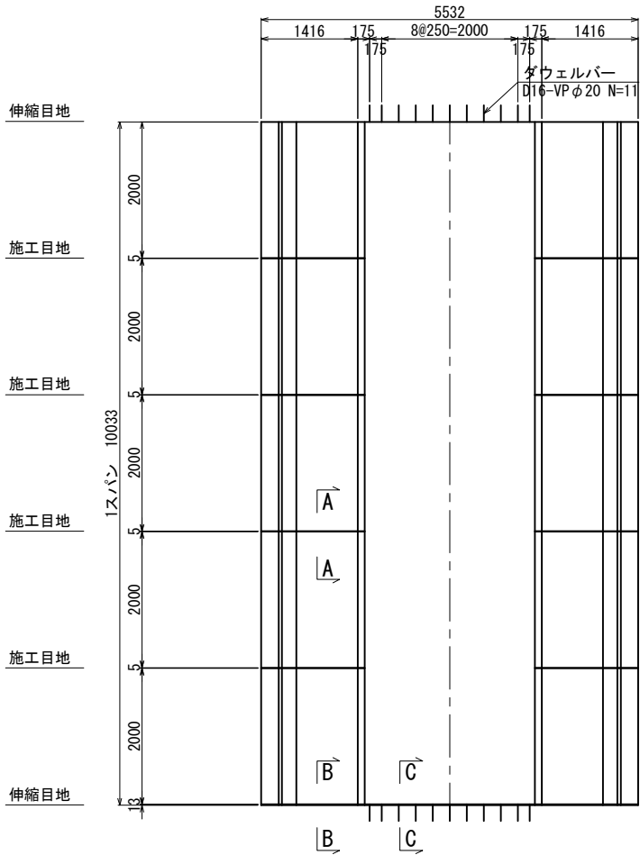
平面図
