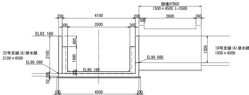
B - B断面図
