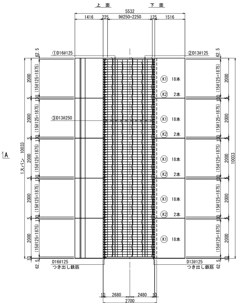
平面図
