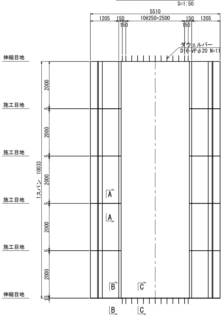
平面図
