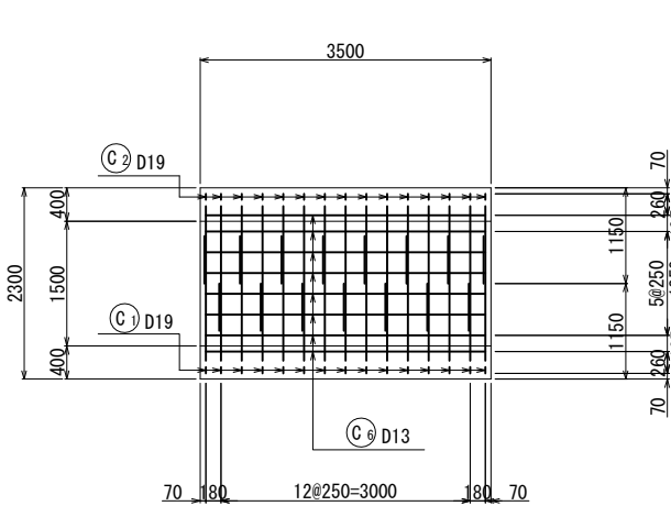
A - A外面図
