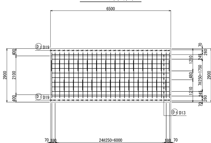
D - D断面図
