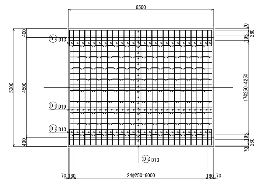
底版上面図
