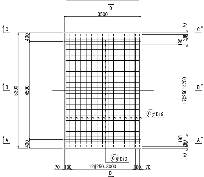
頂版下面図
