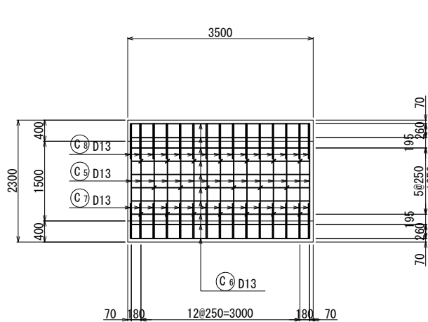
A - A内面図
