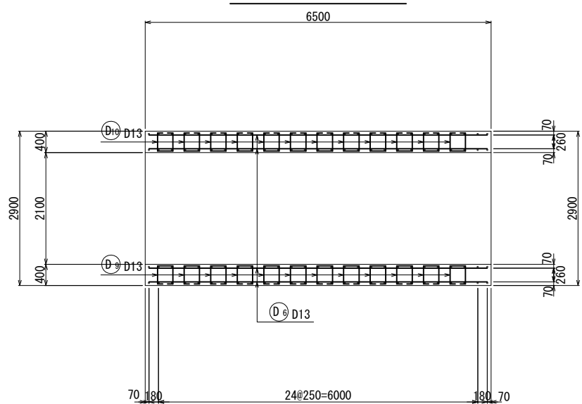
C - C外面図
