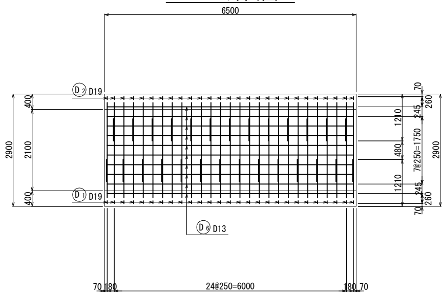
A - A内面図
