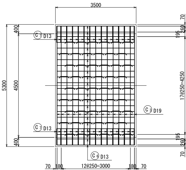
底板上面図
