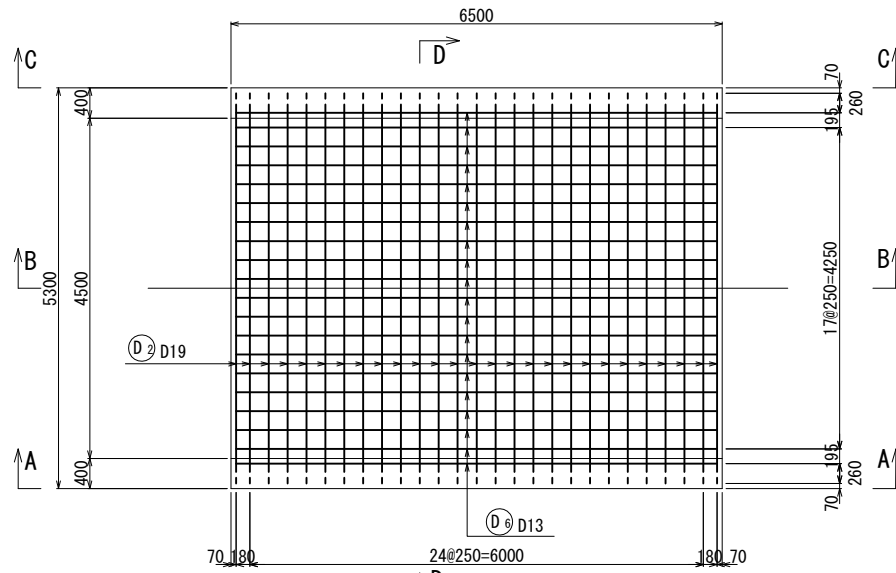
頂版下面図
