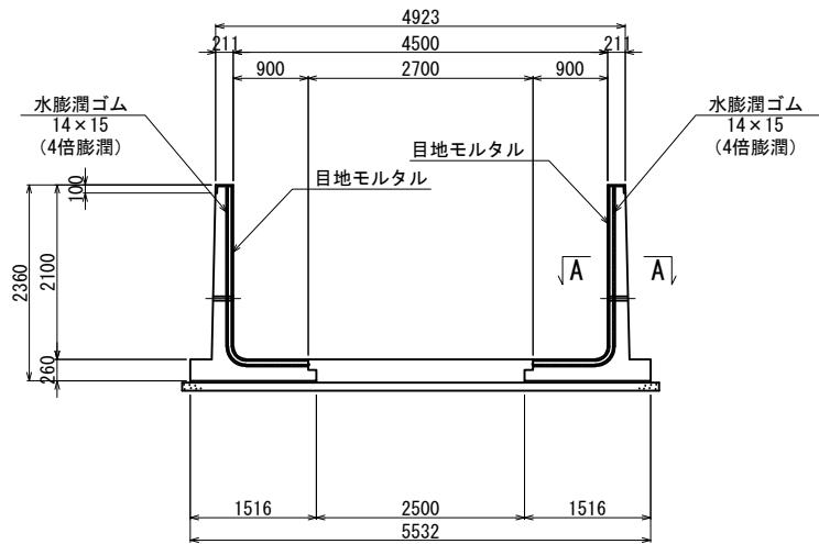
施工目地部断面図
