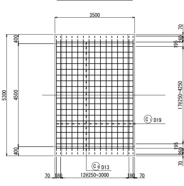
A - A外面図
