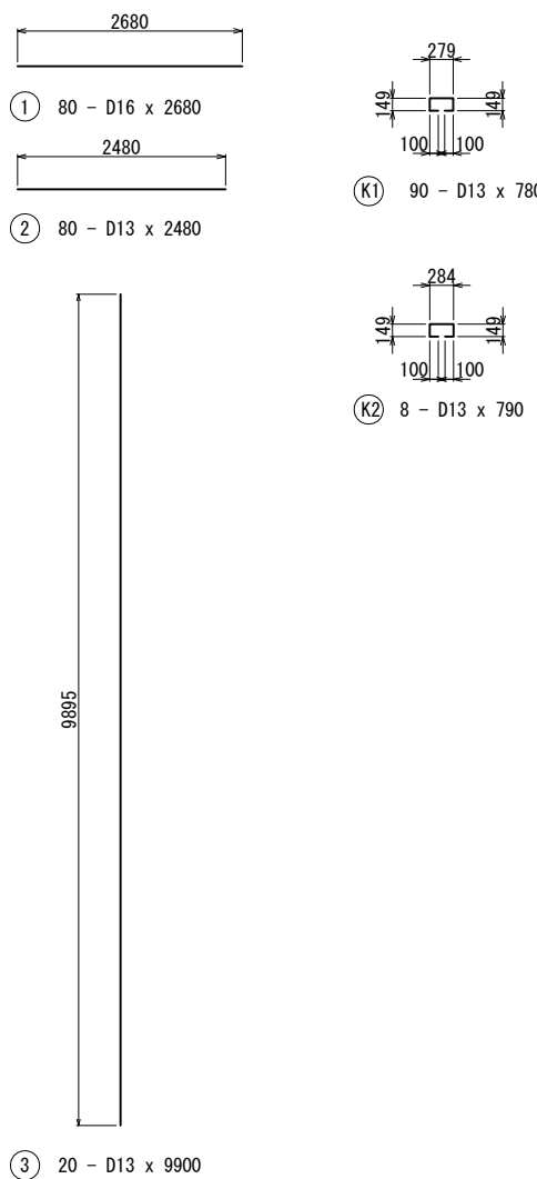
(参考) 鉄筋加工図
