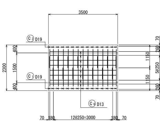
C - C外面図
