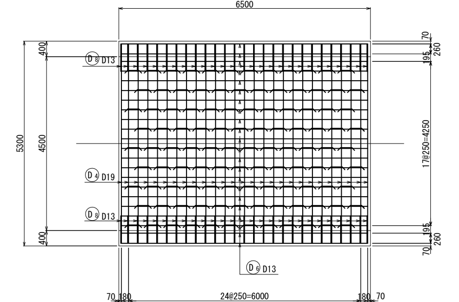
底版上面図
