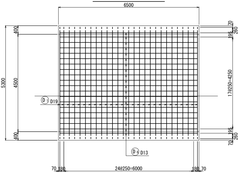
A - A外面図
