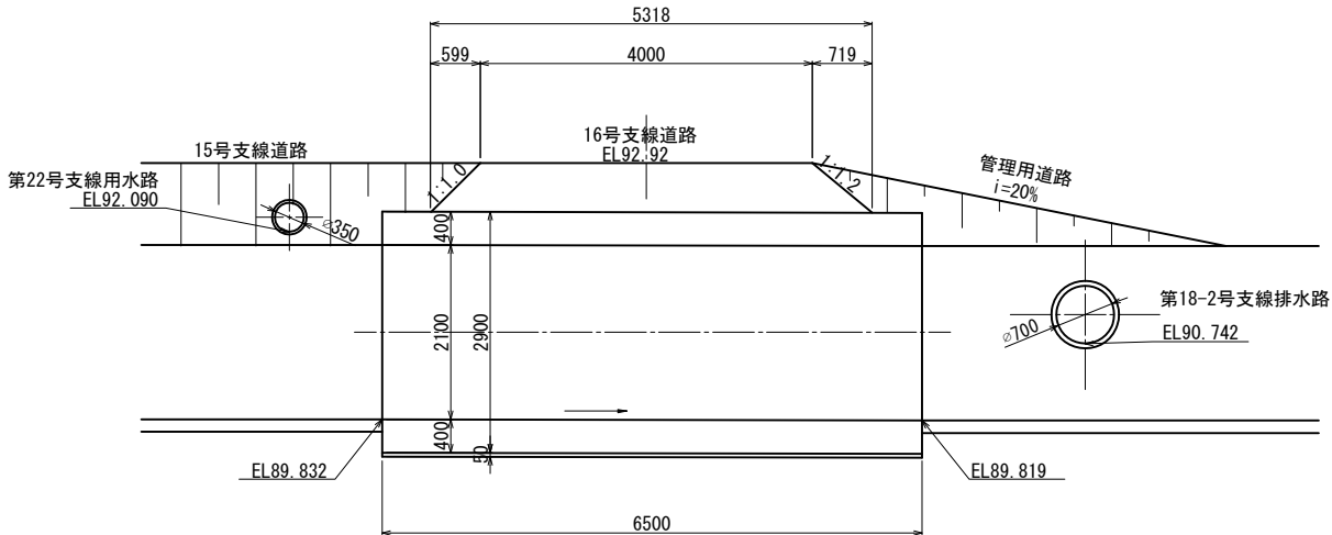
縦断図
