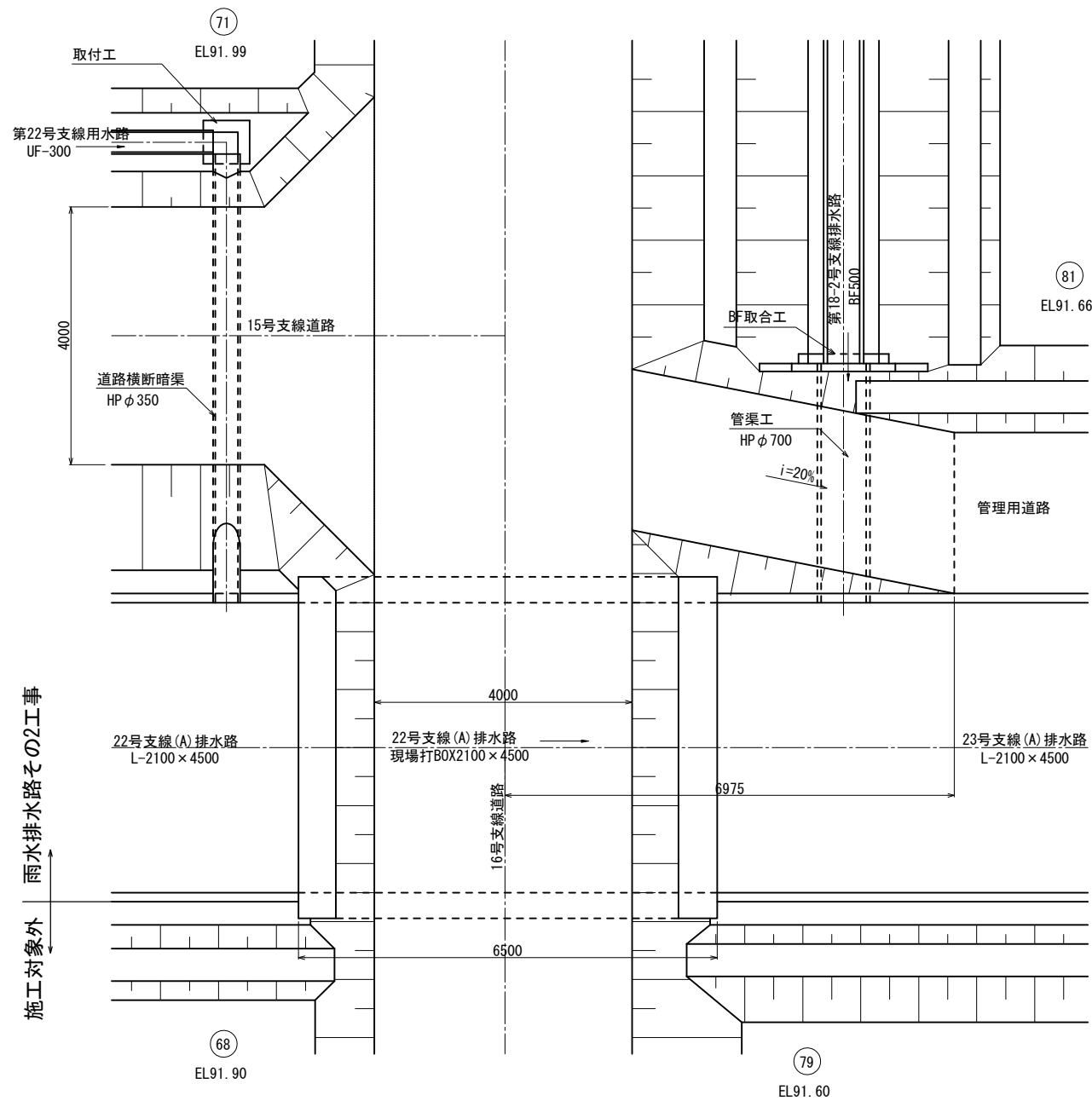
平面図
