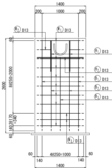
C-C断面図
