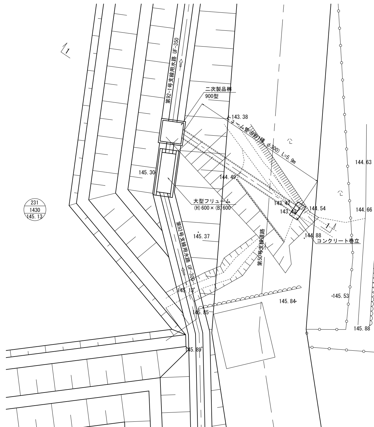
平面图 S=1:50
