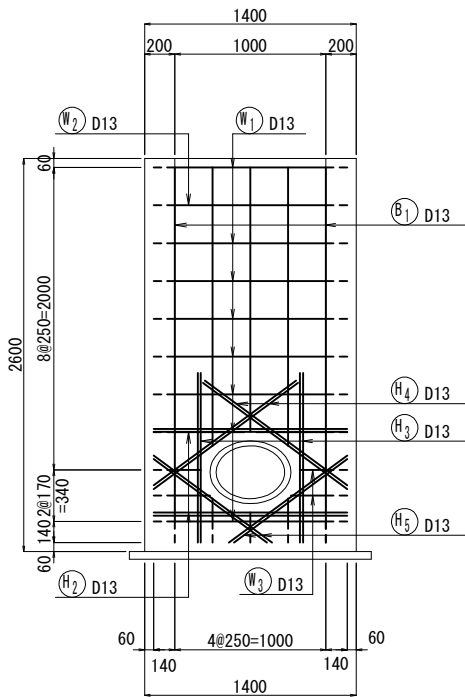
C-C断面図
