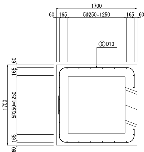
C-C断面図
