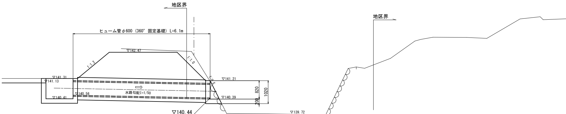
横 断 図 S=1:50
