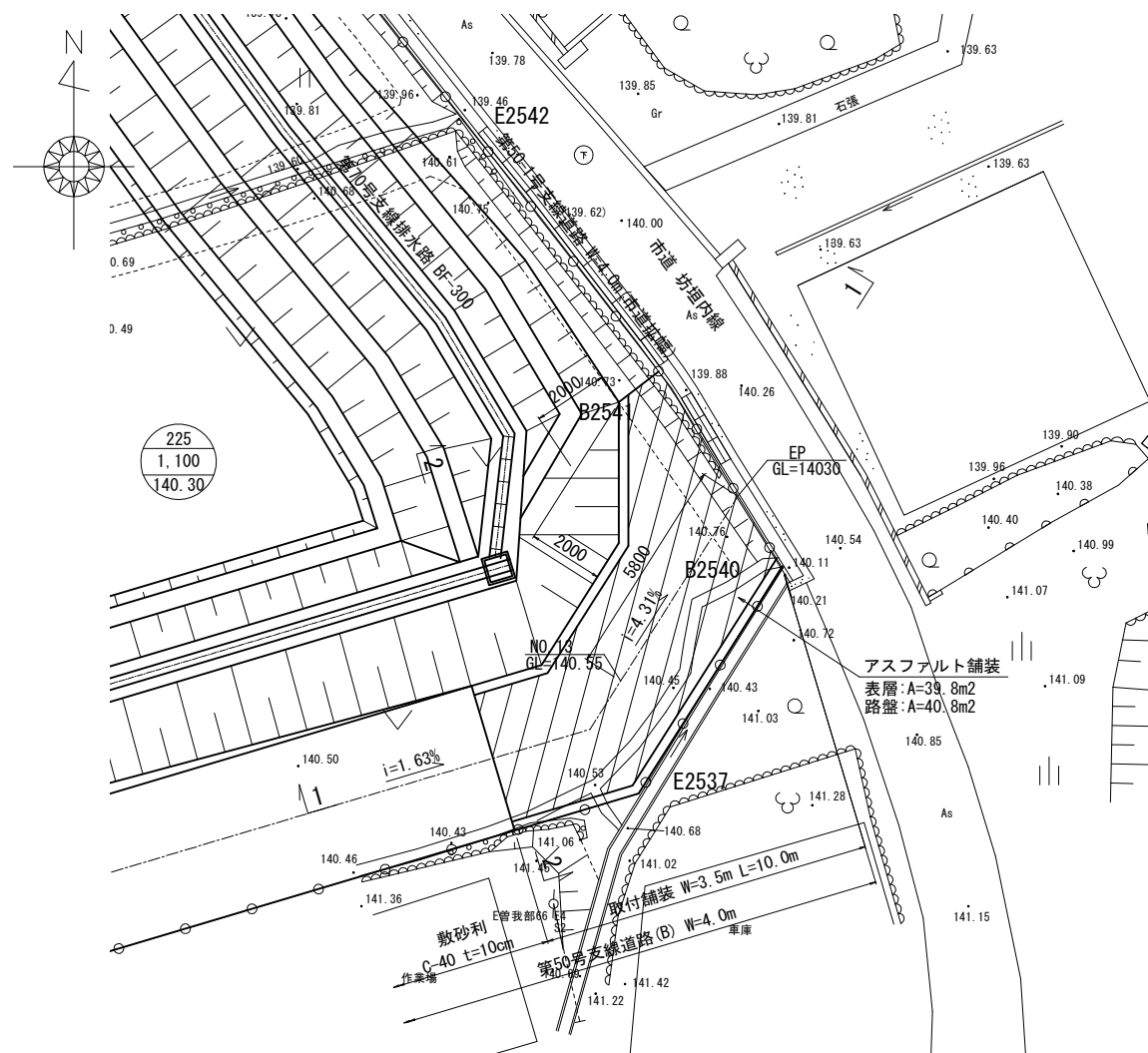
平面图
