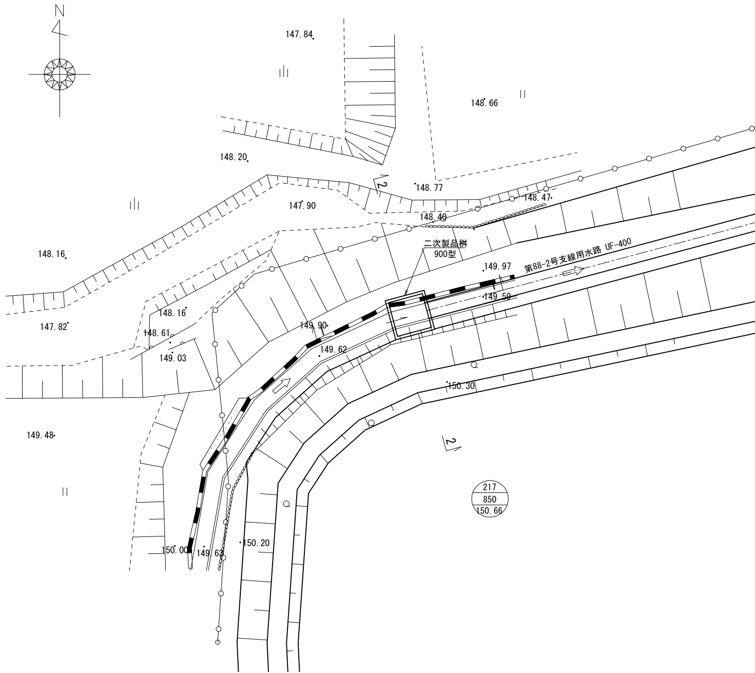
平面図
