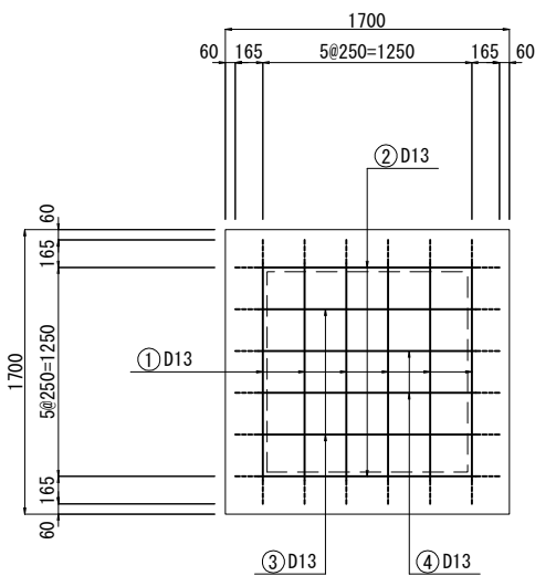
底版
