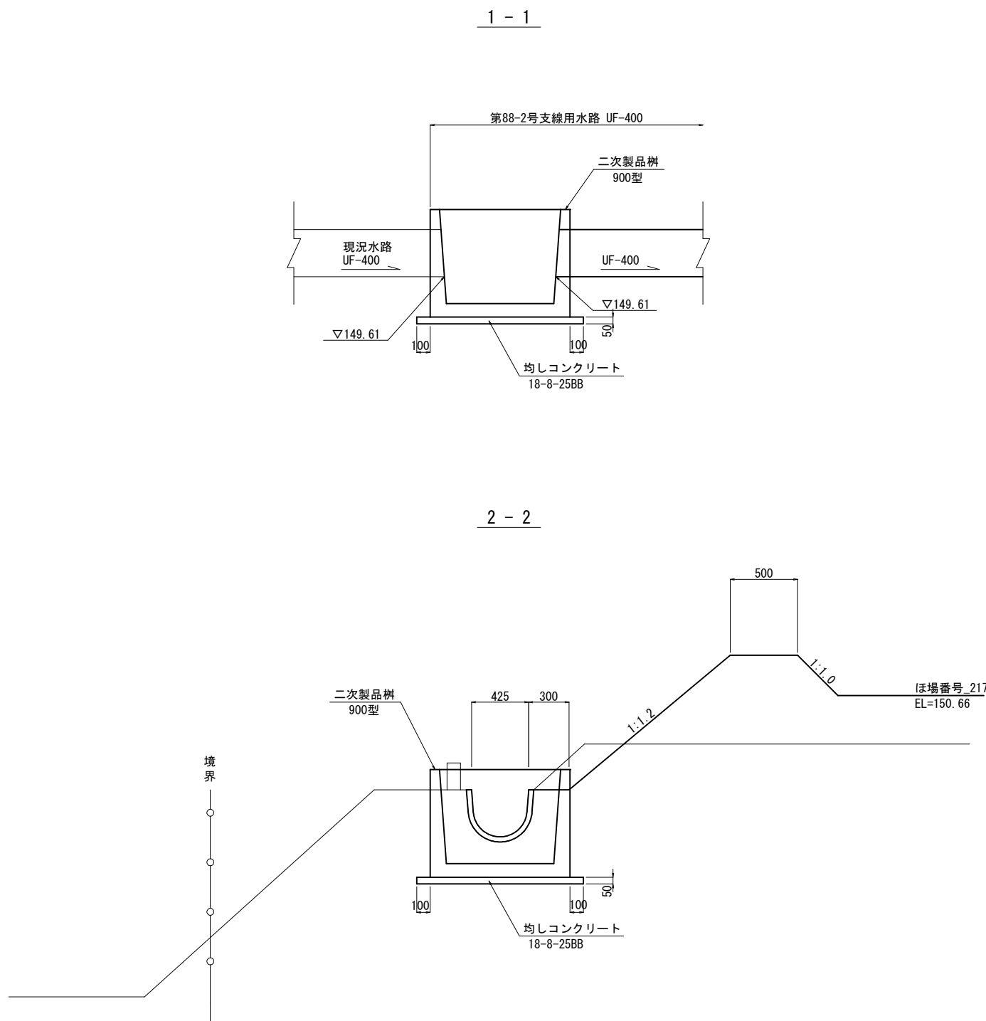
断面図
