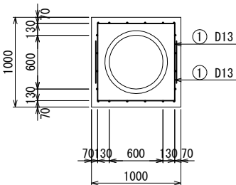
(平面図)
