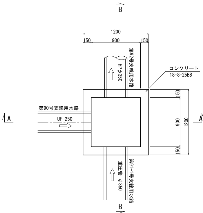
A-A断面図
