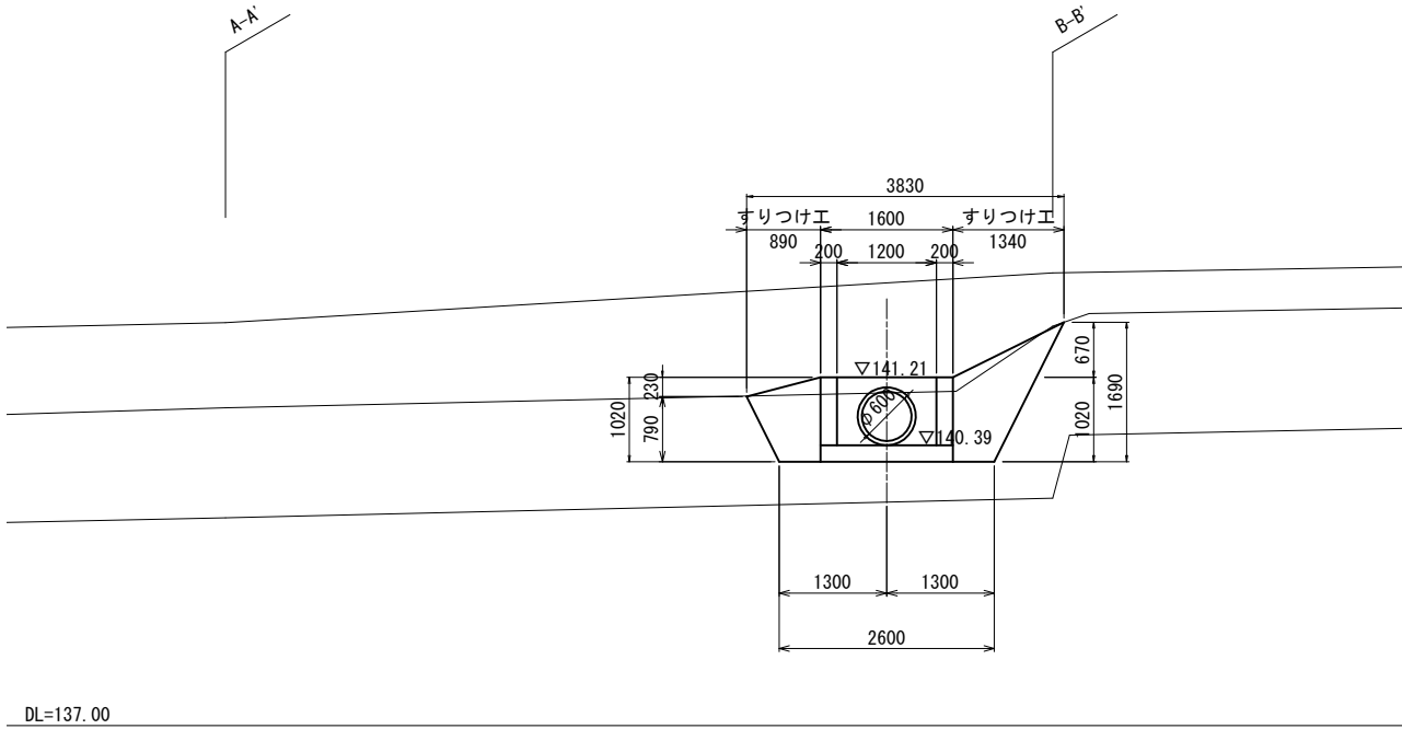
既設護岸復旧工
