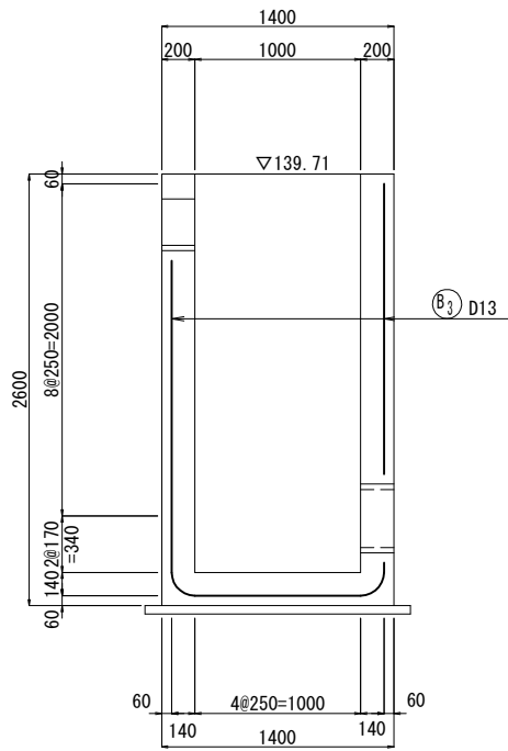
E-E断面図
