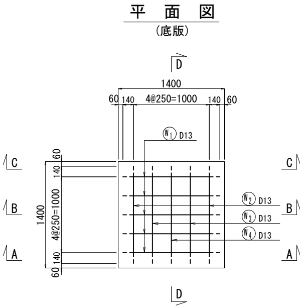
落差柵配筋図
