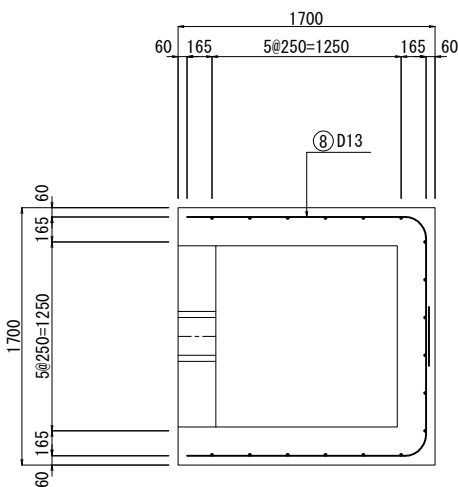
B-B断面図
