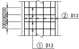
(平面図)
