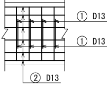
(側面図)
