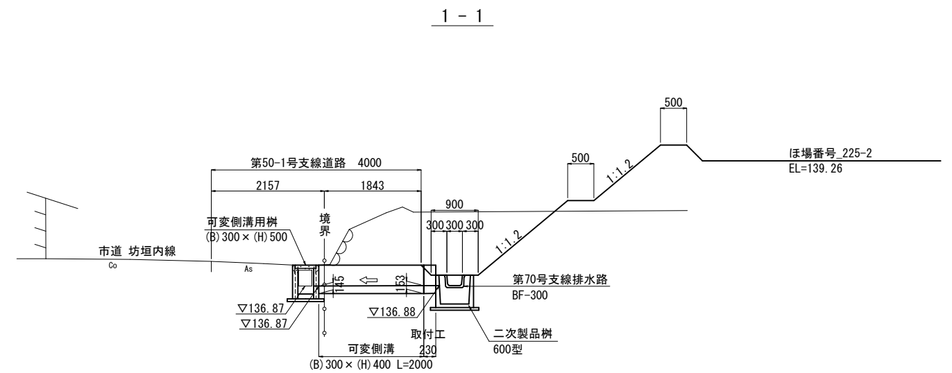
断面図 S=1:50
