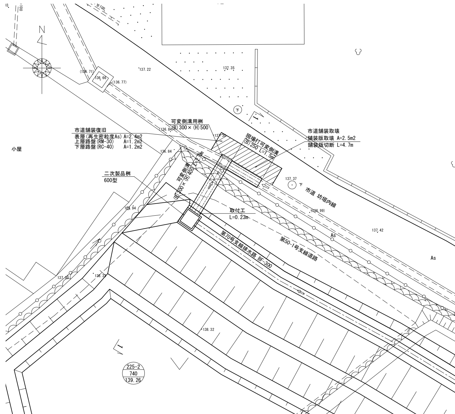
平面图 S=1:50
