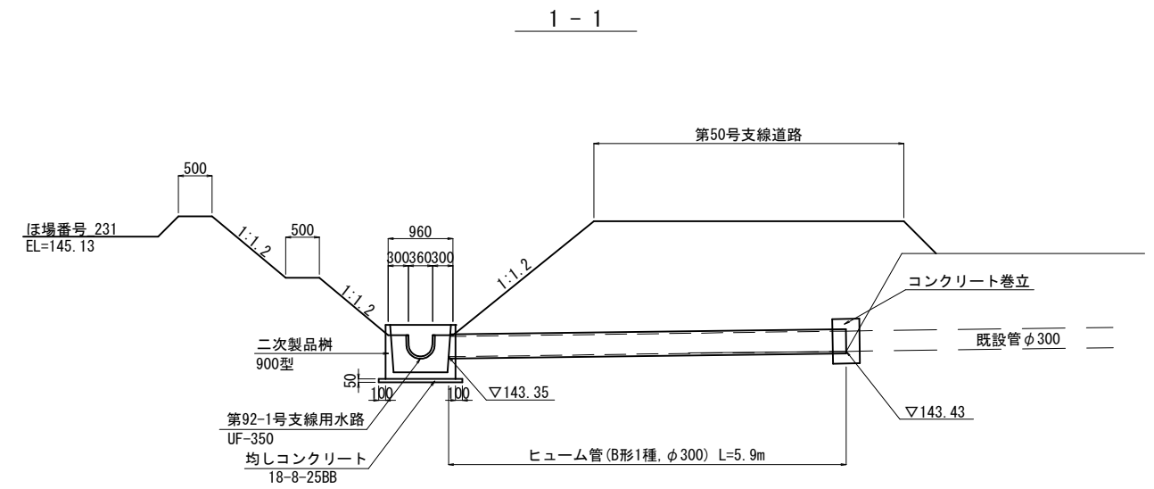
断面図 S=1:50
