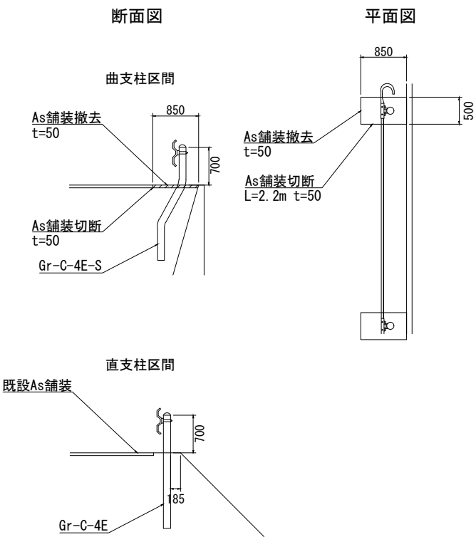
安全対策工 【10-1】
