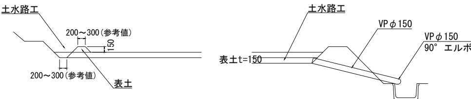
湧水処理工（タイプⅡ） 【15-2, 3】
