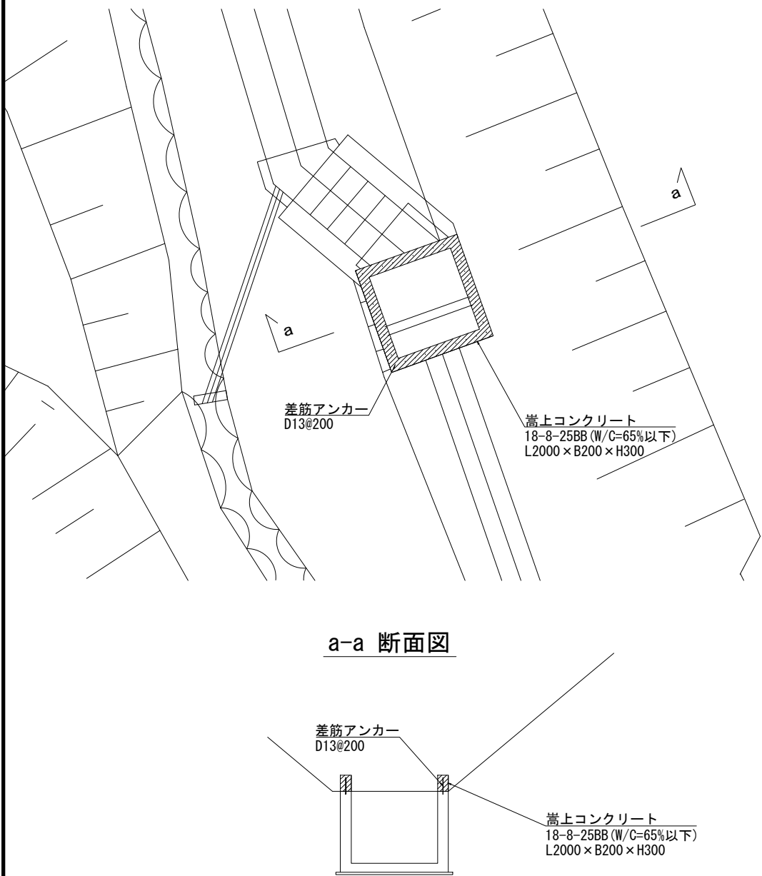
既設柵嵩上げ工
