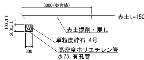
湧水処理工（タイプⅠ） 【13-1, 16-1, 2, 3】
