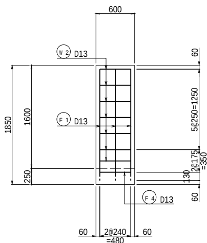
底板上面
