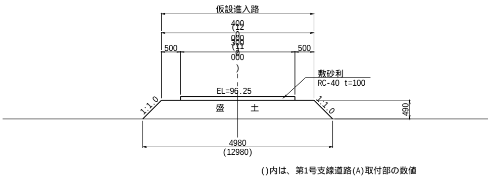
断面図 S=1:50
