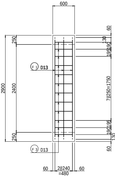
底板下面
