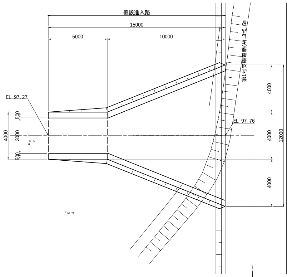
平面図
