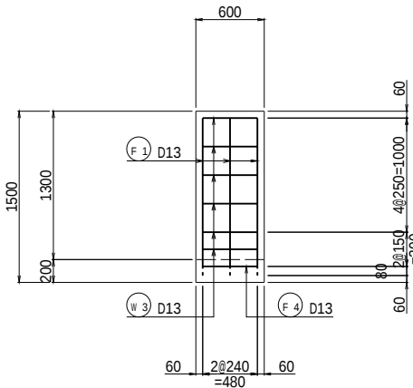
側壁外面
