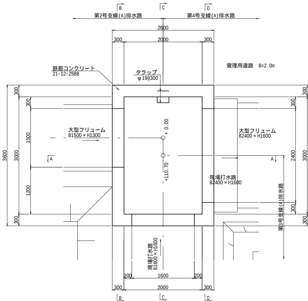
平面図
