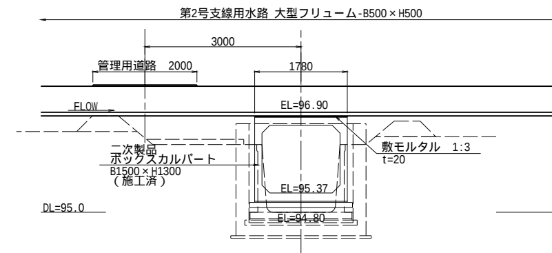
B-B断面図 S=1:50
