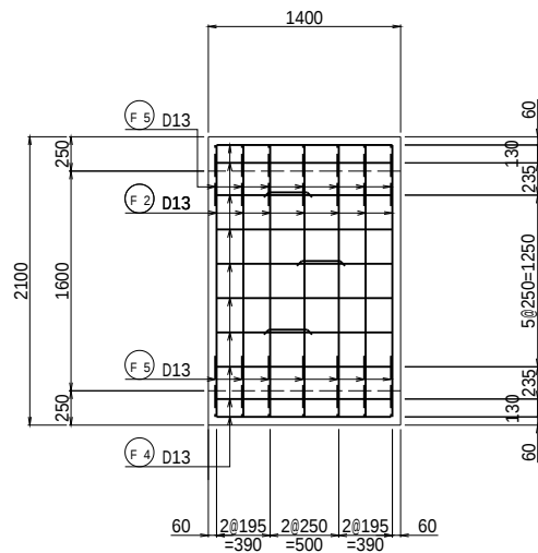
底板上面
