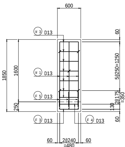
側壁内面
