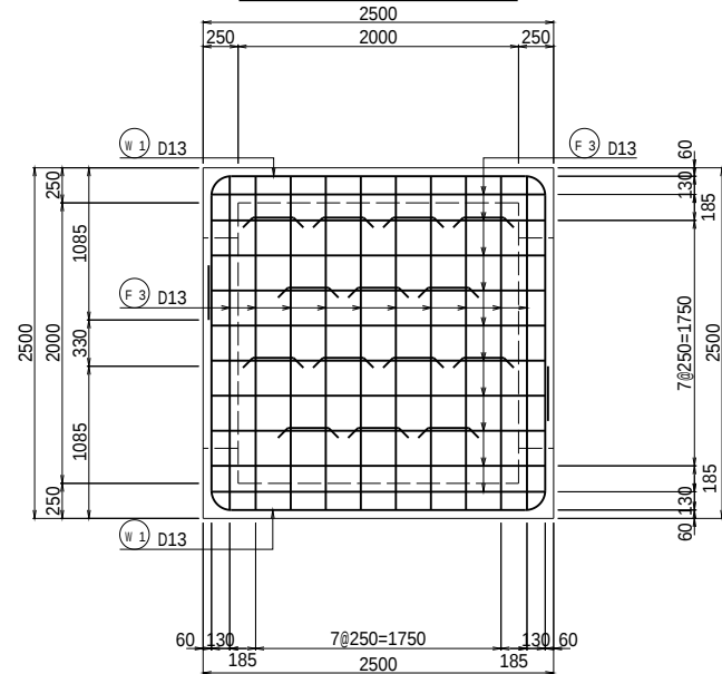
底版下面図
