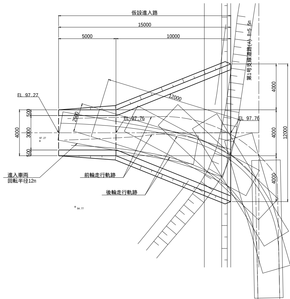
平面図 S=1:100
