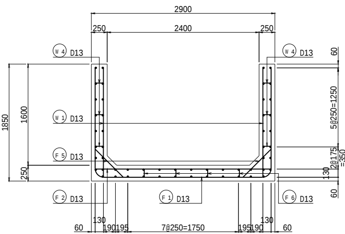
断面図
