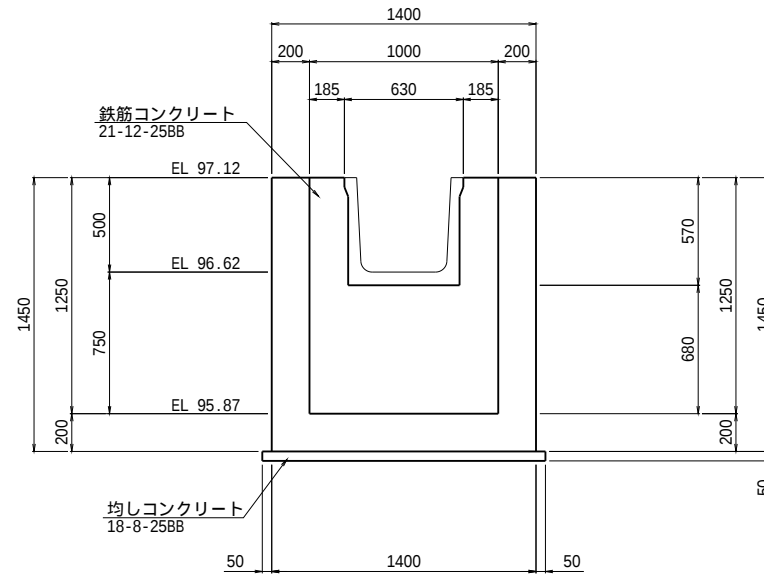
B-B断面図
