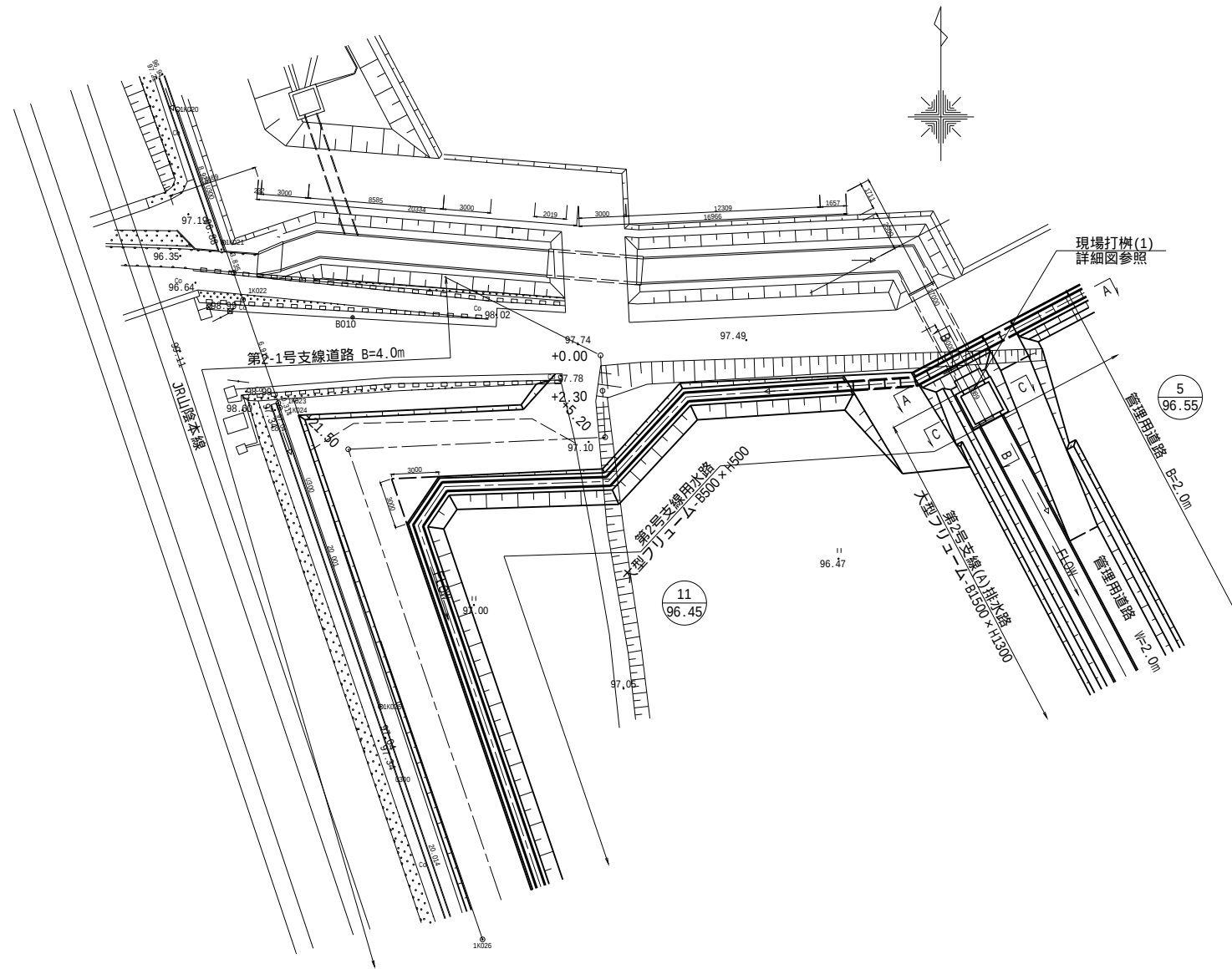
平面図 S=1:200
