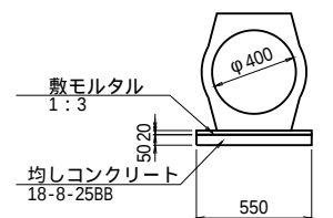
重圧管断面図 S=1:20
