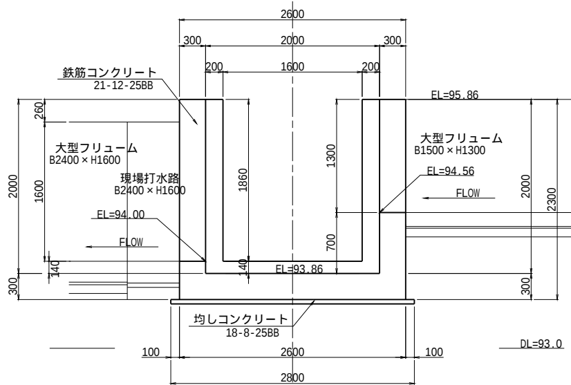
A-A断面図
