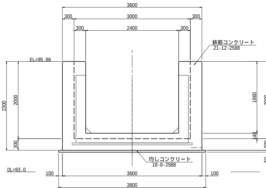
D-D断面図
