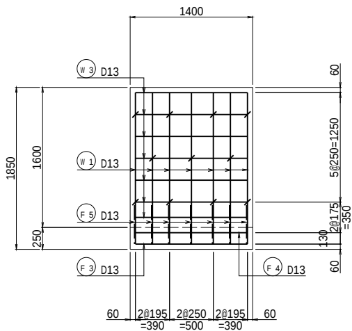
側壁内面
