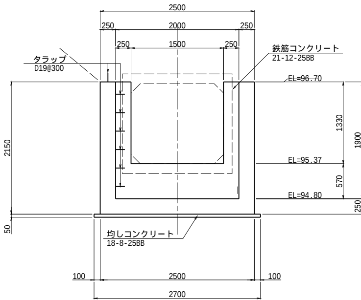
B-B断面図
