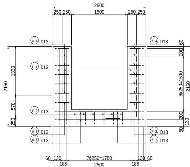
D - D外面補強筋
