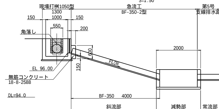
C-C断面図 S=1:50
