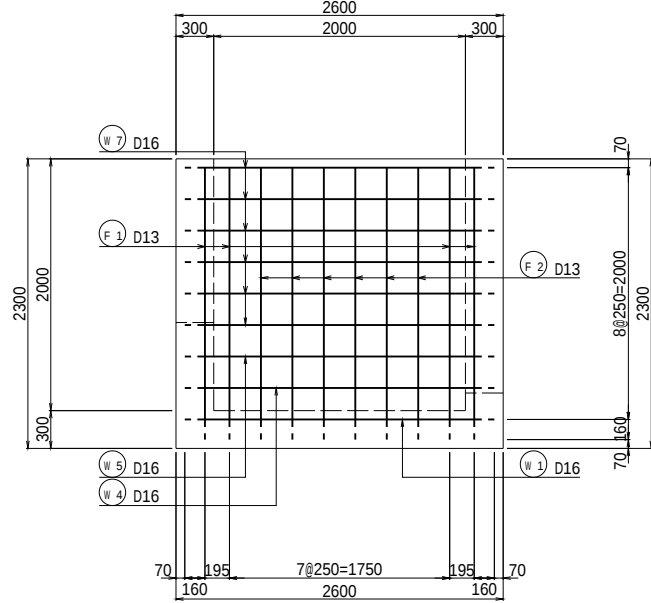
D - D外面図
