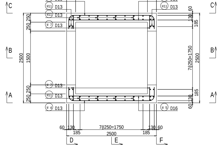
底版上面図
