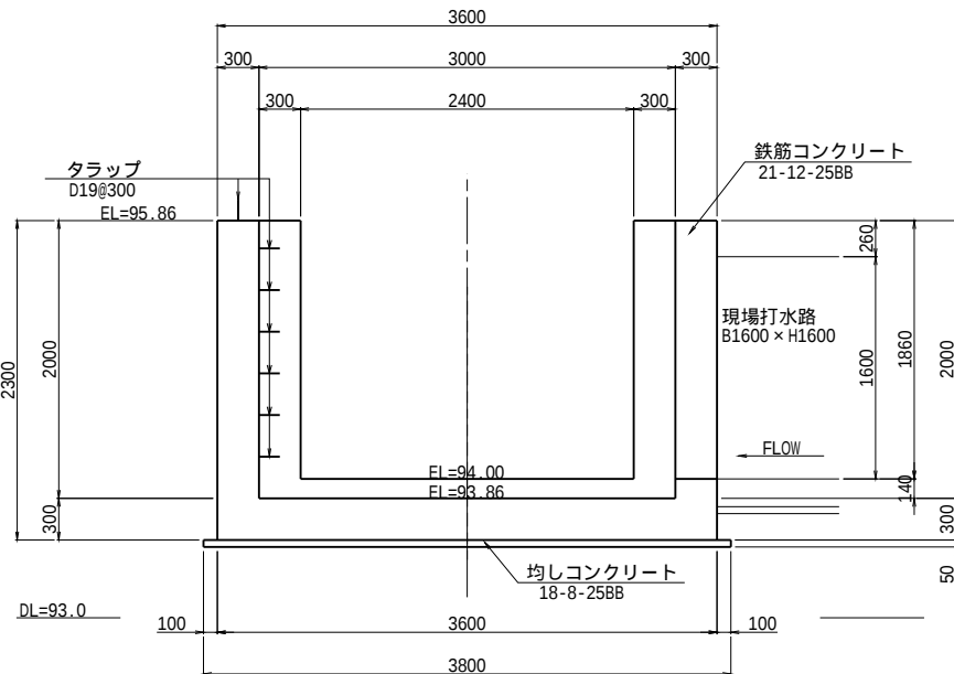
C-C断面図
