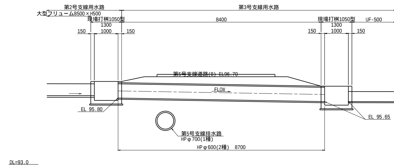
B-B断面図
