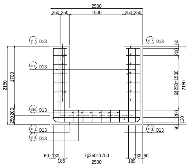
F - F内面図
