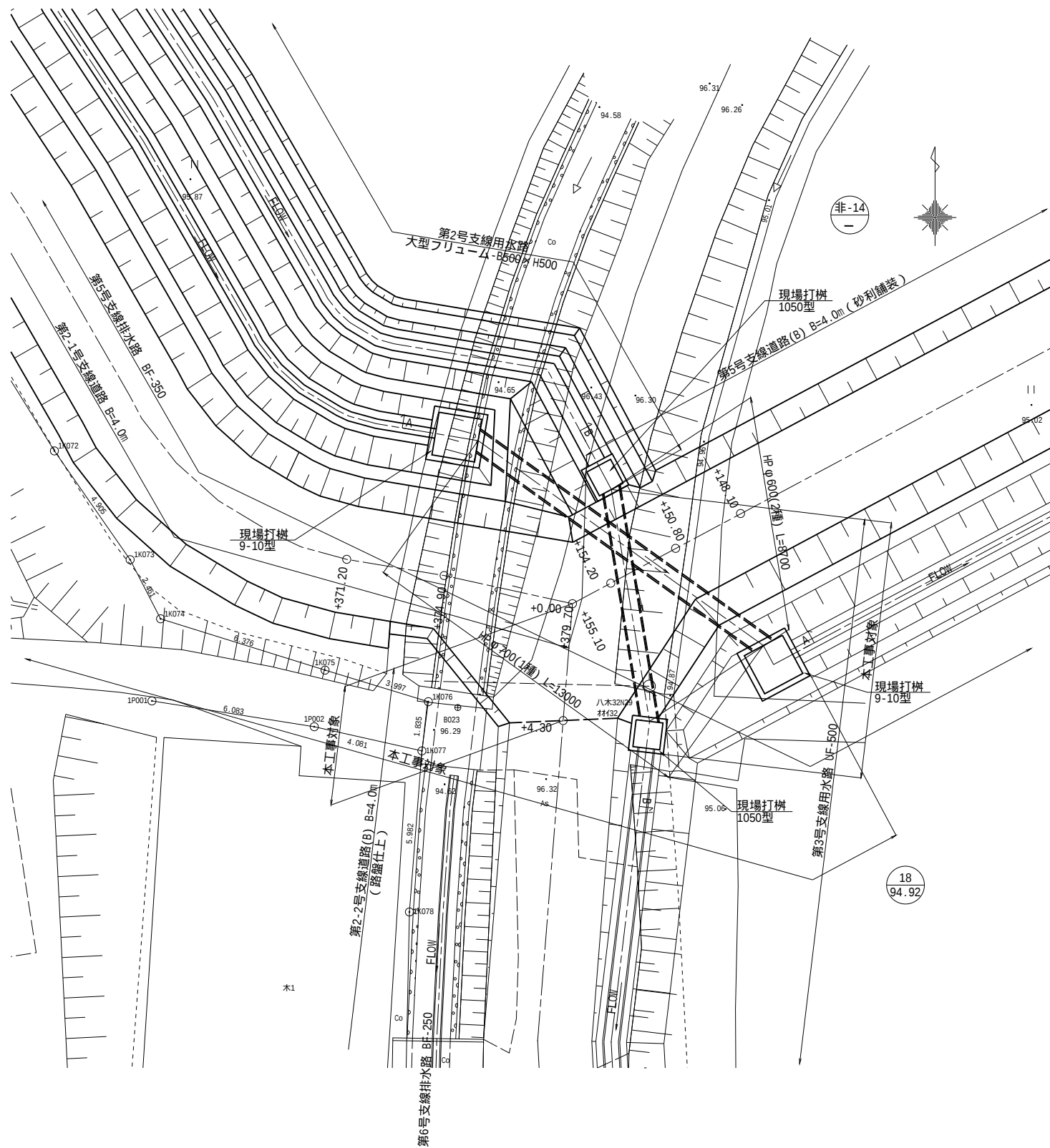
平面图
