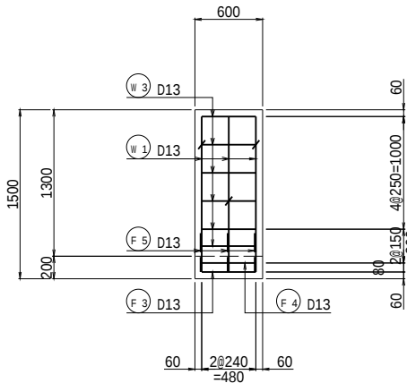
側壁内面
