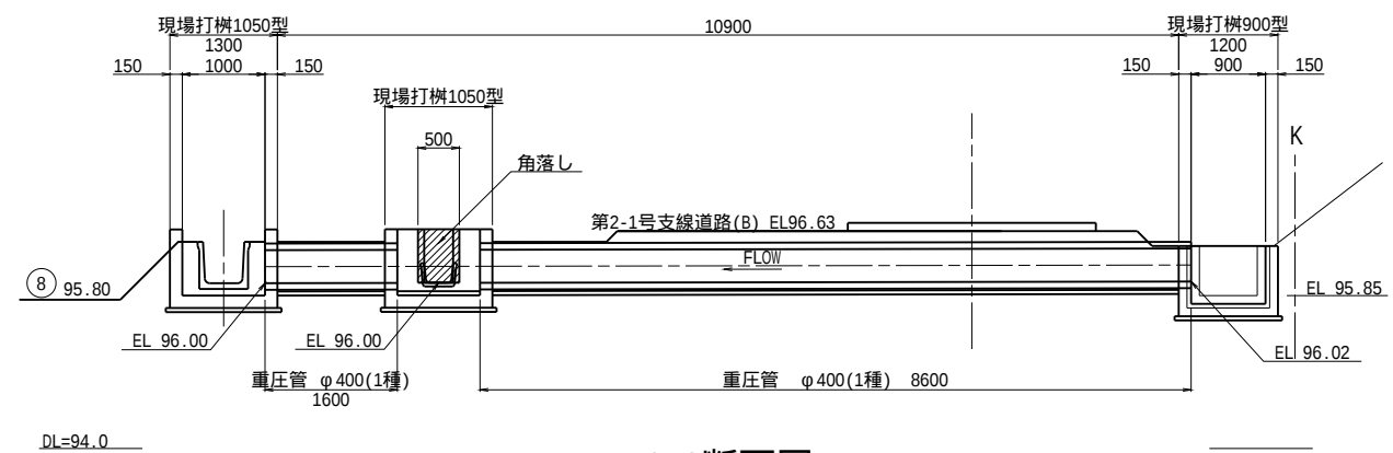
C-C断面図 S=1:50
