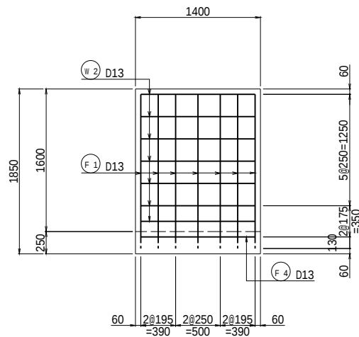
底板上面
