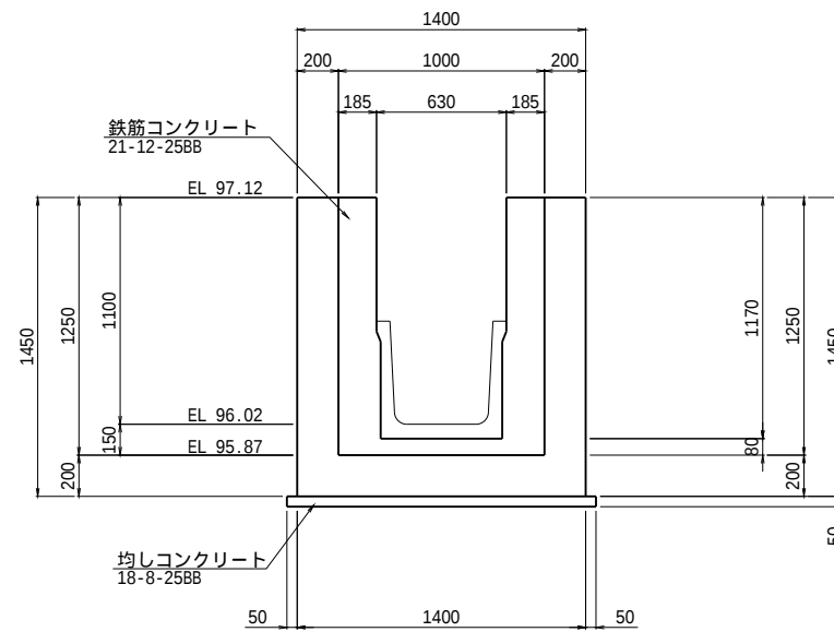
C-C断面図
