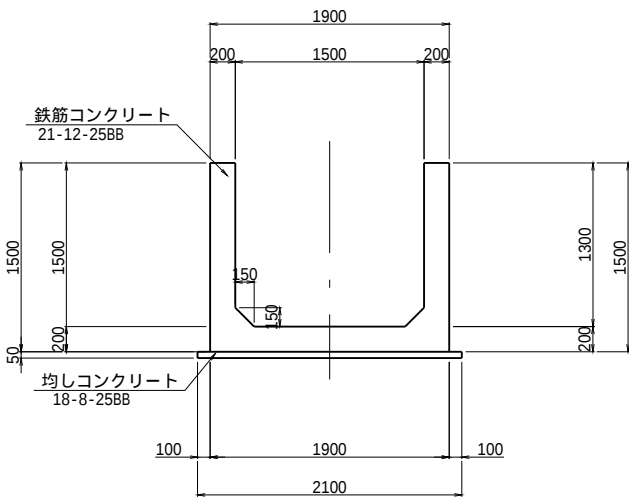
断面図
