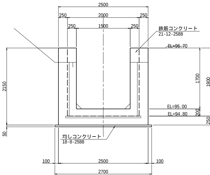
C-C断面図
