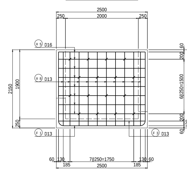
C - C内面図
