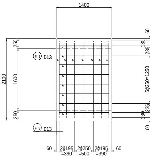
底板下面
