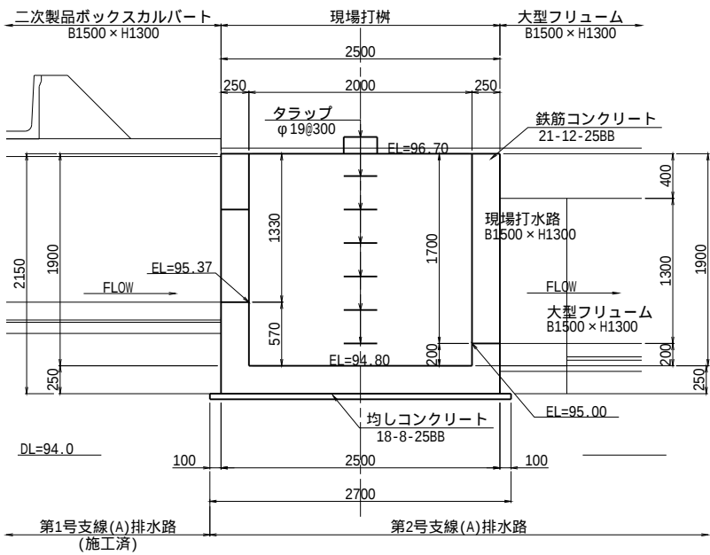
A-A断面図
