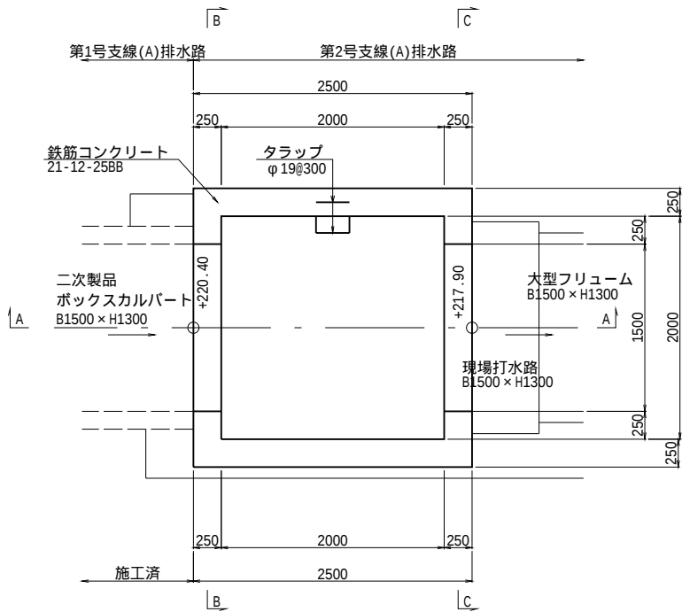
平面図
