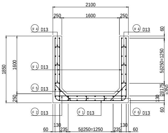
断面図
