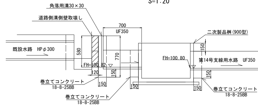
A-A' 断面図
