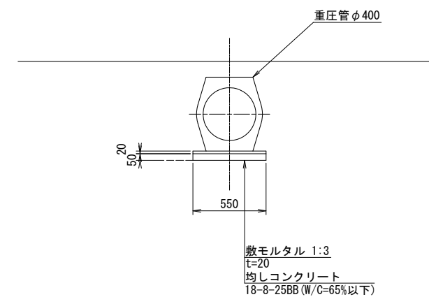
道路横断暗渠断面图 S=1:20
