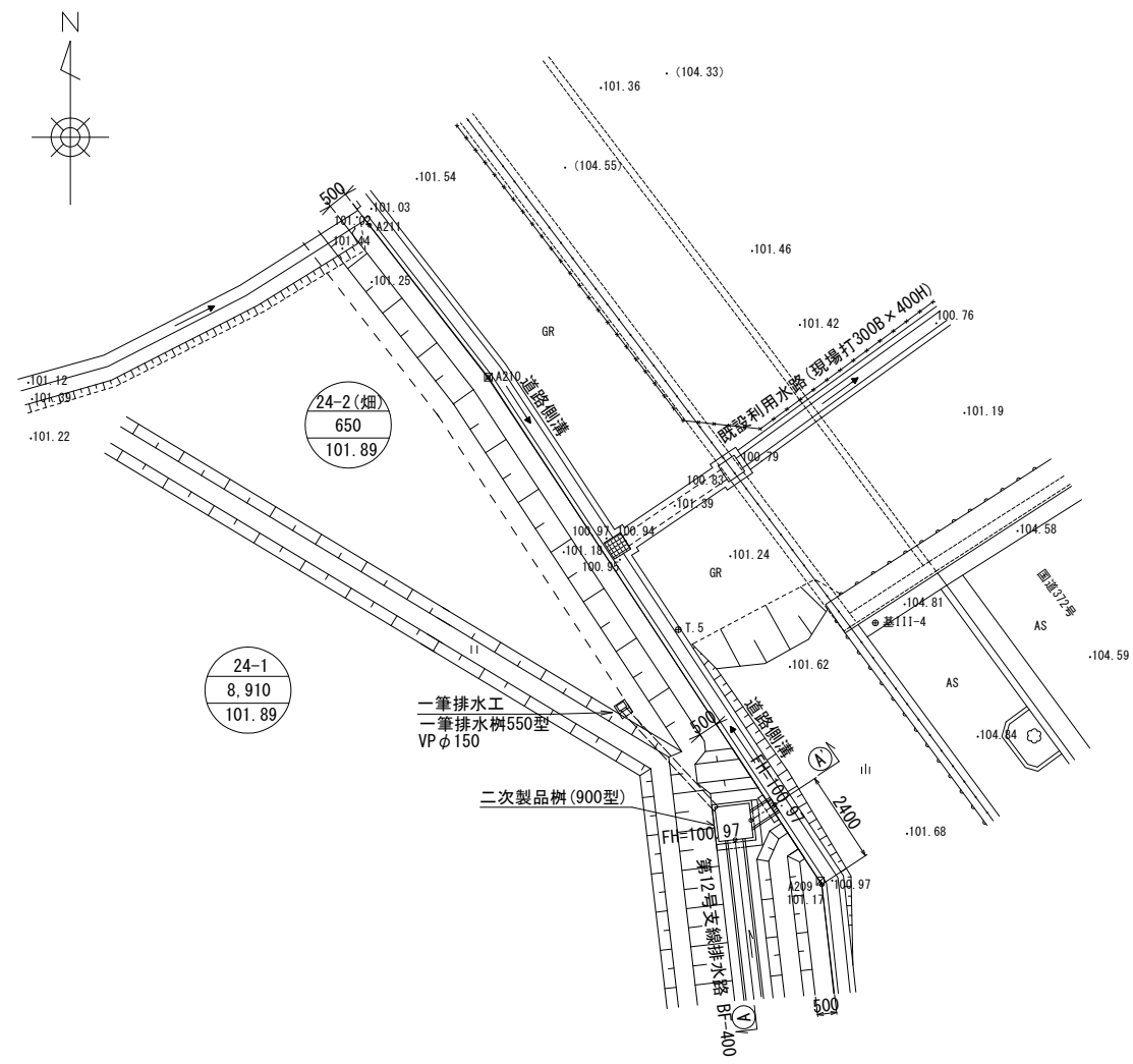
平面図 S=1:100
