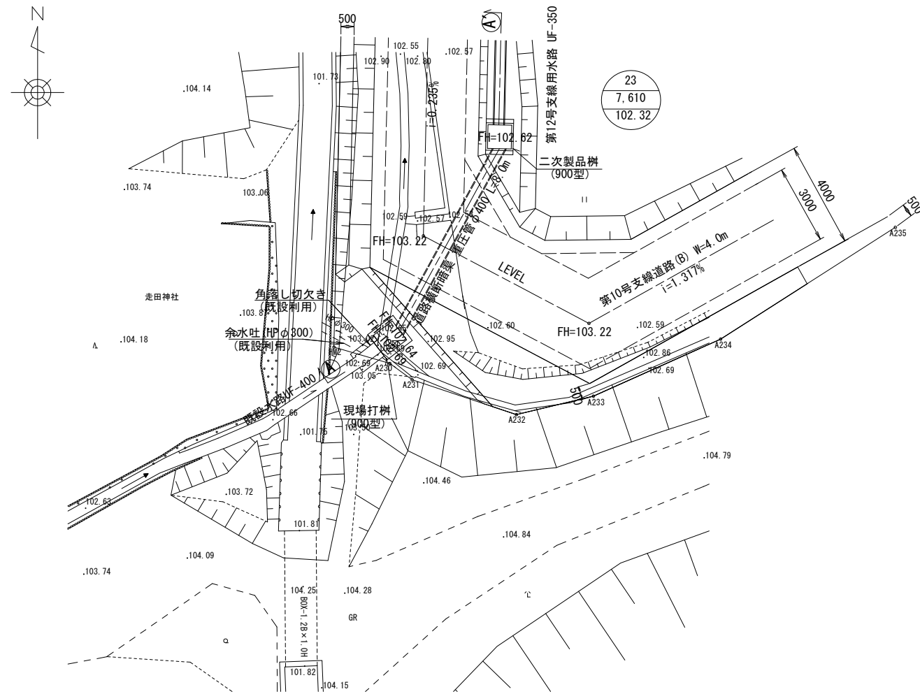
平面图 S=1:100
