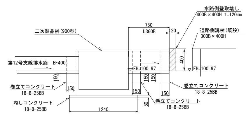
①-①'断面図 S=1:20
