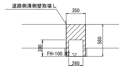
C-C' 断面図
