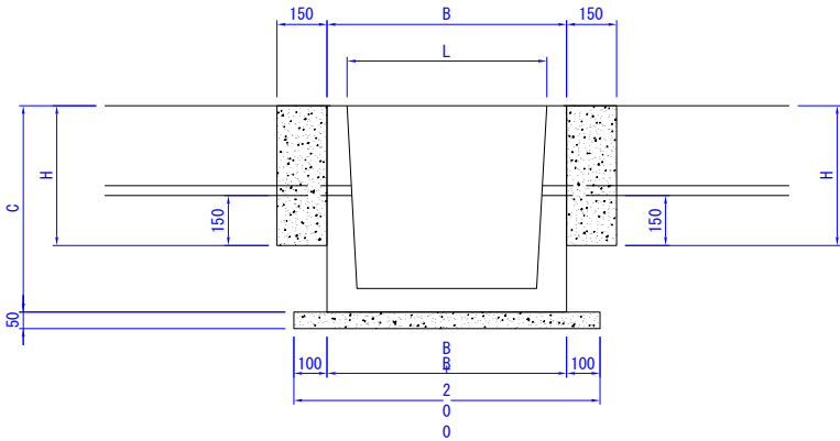
側面図
