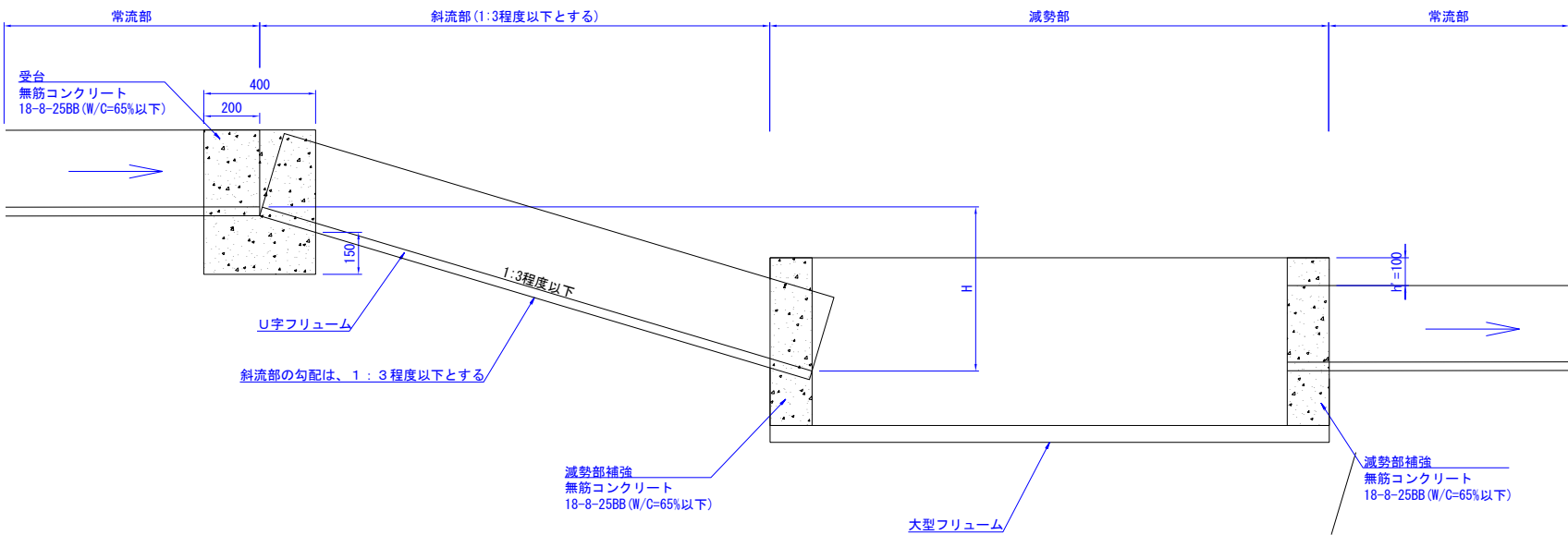
縦断面図
