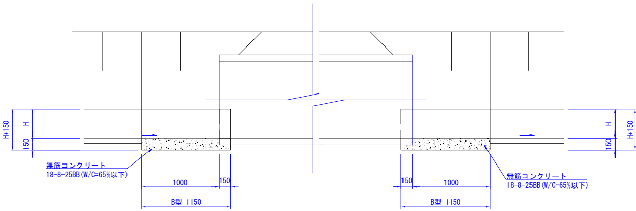
縦断面図
