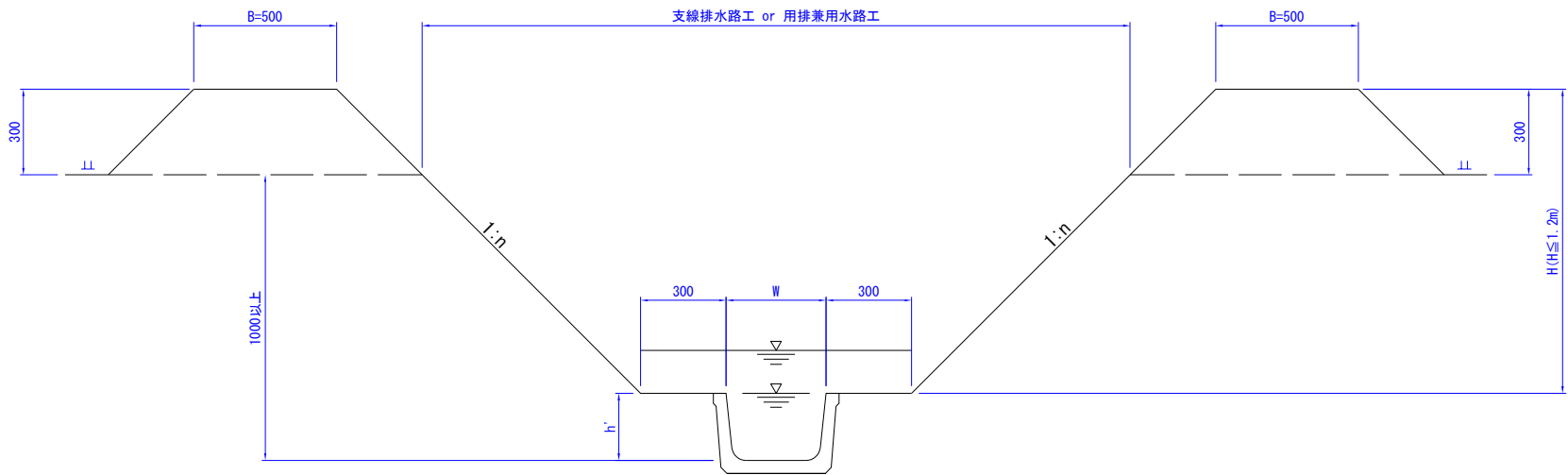
断面図
