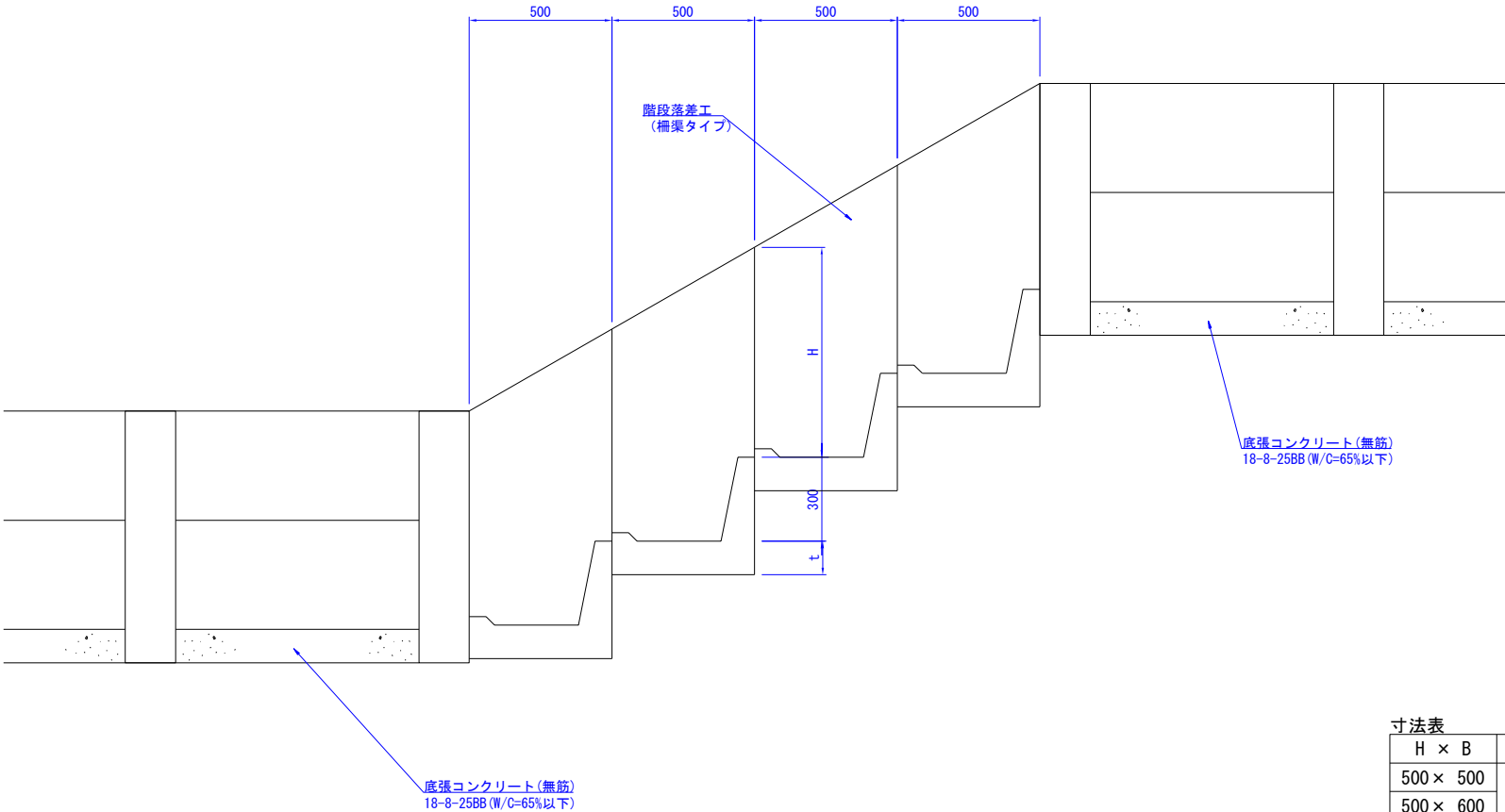
側面図
