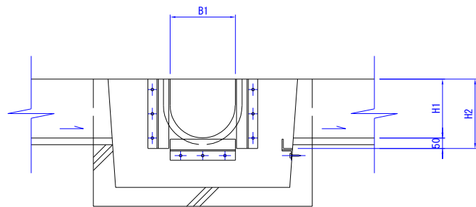
断面図
