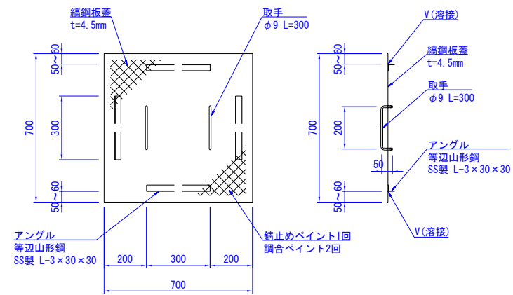
600型
