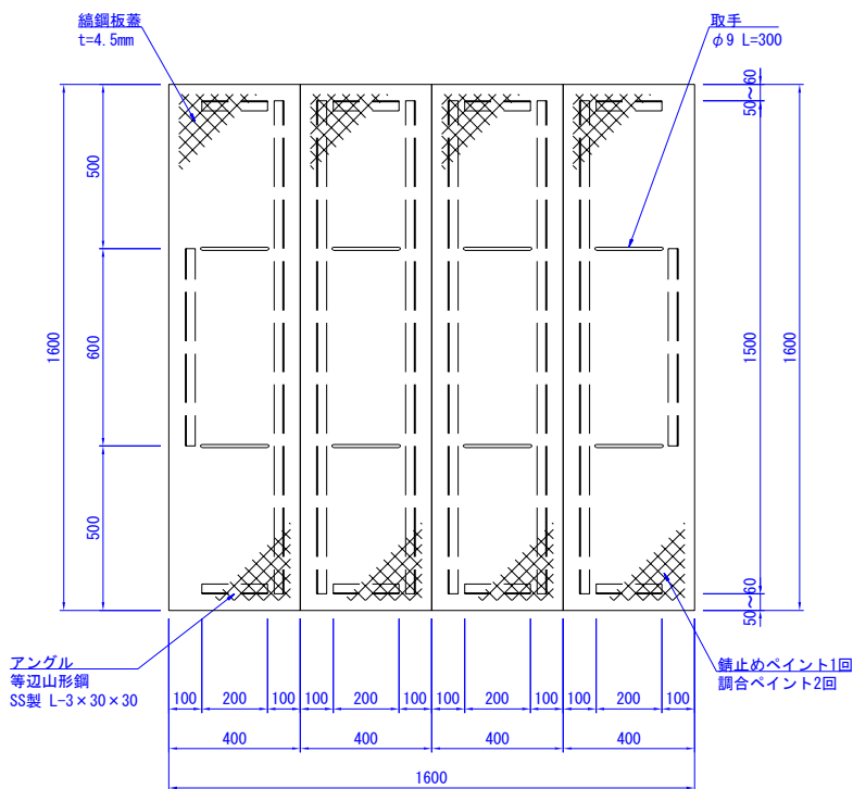
1500型 (4枚割り)
