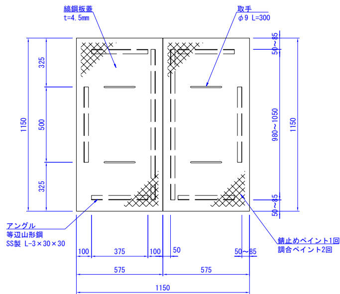
1050型 (2枚割り)
