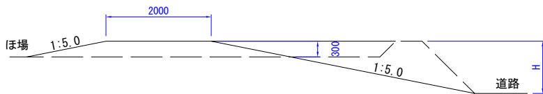
側面図
