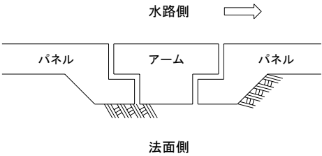
B型平面構造
