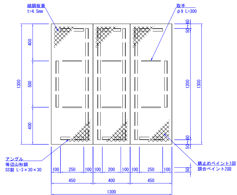
1200型 (3枚割り)
