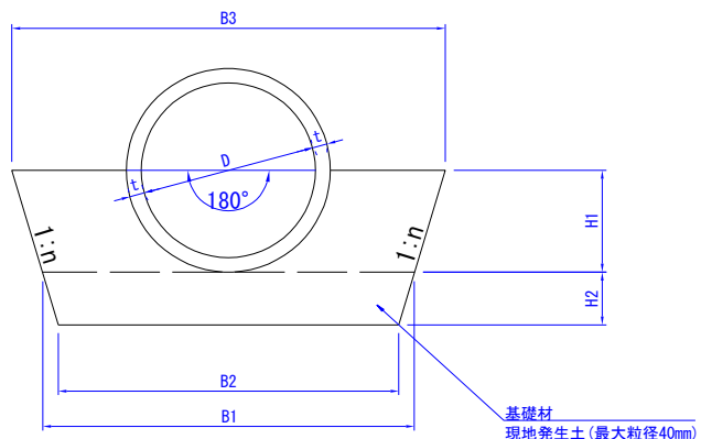
180° 自由基礎
