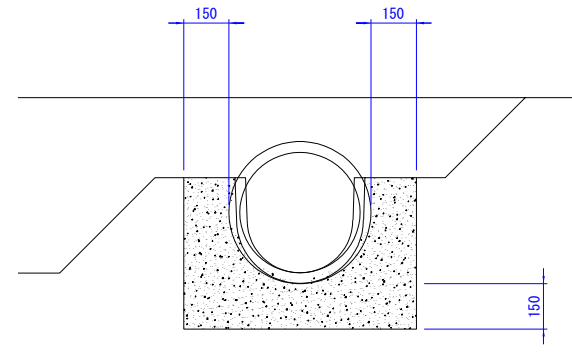
正面図
