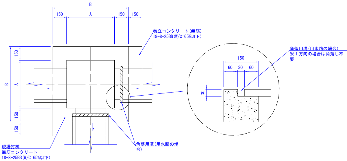
平面図(用水路の場合)
