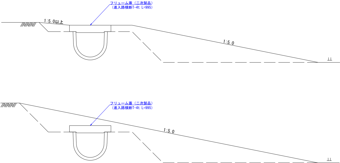
進入路暗渠 (UF)
