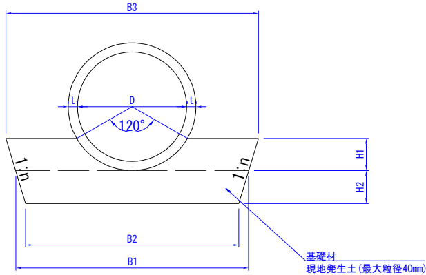
120° 自由基礎
