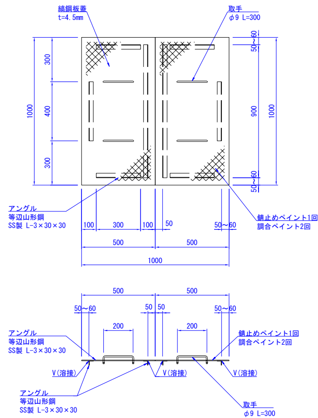
900型 (2枚割り)
