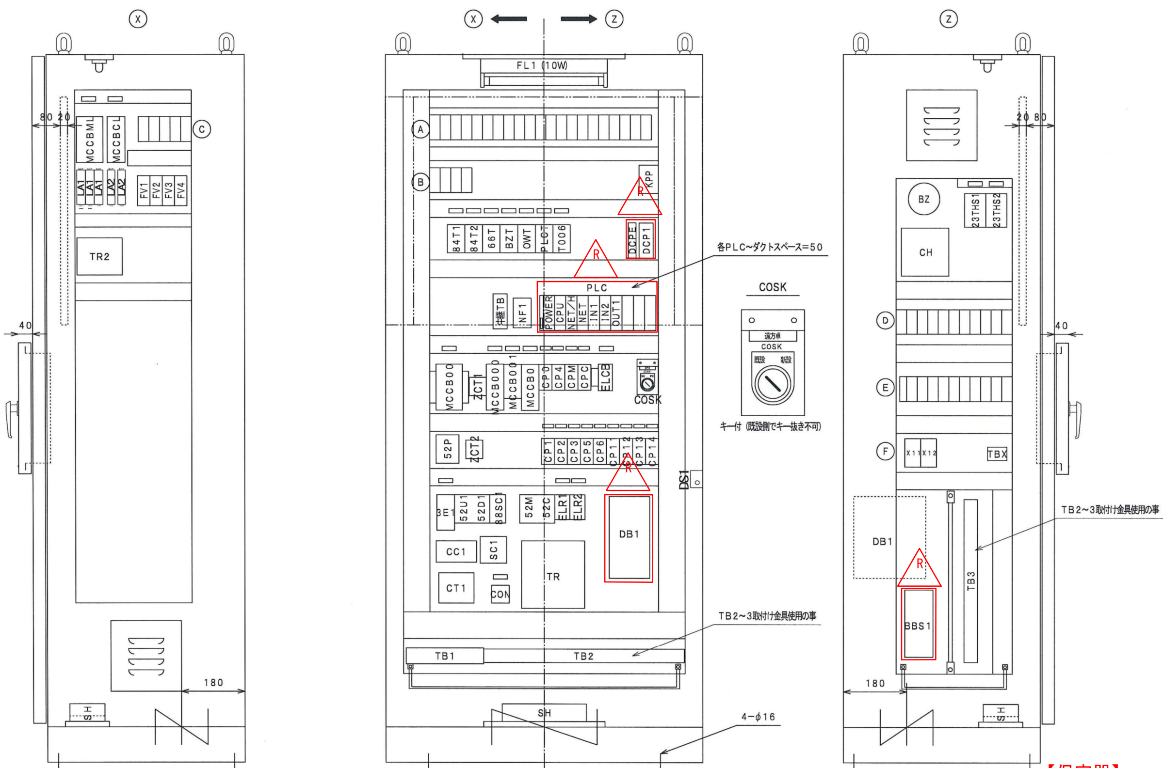
洪水吐ゲート機側操作盤 外形図・盤内配置図
