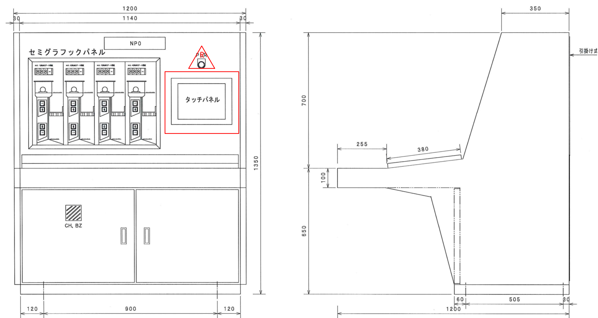
外形図
