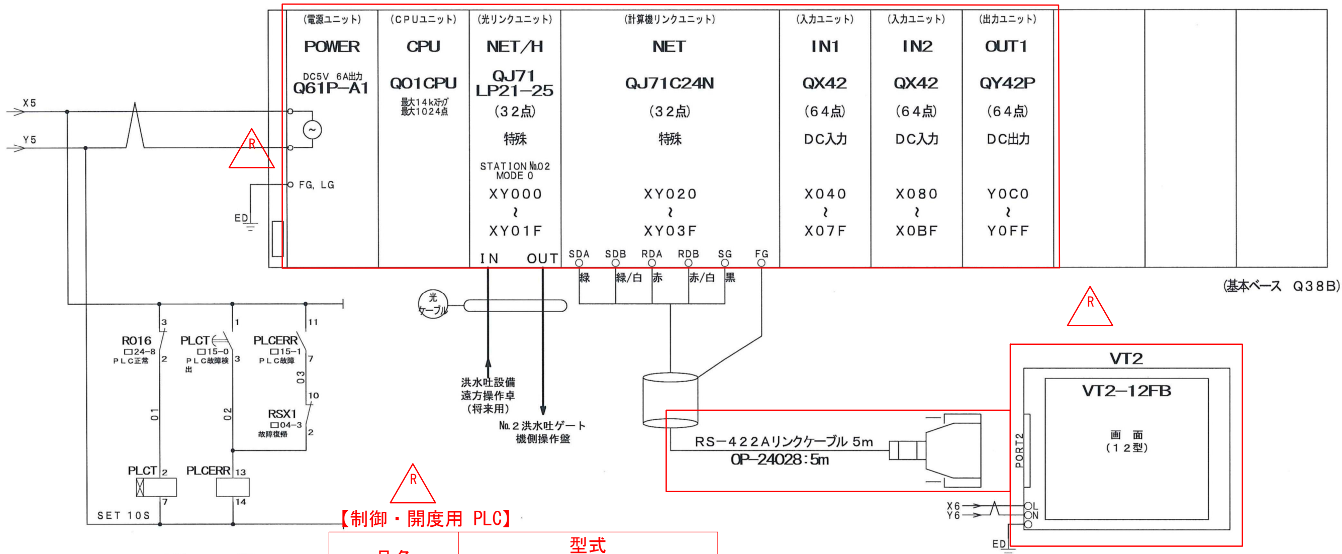
洪水吐ゲート機側操作盤 P L C 構成図
