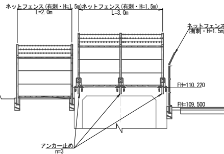
横断面 S=1:50
