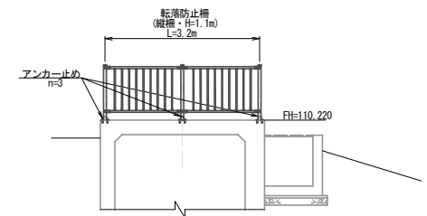
水路横断箇所 S=1:50
