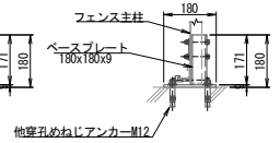
側面図
