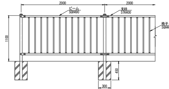
正面図 S=1:20
