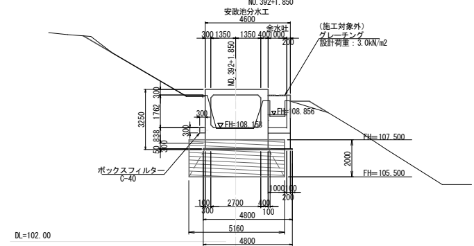
安政池分水工 (B-B断面)
