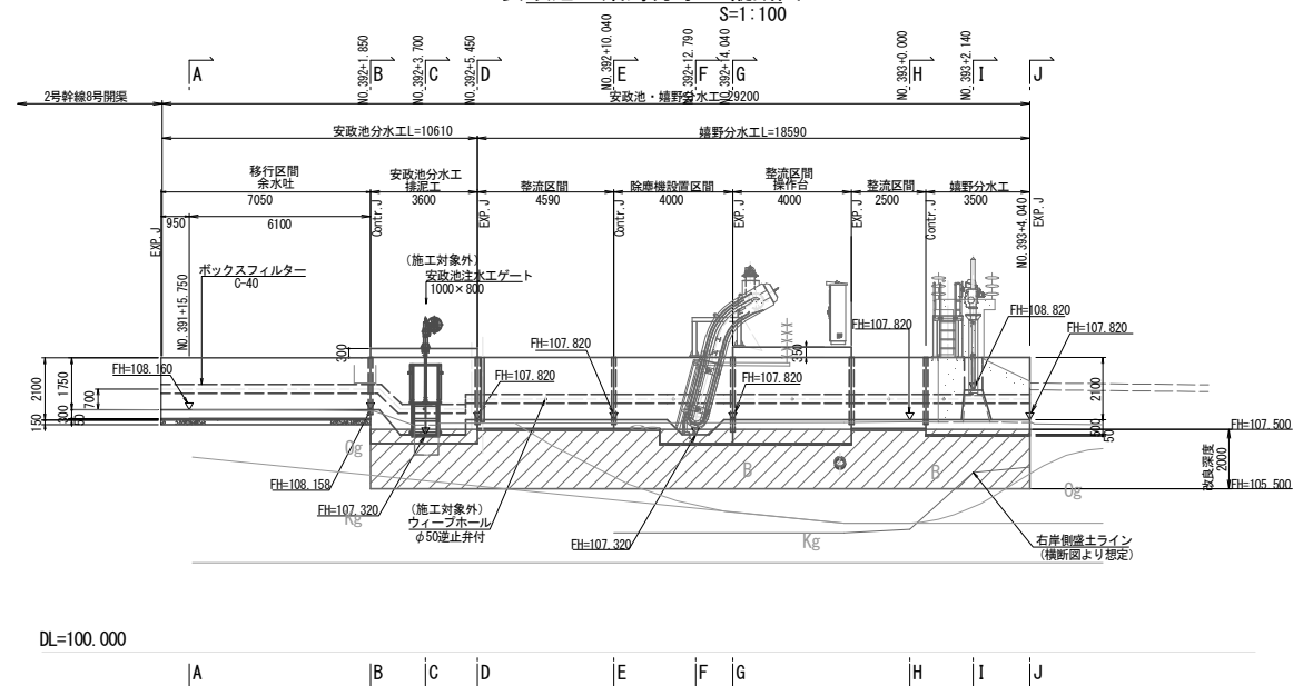
安政池・嬉野分水工縦断面図
