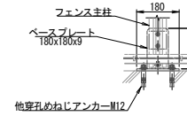
正面図
