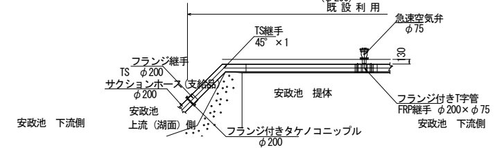
堤体部配管詳細図 S=1/50 (φ200) 既設利用
