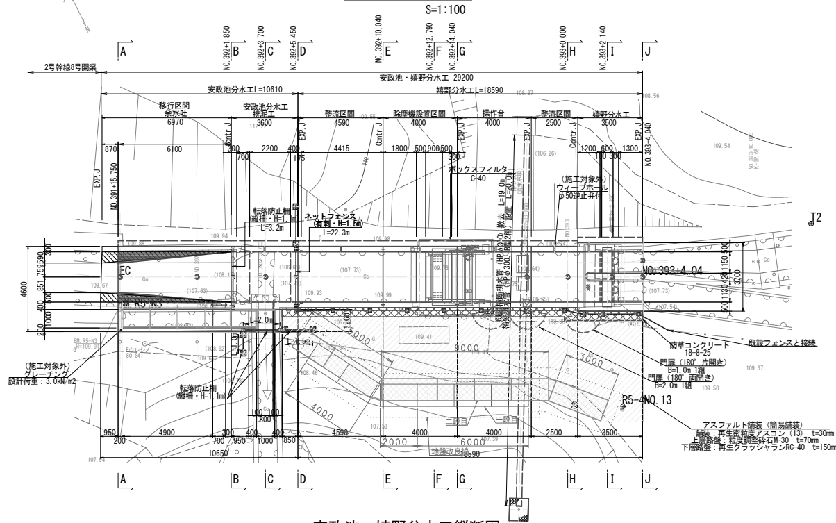
安政池・嬉野分水工縦断面図
