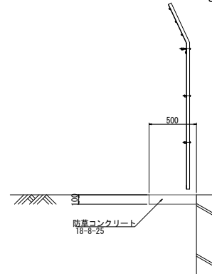
防草コンクリート S=1/20
