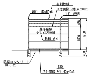
正面図
