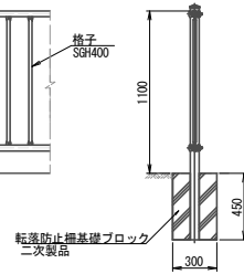
側面図 S=1:20
