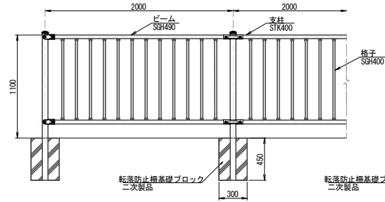
正面図 S=1:20
