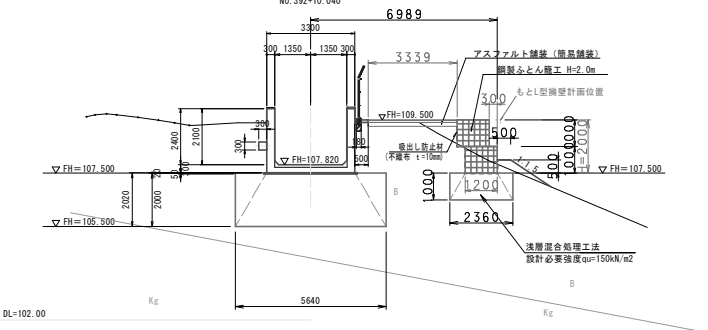
鋼製ふとん籠工 標準断面図
