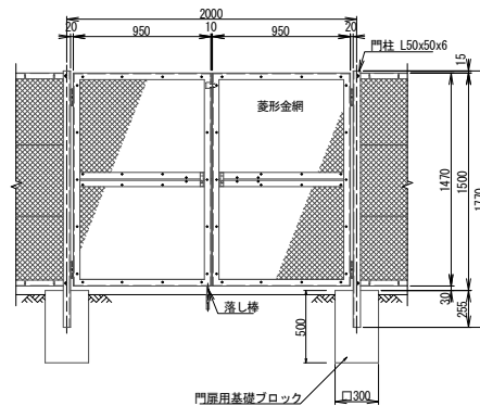
門扉 (ネット式両開) H=1.5m, W1.0m S=1/20
