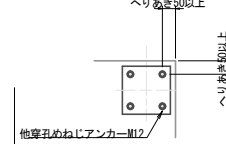
アンカー止め詳細平面図 S=1:10
