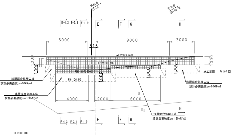
鋼製ふとん籠工正面図
