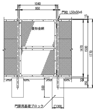
門扉 (ネット式片開) H=1.5m, W1.0m S=1/20
