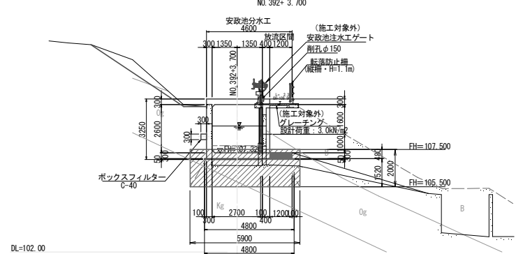
安政池分水工 (C-C断面)
