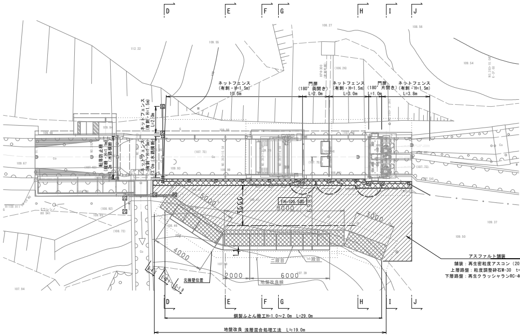
計画平面図
