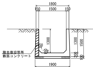
既設水路横断面図 S=1:50
