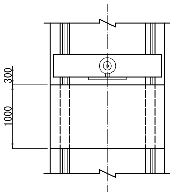
平面図
