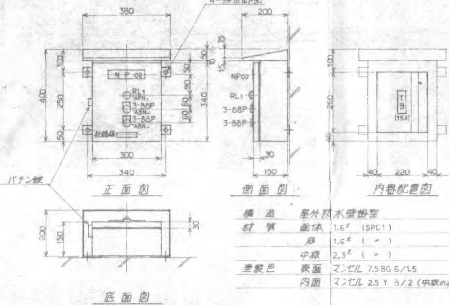
水中ポンプ現場操作盤 1:10
