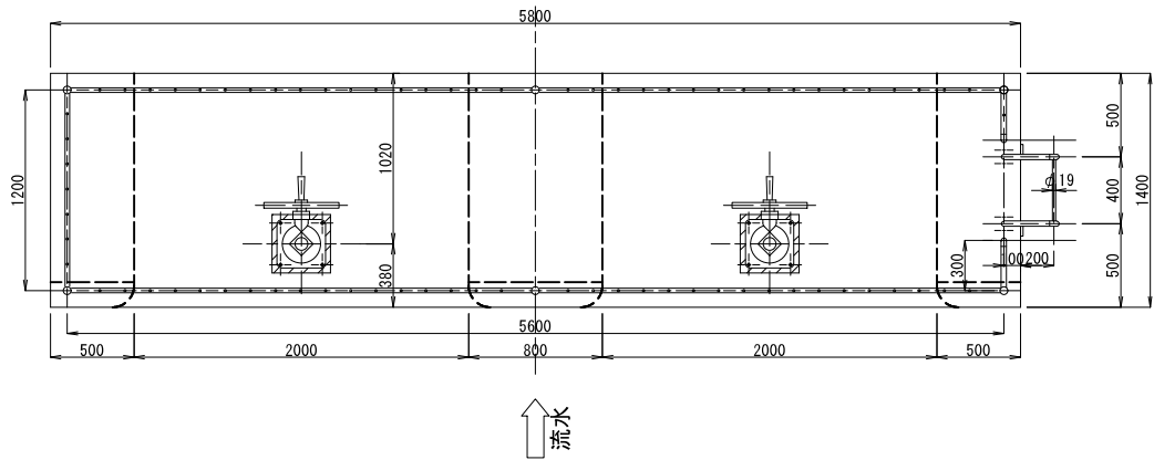
平面図
