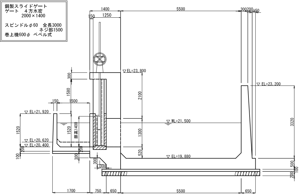
A-A' 断面
