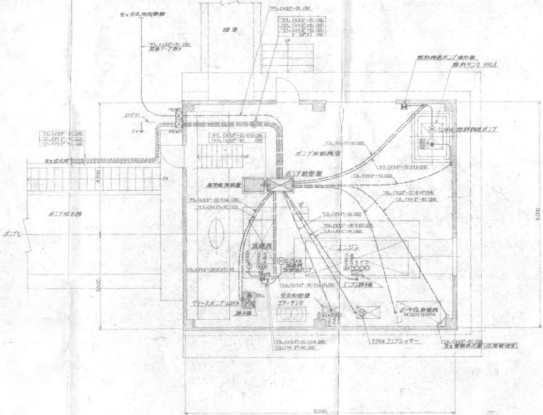
原動機室内ケーブル接続図 1/50
