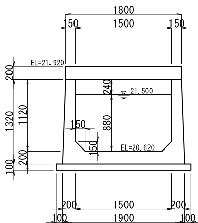
断面図
