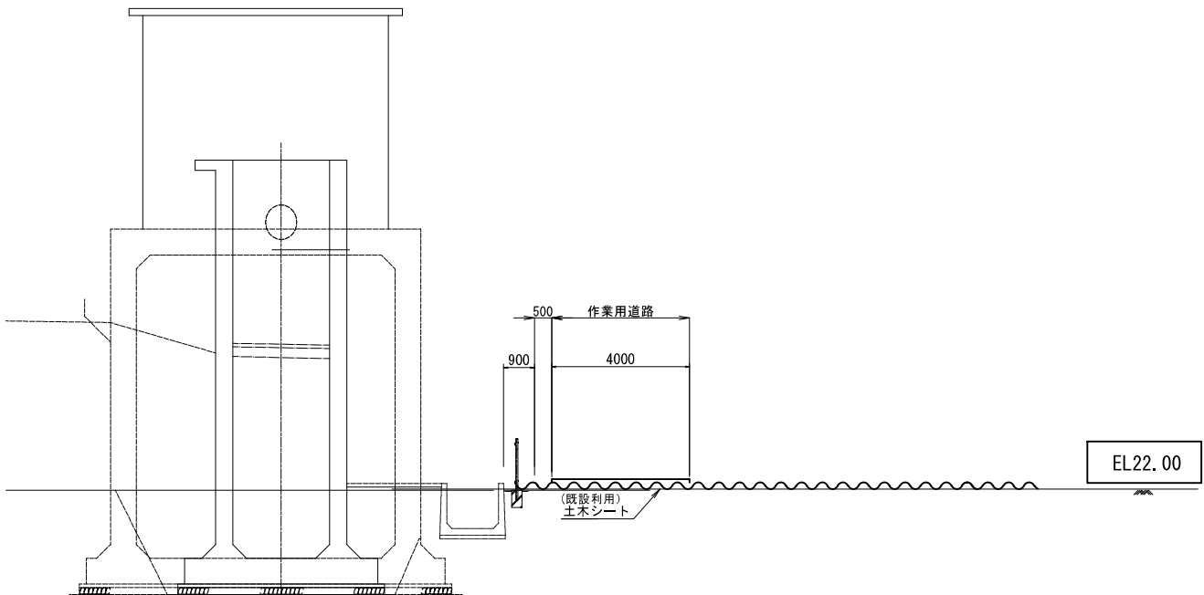
B-B
