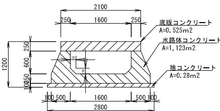
土工図
