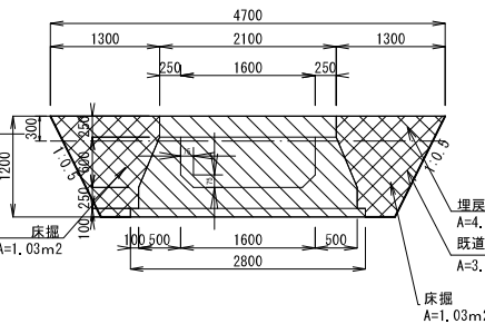
土工図
