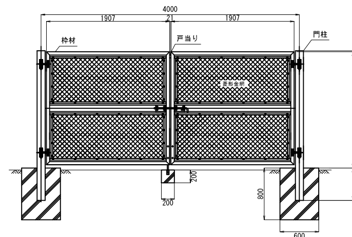
門扉正面図
