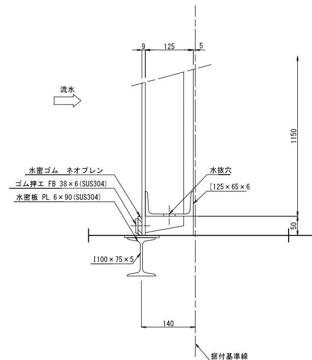
下部水密詳細
