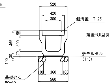
落蓋式側溝
