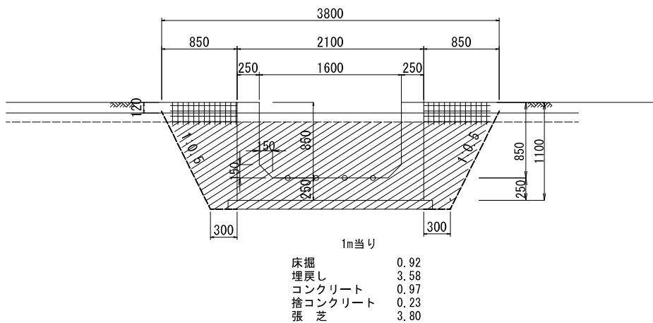
3-3 断面
