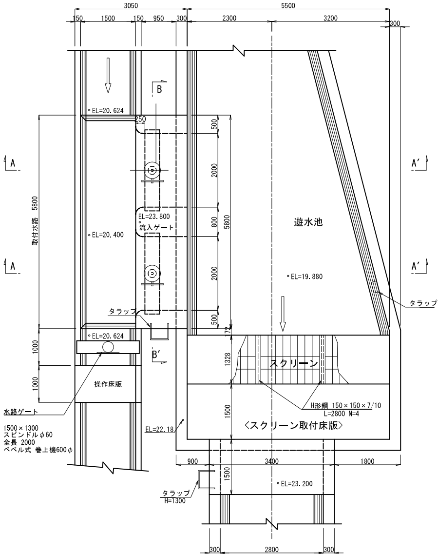
平面図
