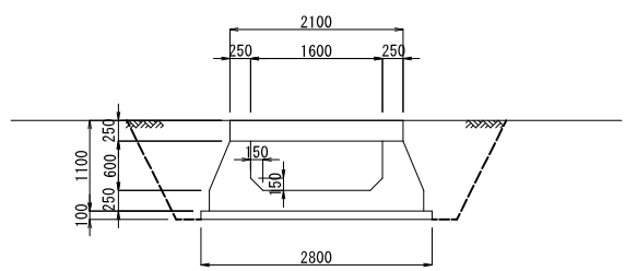
(暗渠工) B~B' 断面
