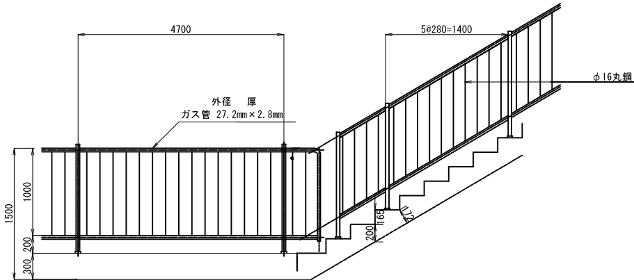
ポンプ揚水路手すり
