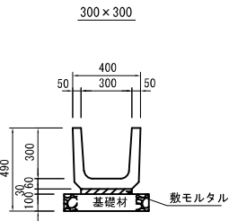
既設U型側溝標準図
