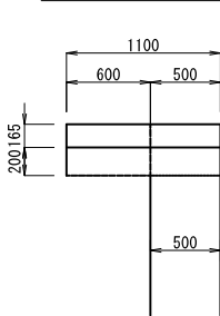
A-A' 断面図
