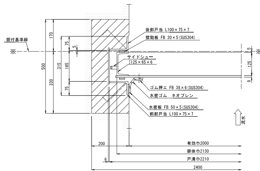
側部水密詳細
