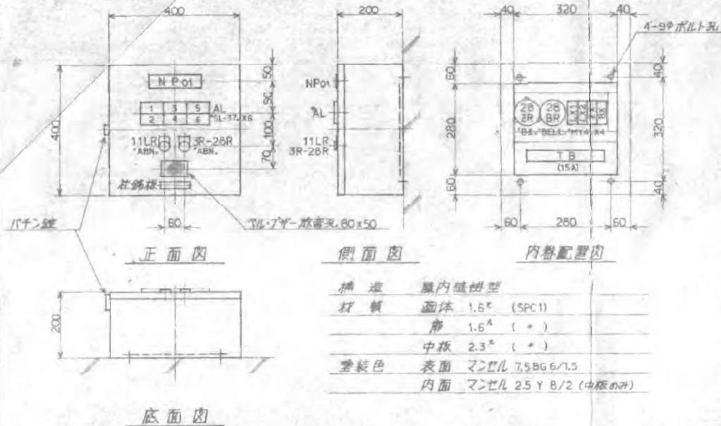
警報表示盤 1:10
