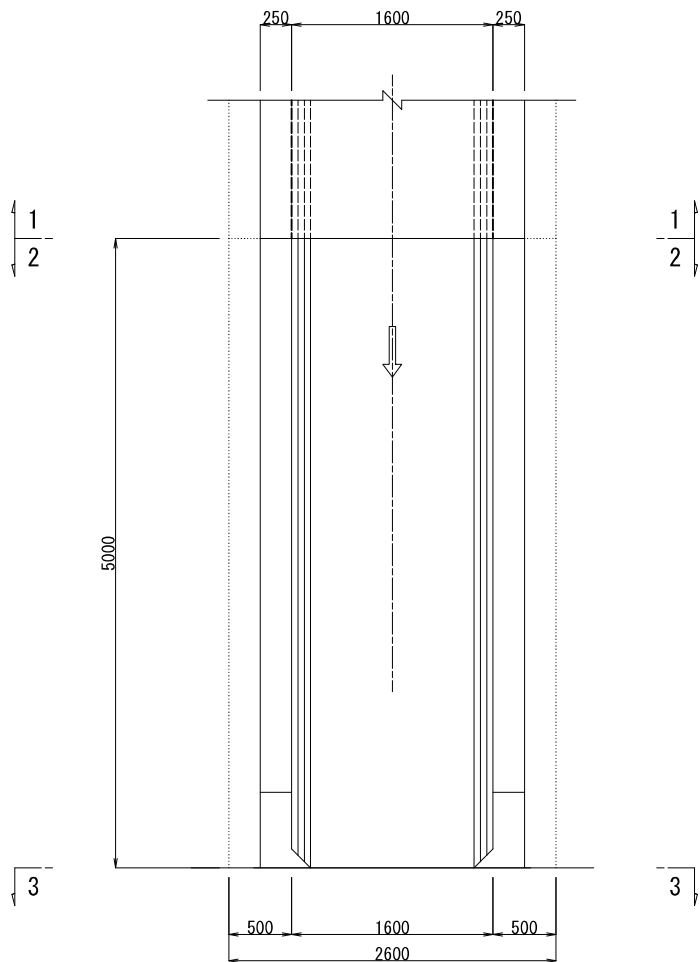
平面図
