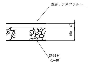
舗装断面図
