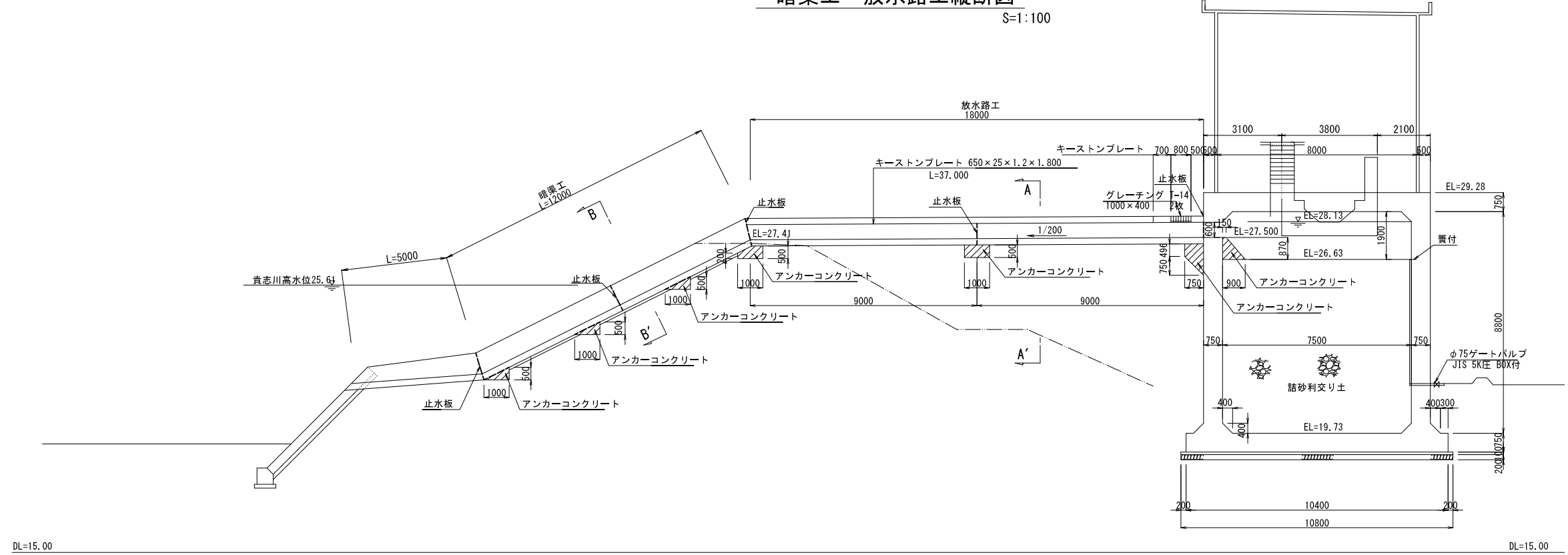
暗渠工・放水路工縦断面図
