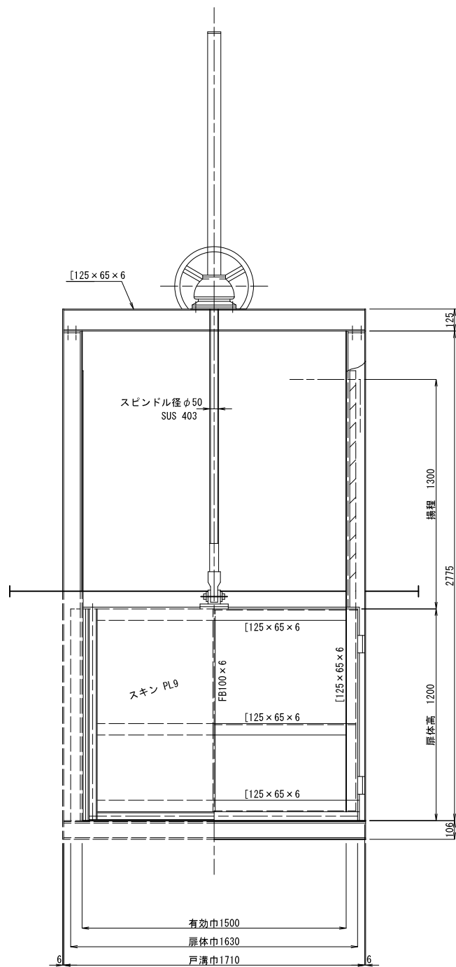
正面図
