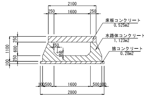
(放水路工) A~A' 断面
