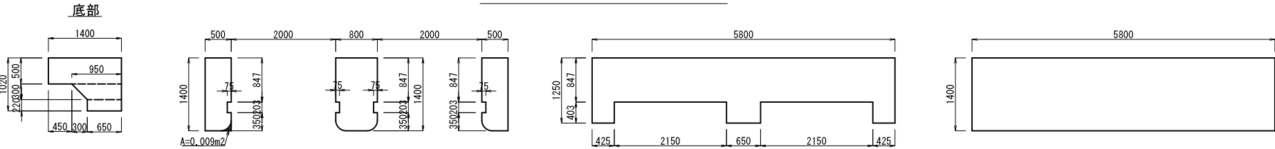
流入部ゲート取付工
