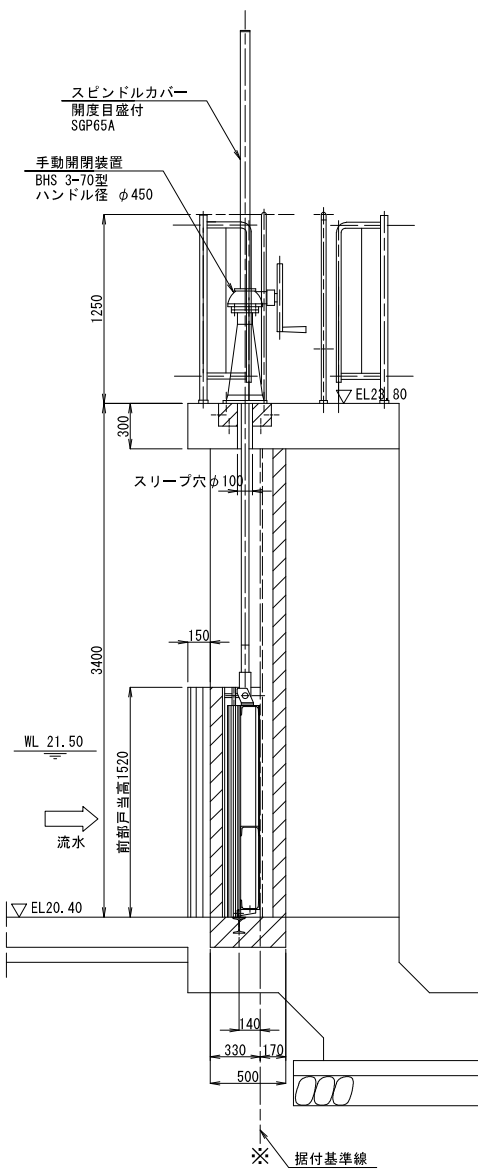
側面図
