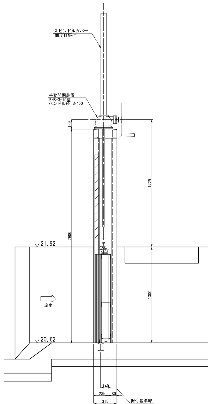
側面図
