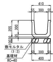
側溝U型
