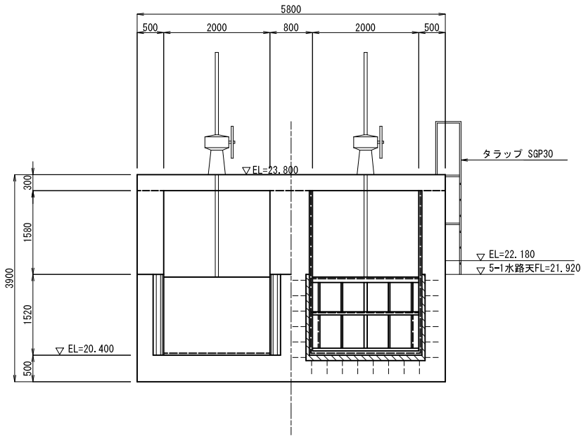
B-B' 断面
