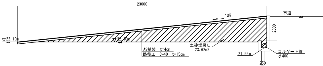
工事用進入路 標準断面図
