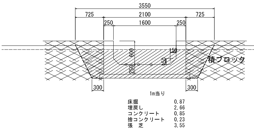
3-3 断面
