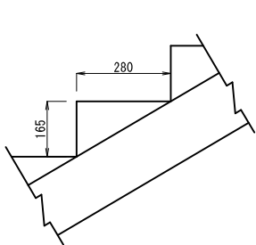
階段工詳細図
