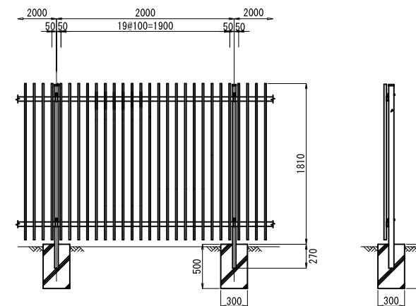
フェンス正面図・側面図
