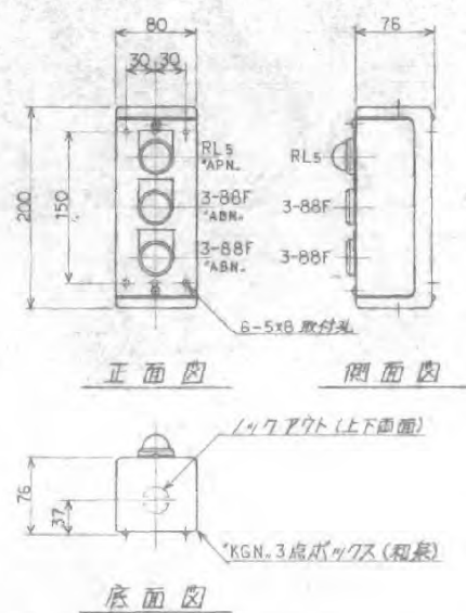
燃料移送ポンプ現場操作盤 1:5
