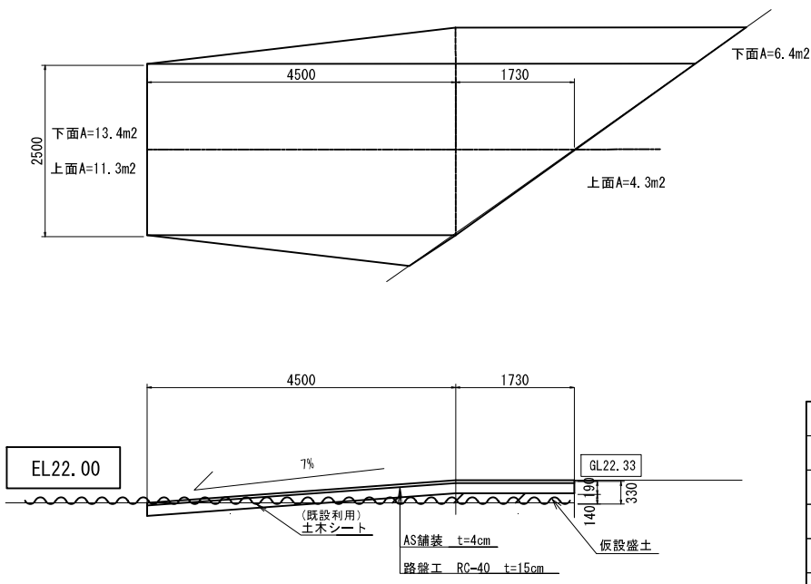
A-A (工事用進入路)
