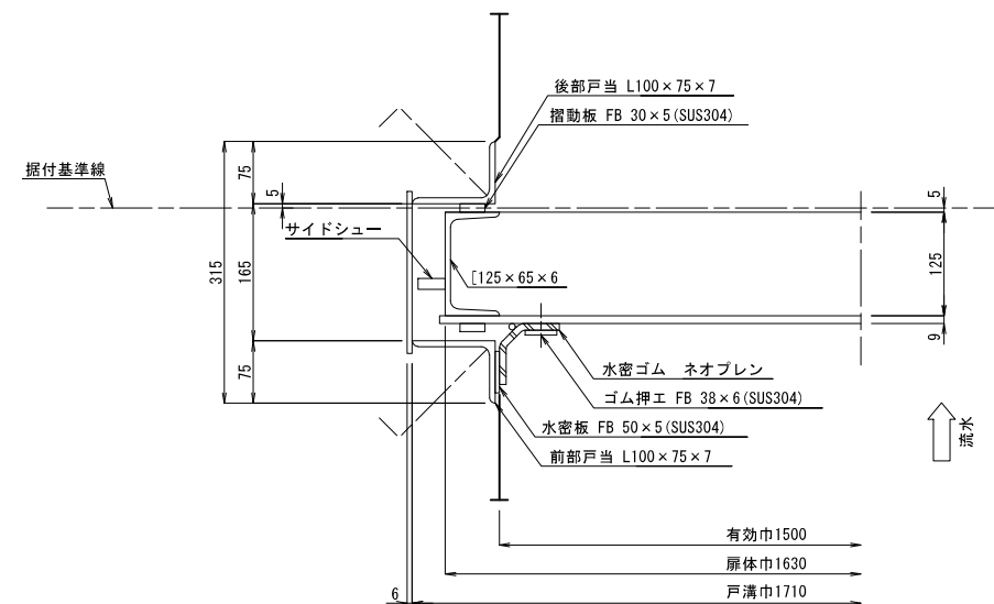
側部水密詳細
