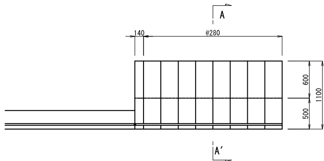
ポンプ揚水路階段工
