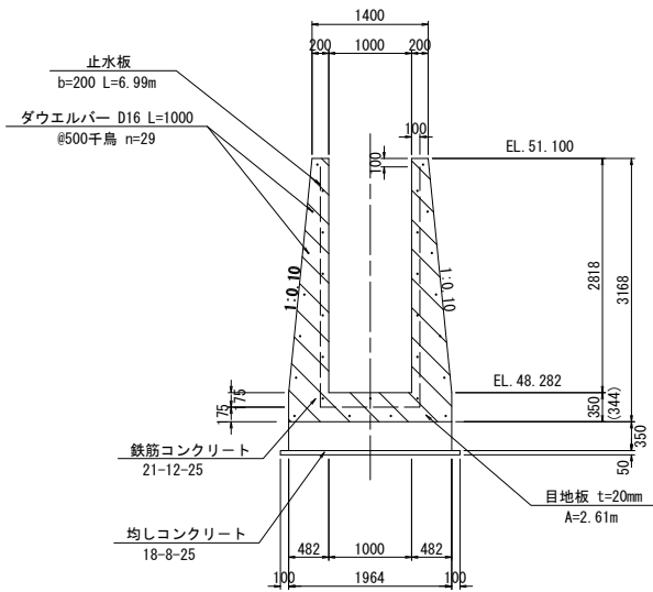
D-D断面 S=1:50
