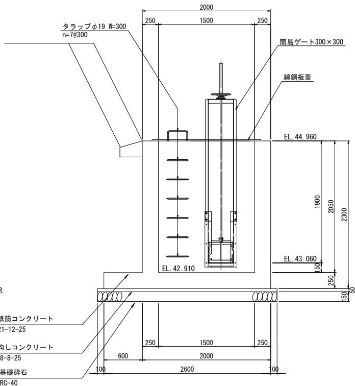
E-E断面
