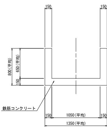
洪水吐2
