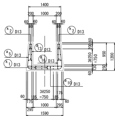
C-C 断面
