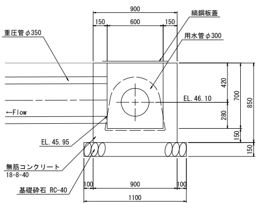
B-B断面
