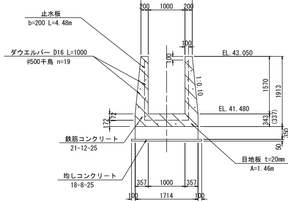
I-I断面 S=1:50
