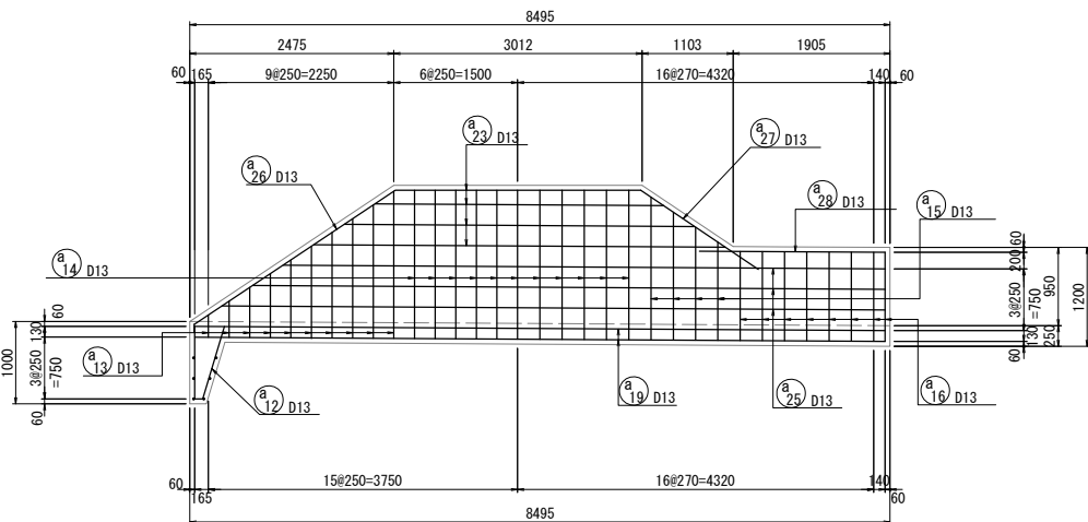
右岸側壁外面
