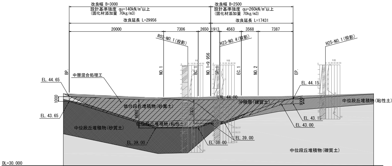
縦断図 S=1:250
