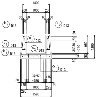
A-A 断面
