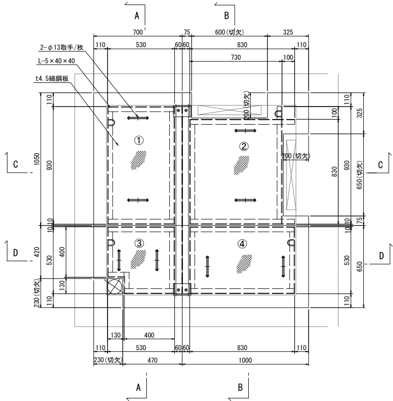
平面図 S=1:15
