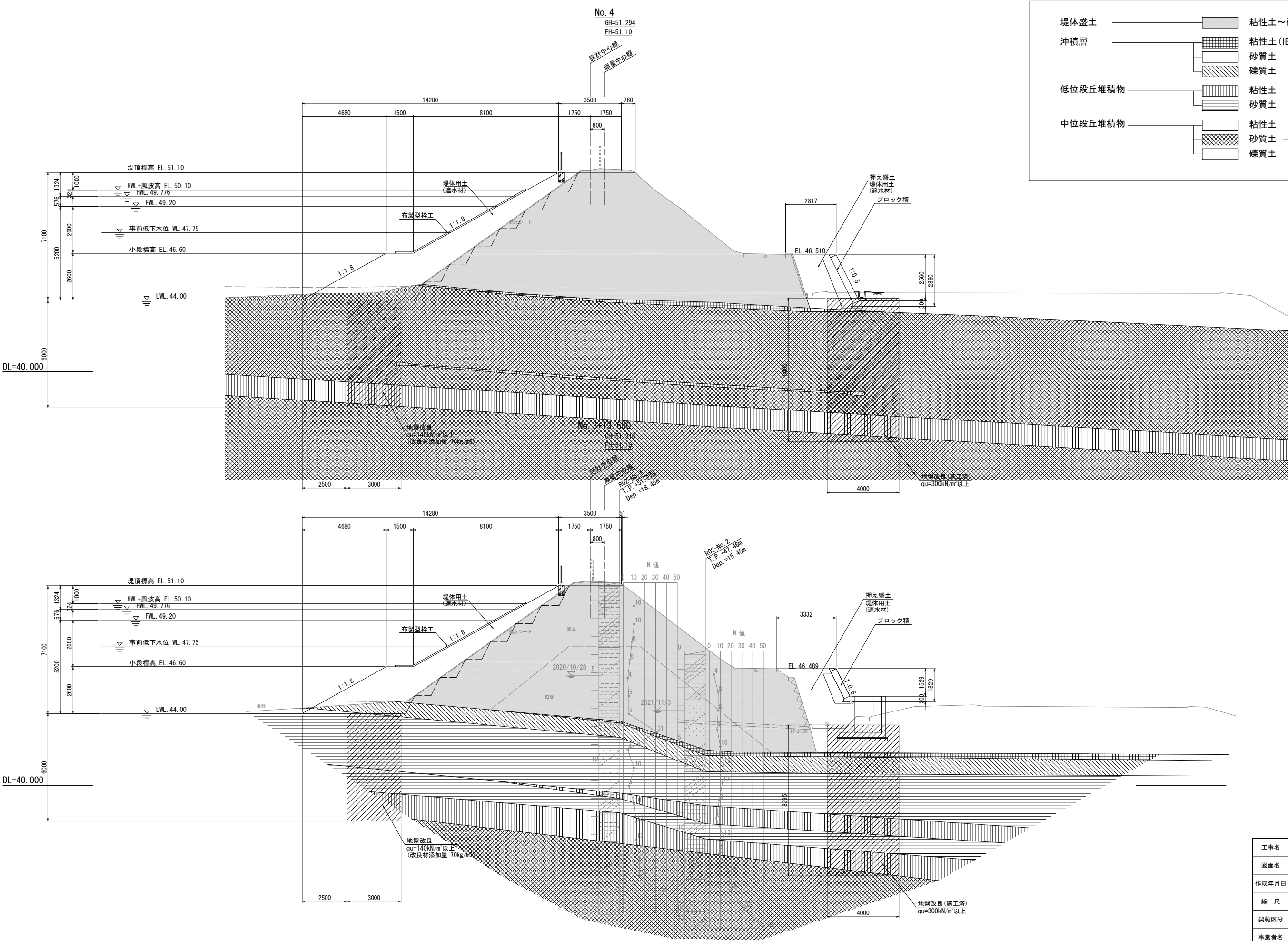
花ヤ池 堤体工横断図(4) S=1:100
