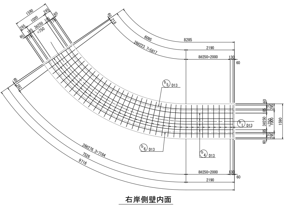
底版下面
