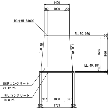
B-B断面
