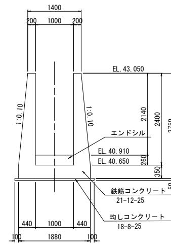
L-L断面 S=1:50
