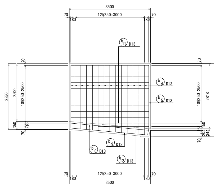
側壁内面
