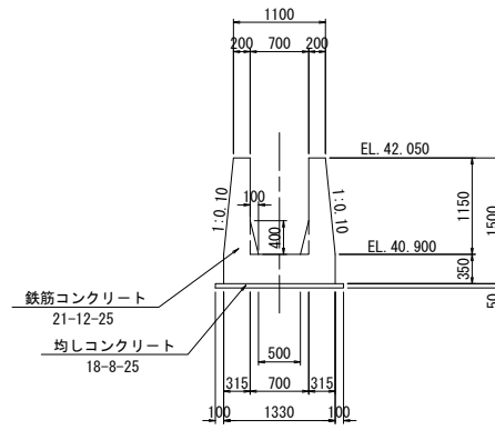
止水壁構造図 S=1:50
