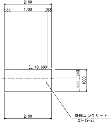
A-A断面 S=1:50
