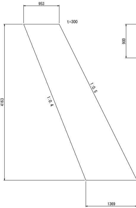
4号小口止工
