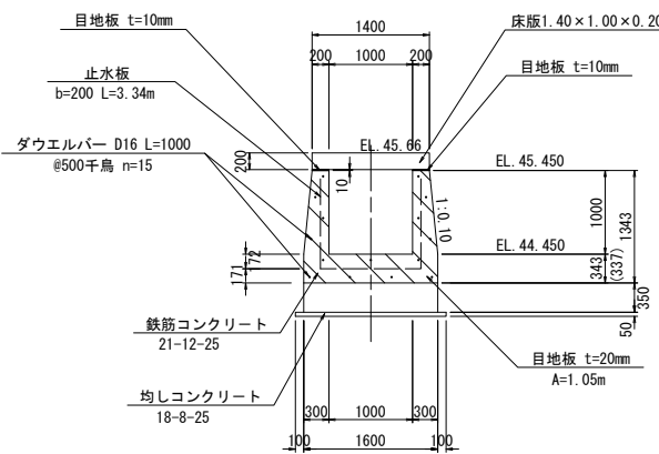
F-F断面 S=1:50
