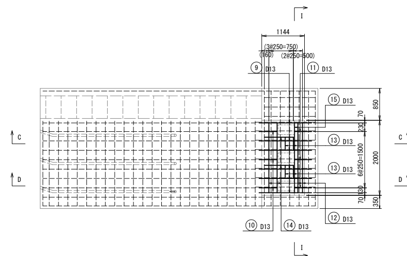
巻上機部平面図
