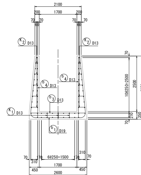
B-B 断面
