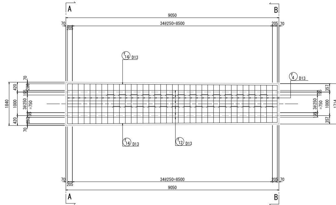
底版上面
