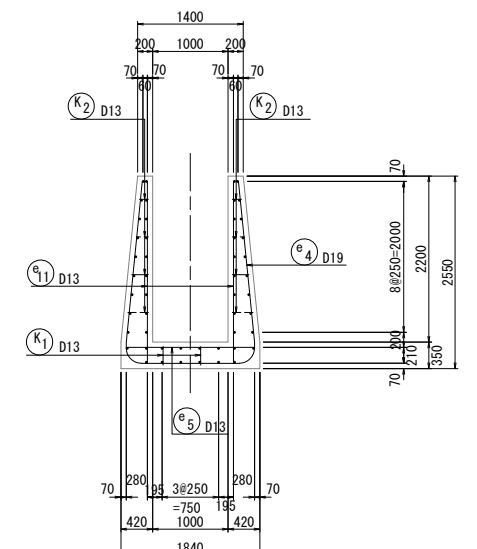
B-B 断面
