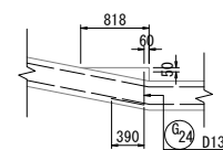
a-a断面
