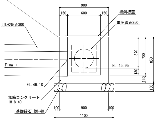
B-B断面
