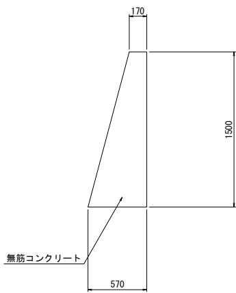
土留1・2
