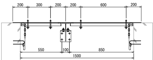
D-D断面 S=1:15
