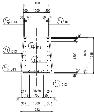
B-B 断面
