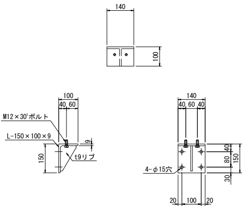
ブラケット詳細図 S=1:10
