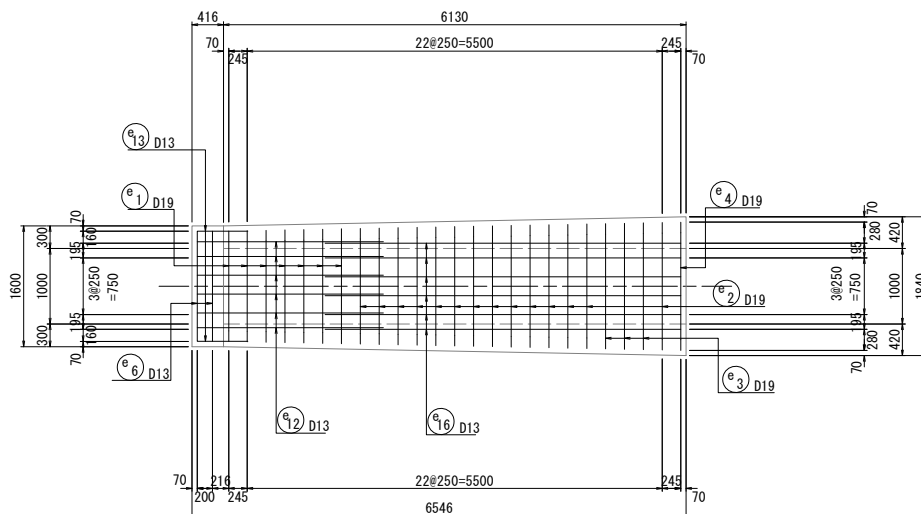
底版下面
