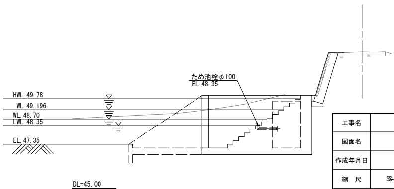
C-C断面
