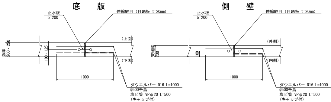
継目工詳細図
