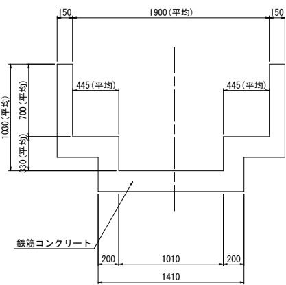
洪水吐1
