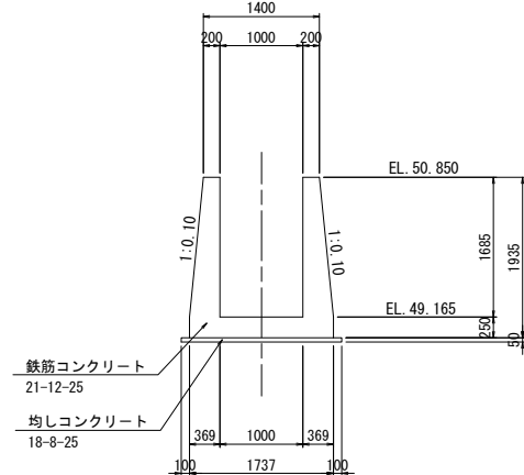
C-C断面
