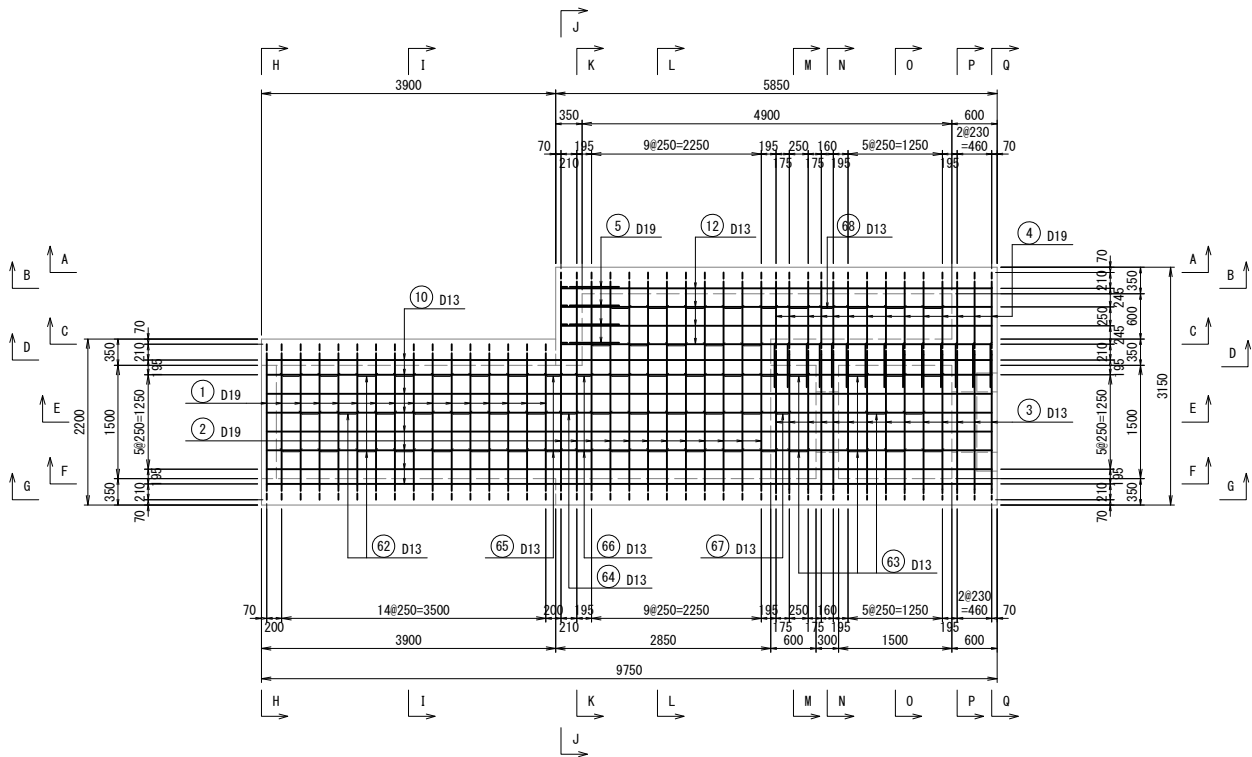
底板下面
