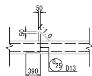
b-b断面
