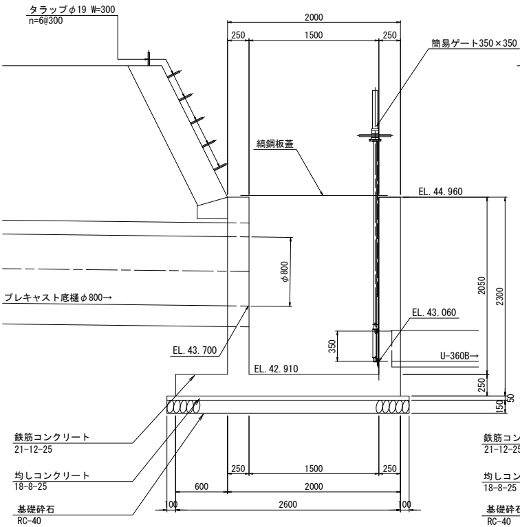
A-A断面
