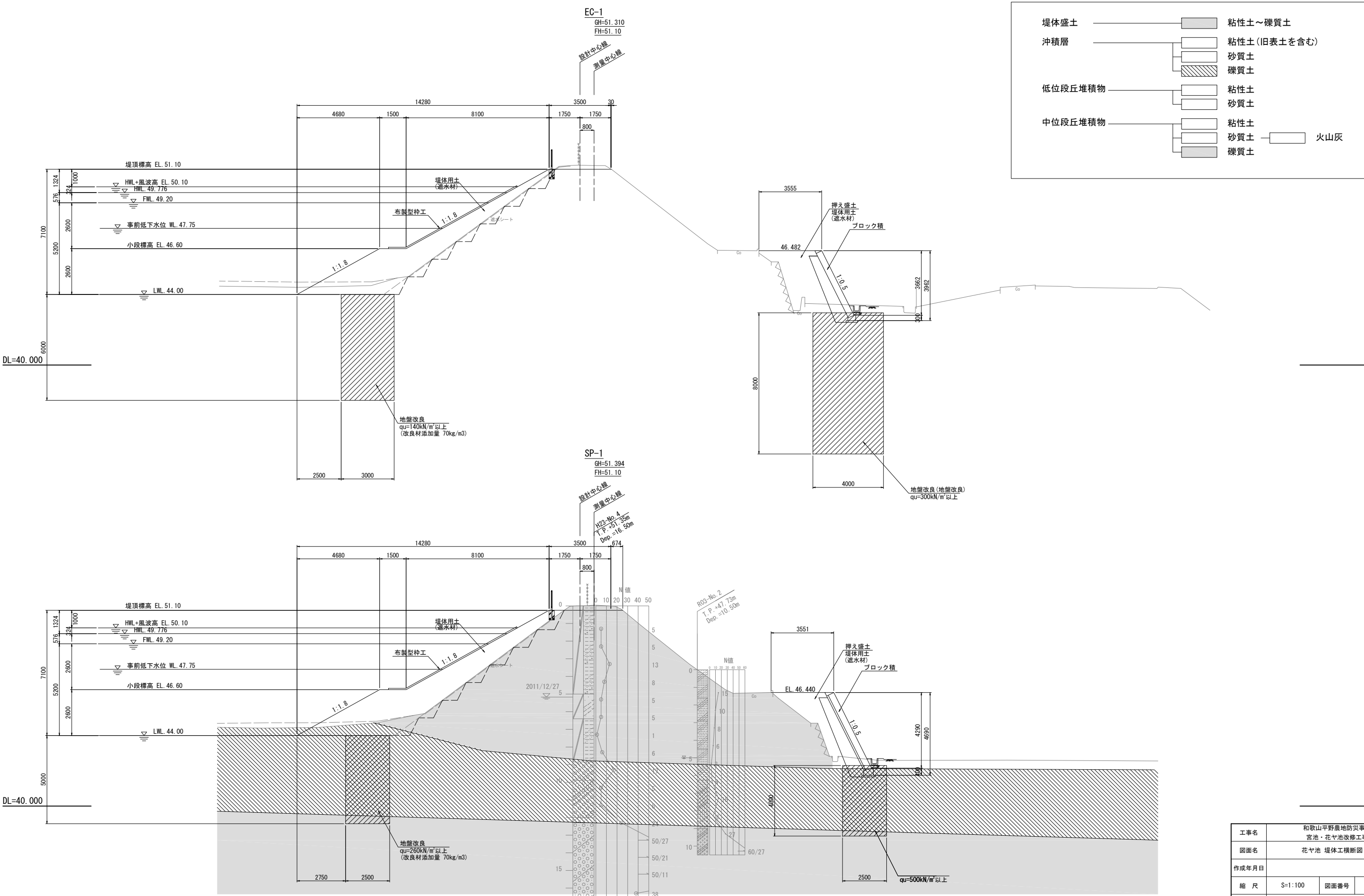
花ヤ池 堤体工横断図(3) S=1:100
