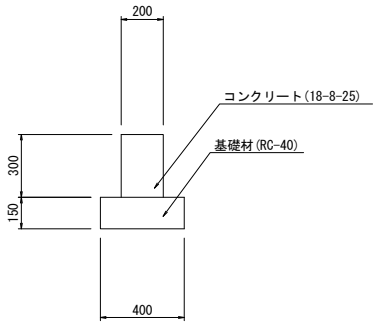
天端工詳細図
