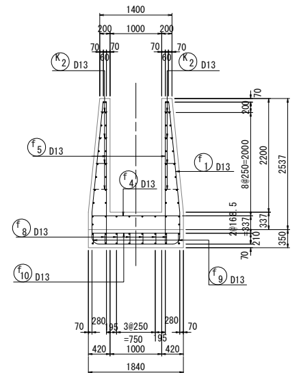
B-B 断面
