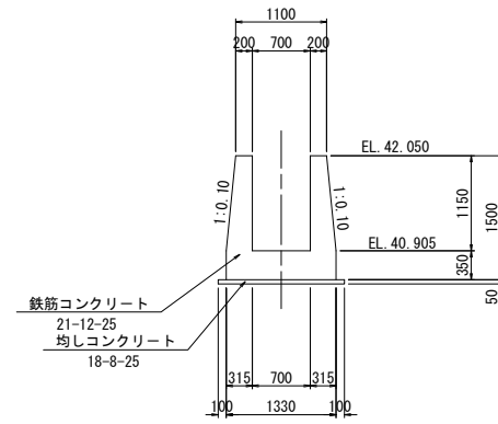
K-K断面 S=1:50
