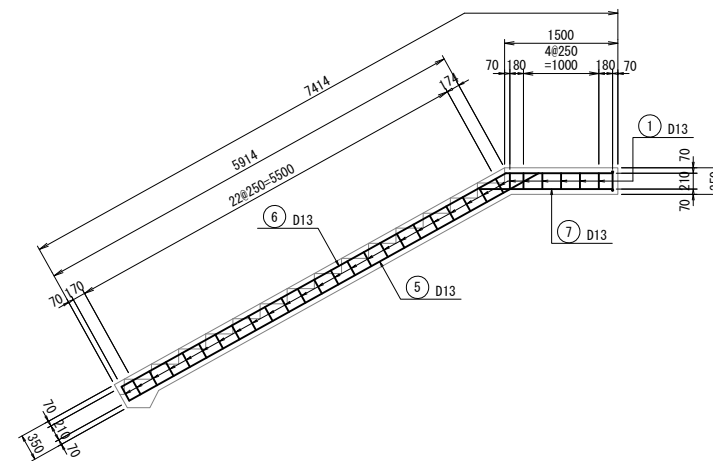
B - B
