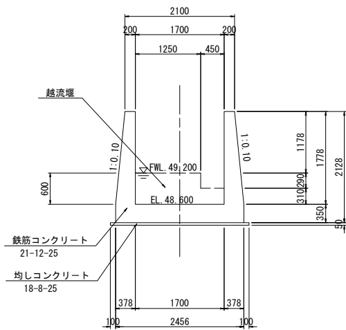
B-B断面 S=1:50
