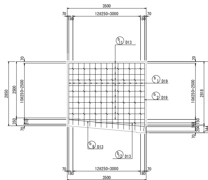
側壁外面
