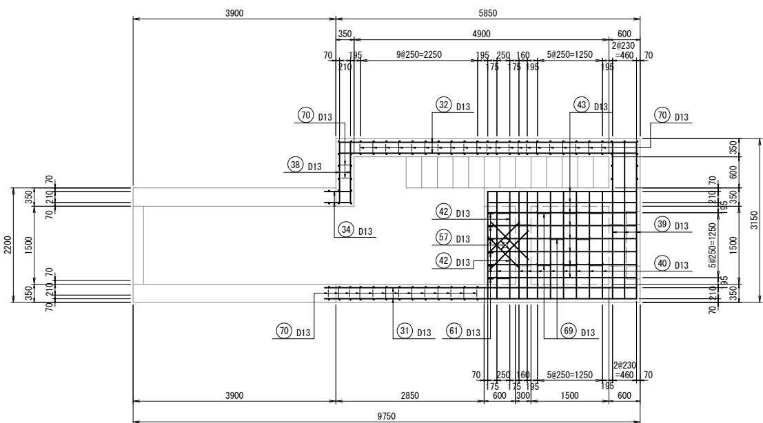
頂版下面
