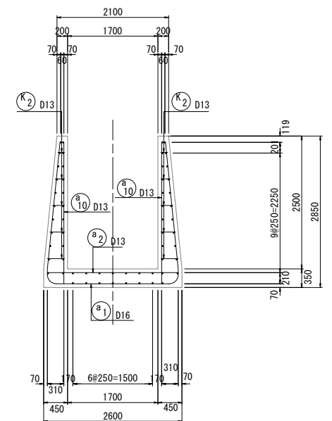
C-C 断面
