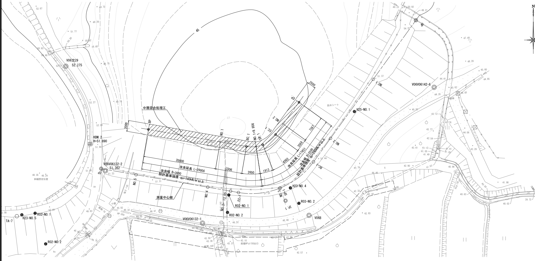
平面図 S=1:250
