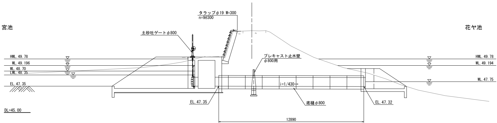
B-B断面
