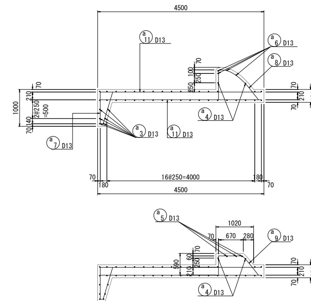
A-A 断面
