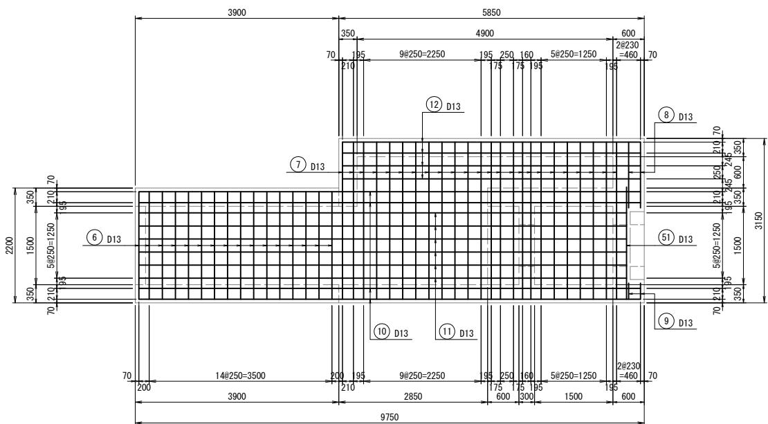
底板上面
