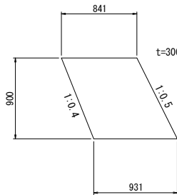
5号小口止工
