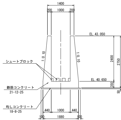
I-I断面 S=1:50
