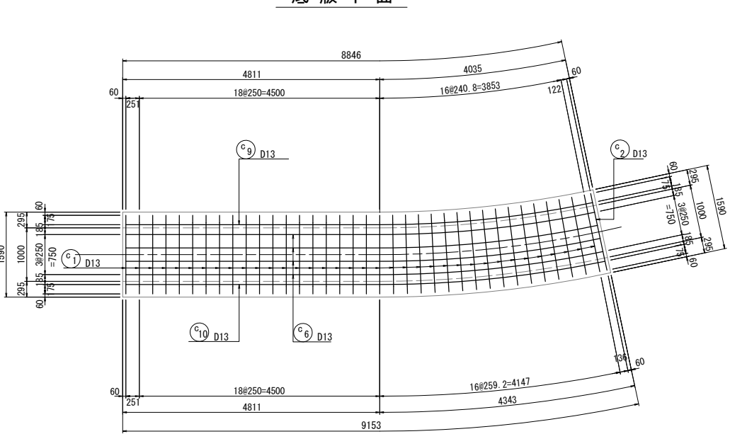
底板下面
