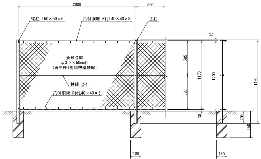
転落防止柵・門扉 S=1:30
