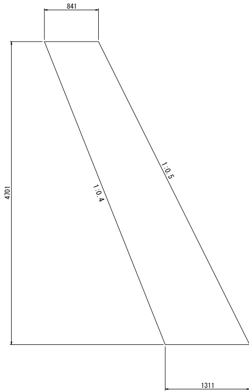
3号小口止工
