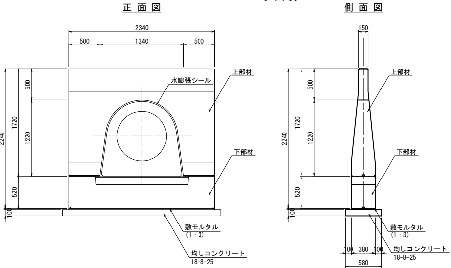
止水壁標準図 S=1 : 30
