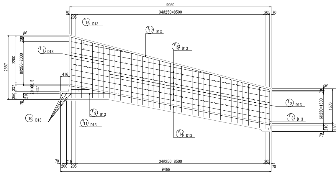
側壁内面
