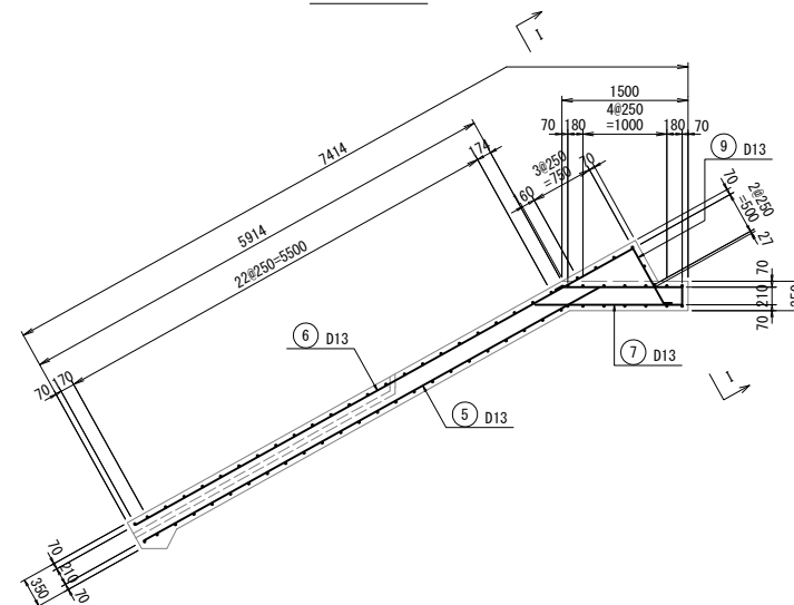
C - C
