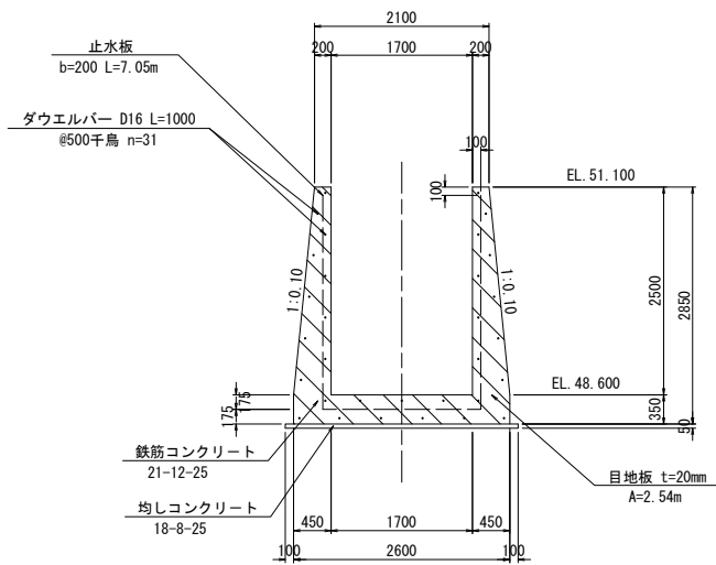
C-C断面 S=1:50
