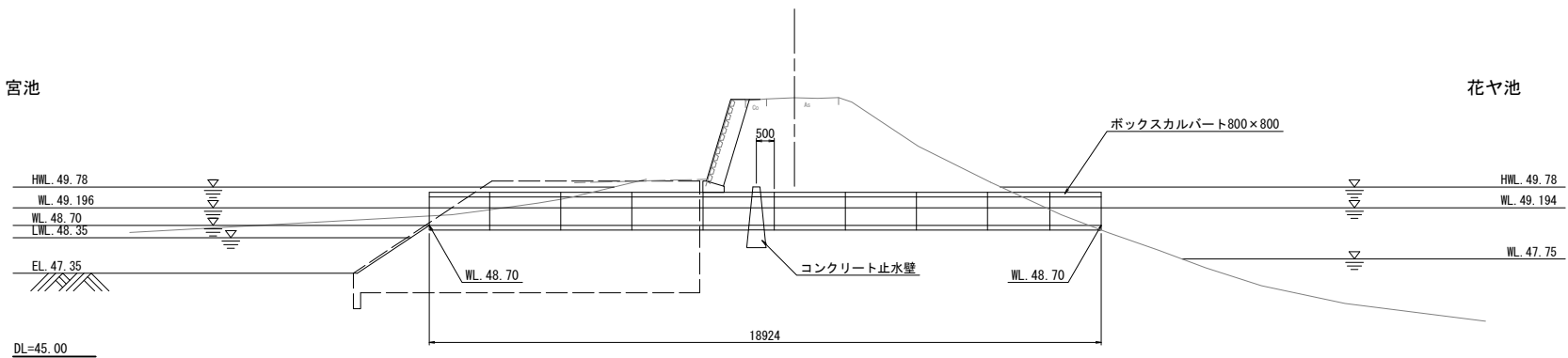
B-B断面
