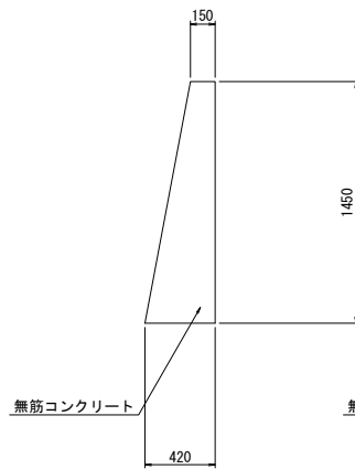
土留1・2
