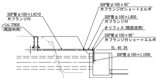
縦断面図
