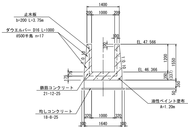
F-F断面 S=1:50
