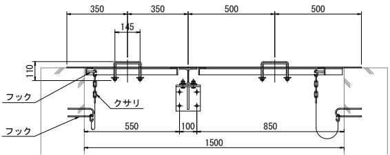
C-C断面 S=1:15
