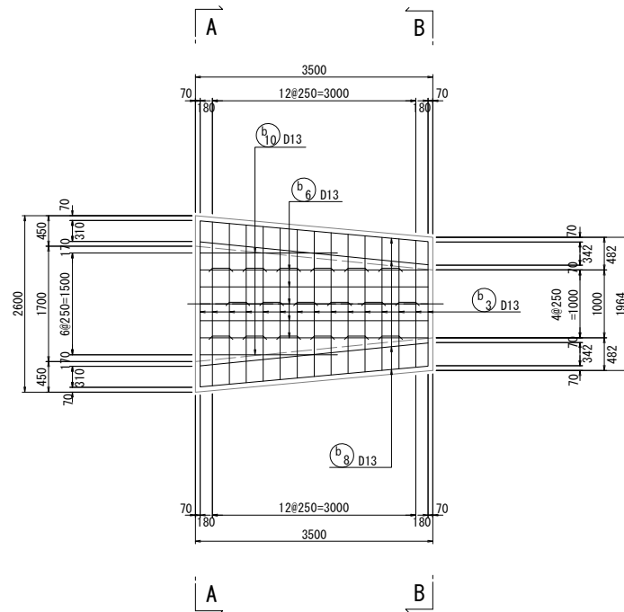
底版上面
