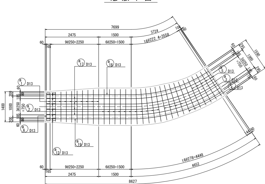
底版下面
