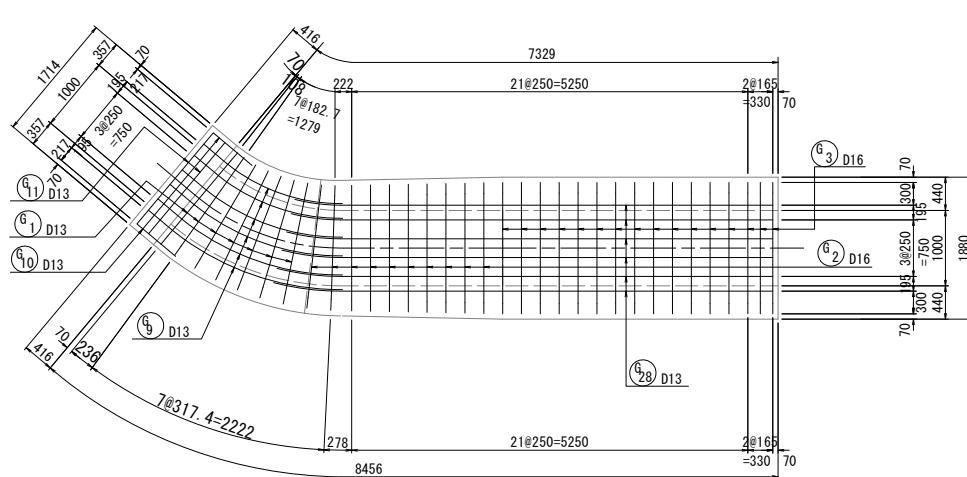
底版下面
