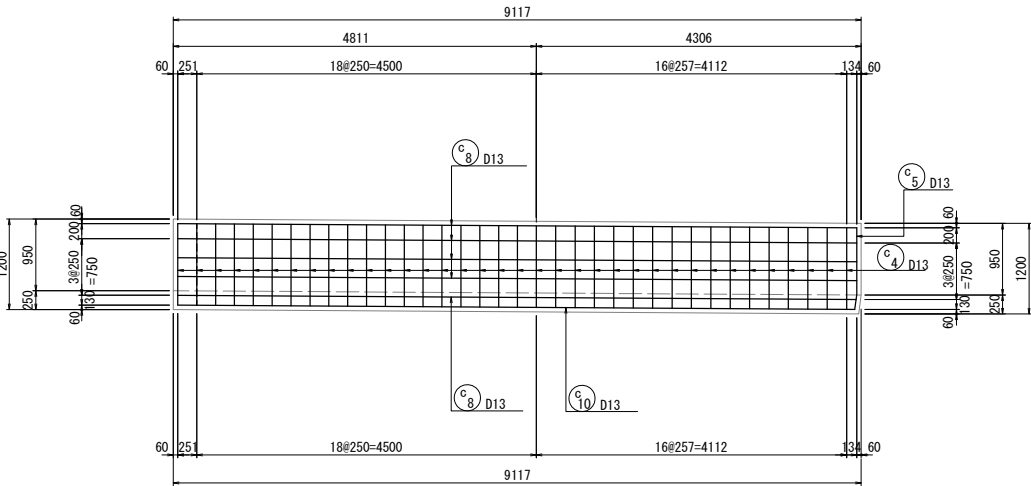
右岸側壁外面
