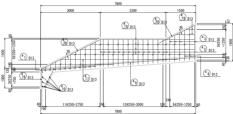
右側壁(外側)
