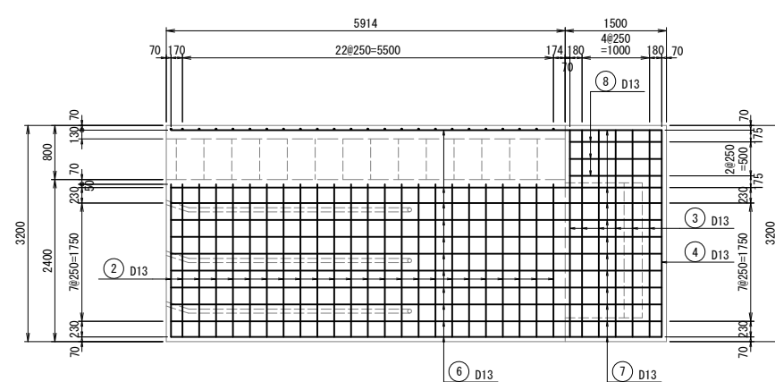
底板上面
