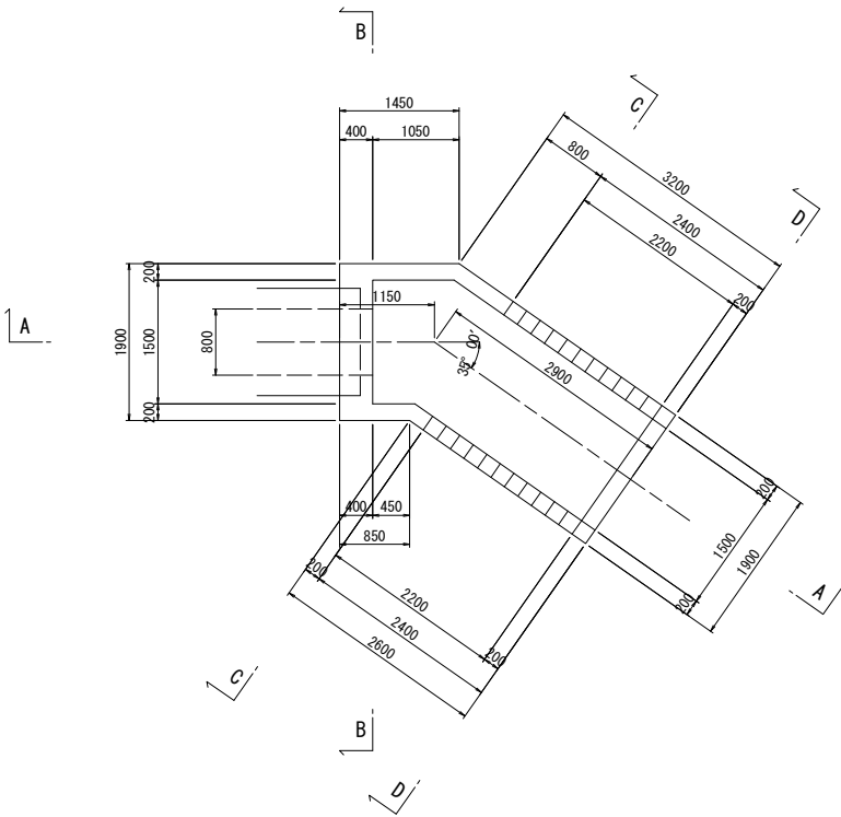
平面図
