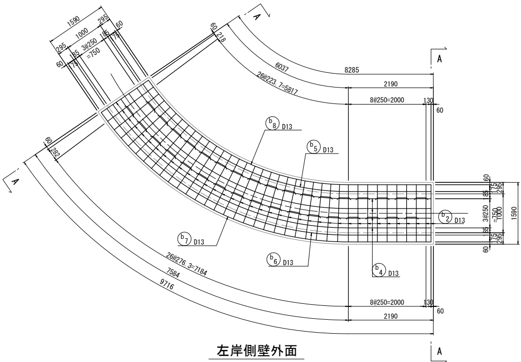
底版上面
