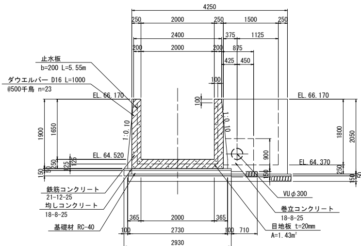
D-D断面
