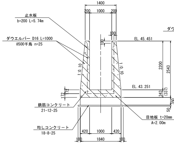
H-H断面 S=1:50
