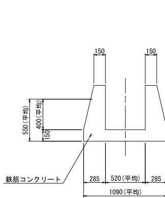
洪水吐3
