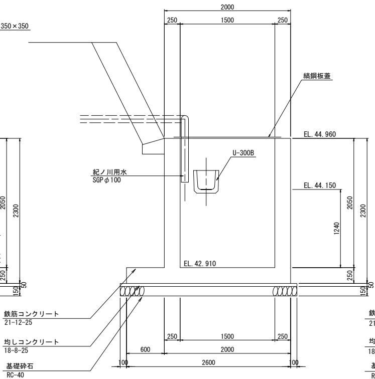
D-D断面
