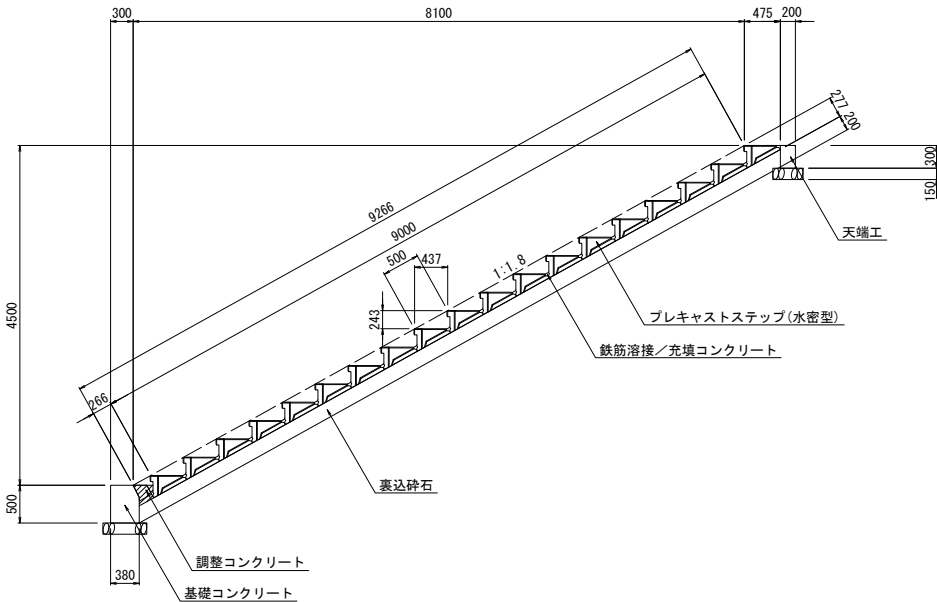
断面図 S=1:50
