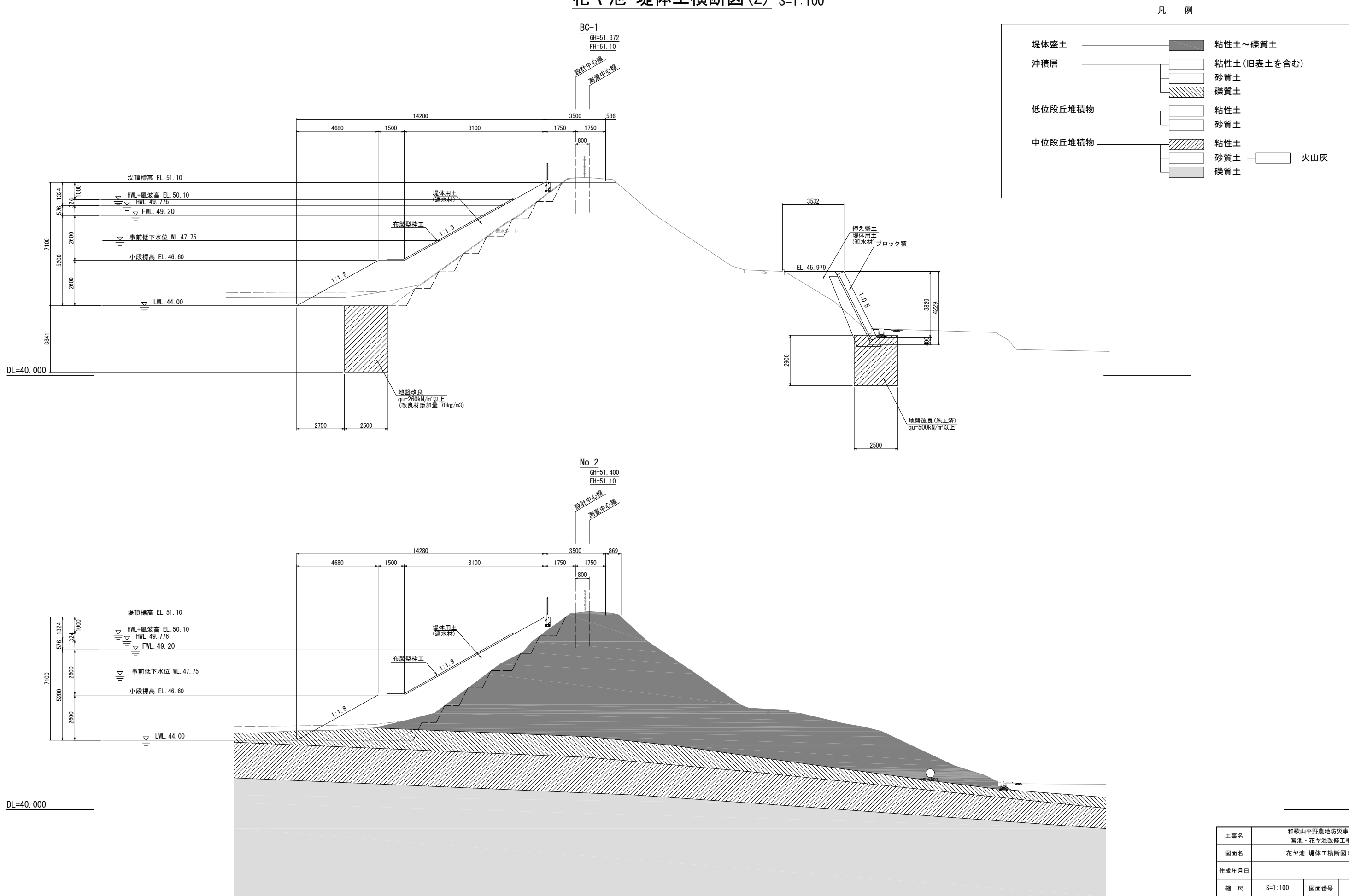
花ヤ池 堤体工横断図(2) S=1:100
