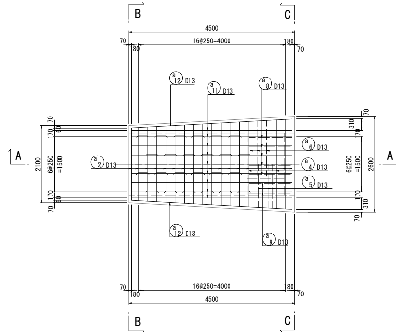
底板上面
