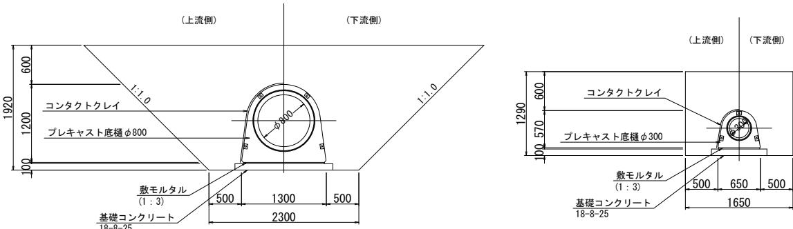
底樋管φ800
