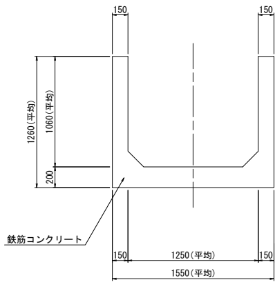
洪水吐1
