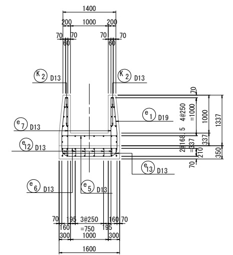
B-B 断面
