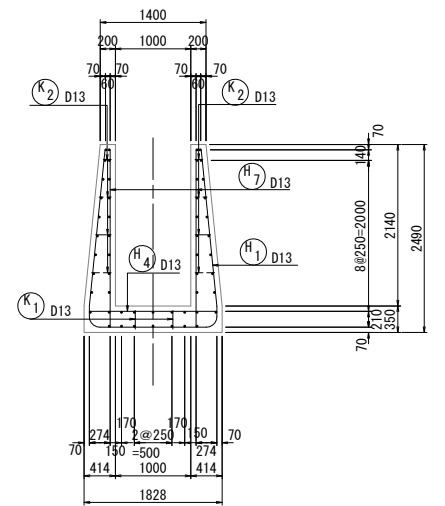
B-B 断面
