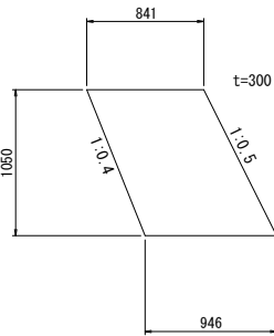
1号小口止工
