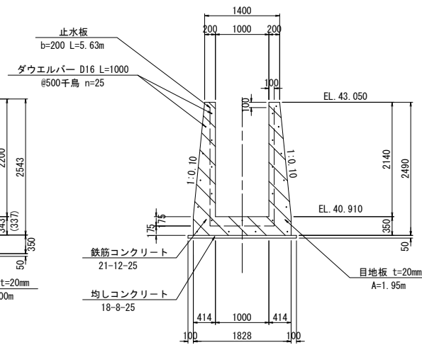
K-K断面 S=1:50
