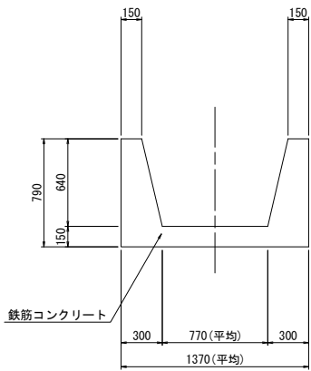
洪水吐2
