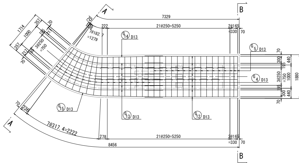
底版上面
