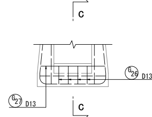
c-c断面
