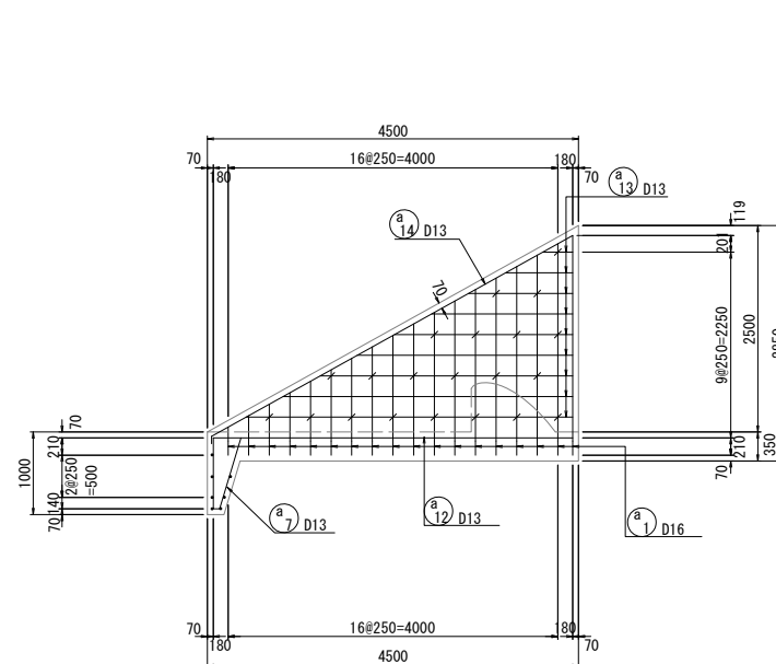
側壁外面
