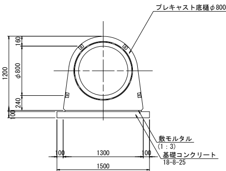
底樋管φ800
