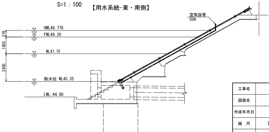
C-C断面
