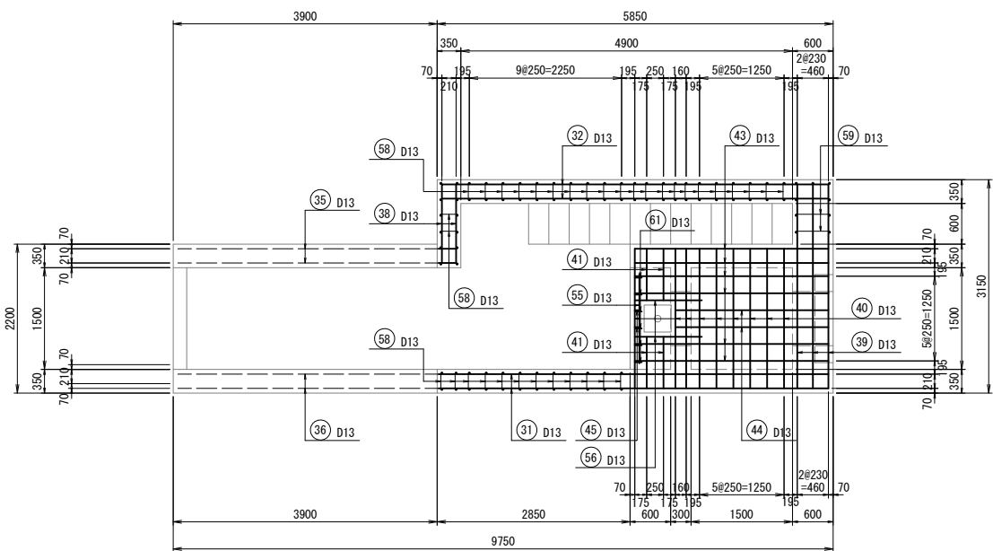
頂版上面
