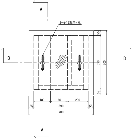
B-B
