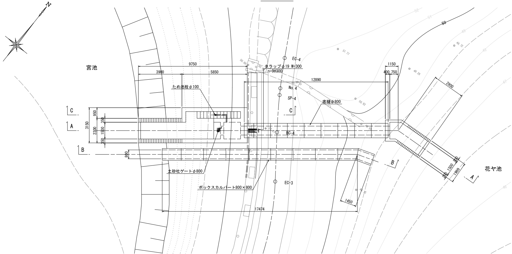
平面図
