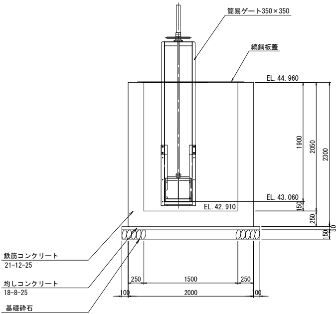
C-C断面
