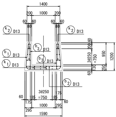
A-A 断面
