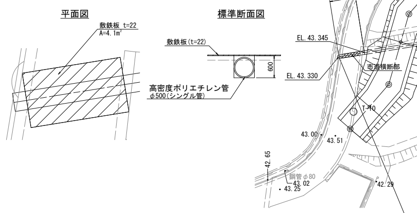
市道横断面詳細図 S=1:50
