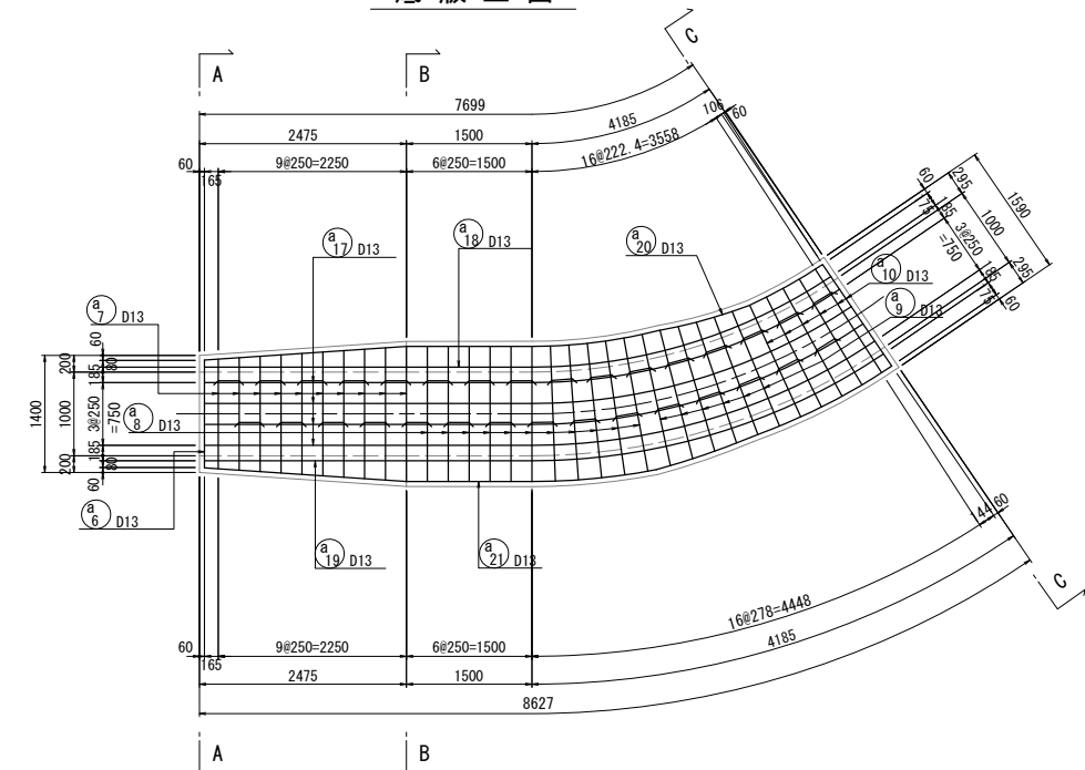
左岸側壁外面
