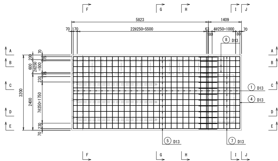
底板下面
