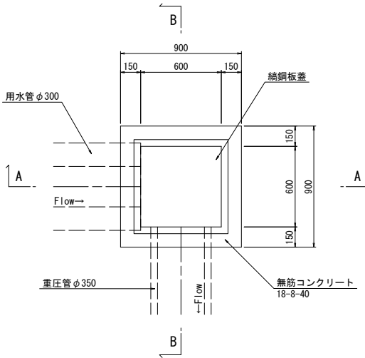
A-A断面
