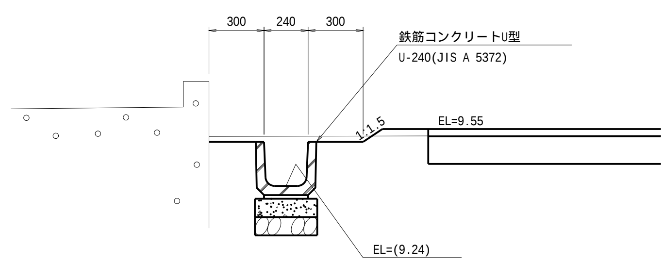
A-A断面 S=1/20
