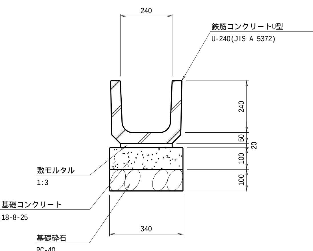
鉄筋コンクリートU型 U-240 S=1/10
