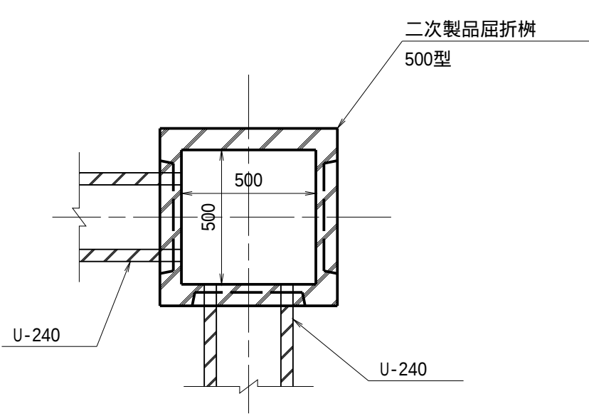
屈折樹 (500型) S=1/20
