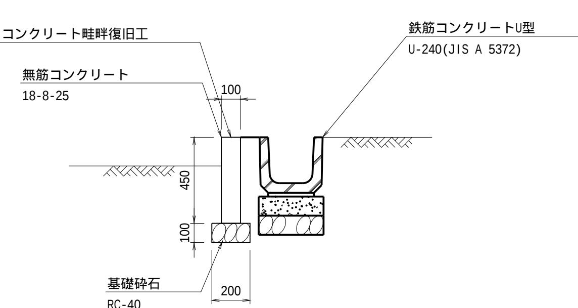
B-B断面 S=1/20
