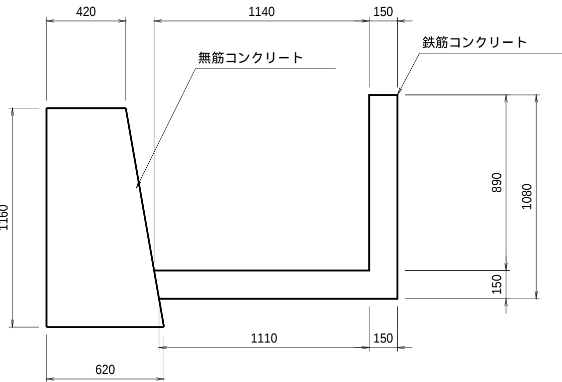
水路取壊工(岩橋支線水路)
