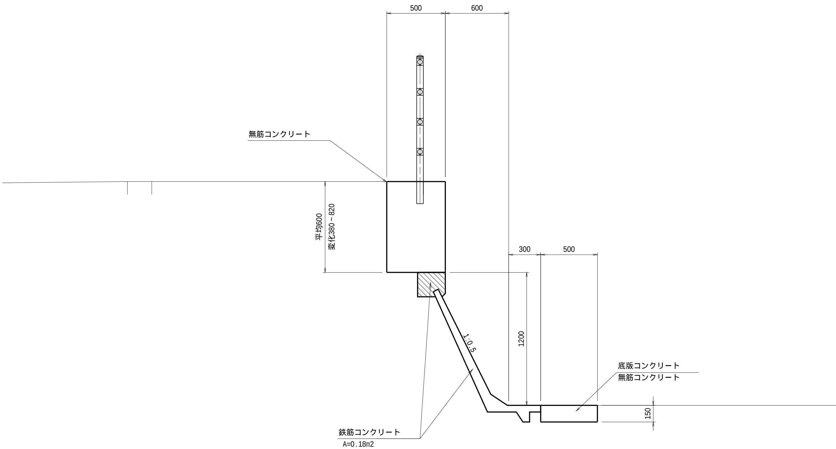
既設水路取壊工 Type b
