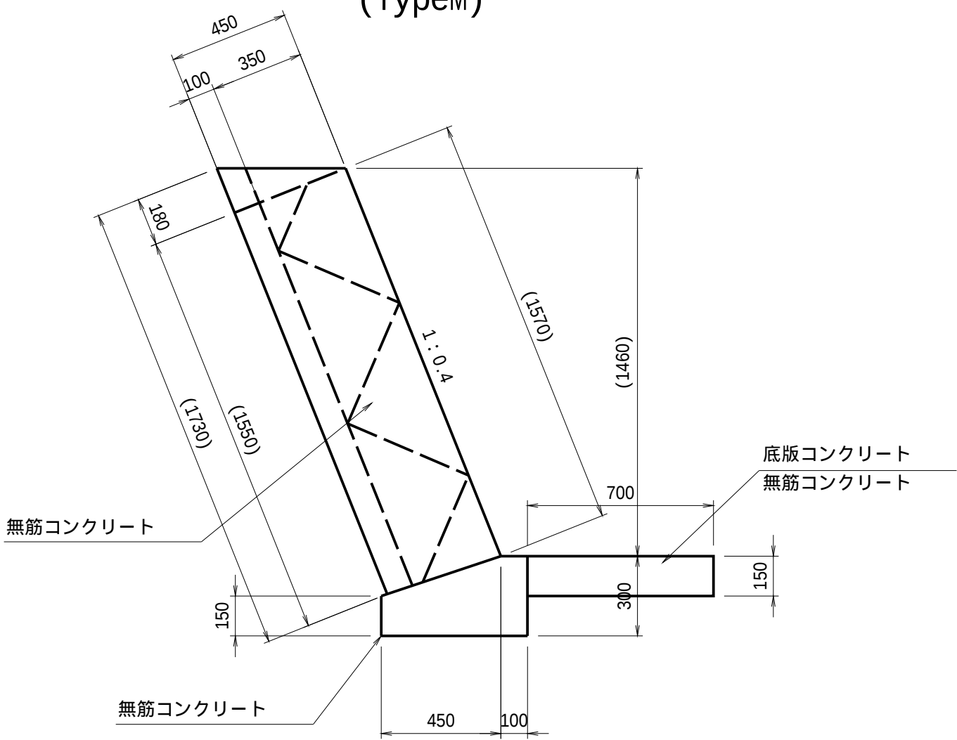
水路取壊工(宮井水路)(左岸)
