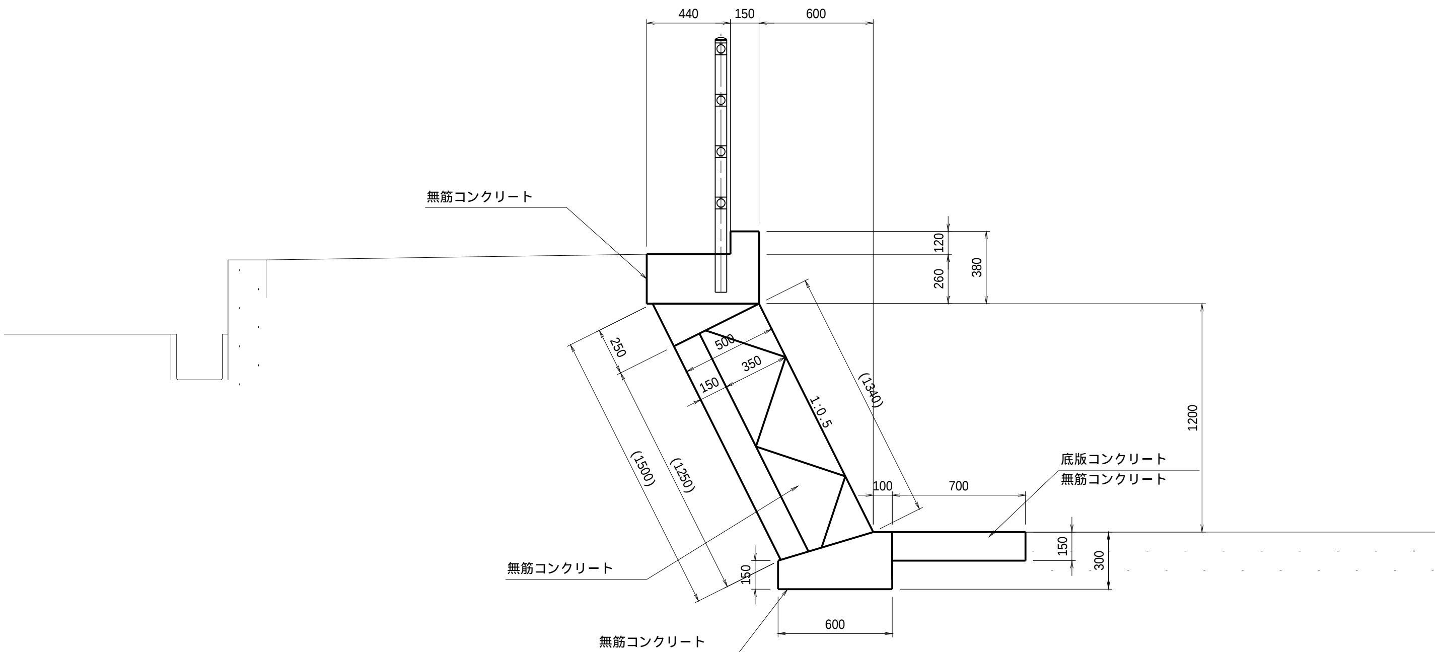
既設水路取壊工 Type a
