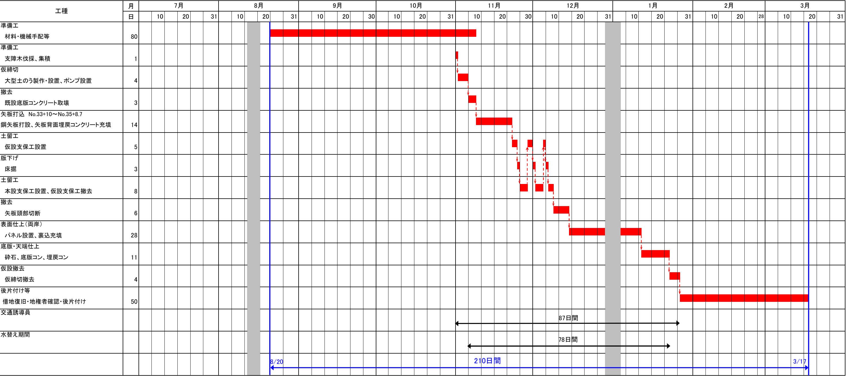
令和6年度 和歌山平野農地防災事業 名草排水路第3-2工区工事 工程表
