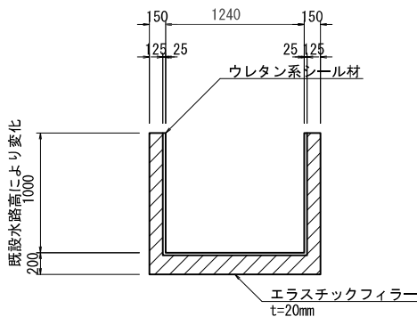
収縮継目断面図 S=1:30
