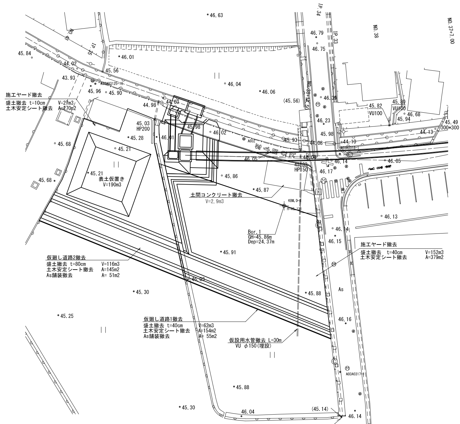
平面图 S=1:200
