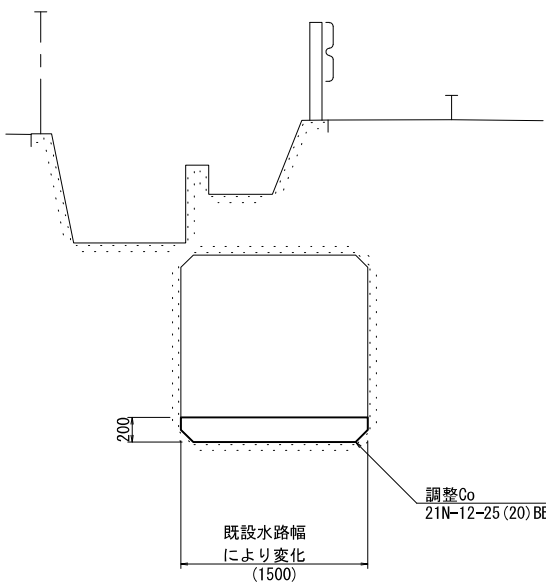
暗渠部 S=1:30
