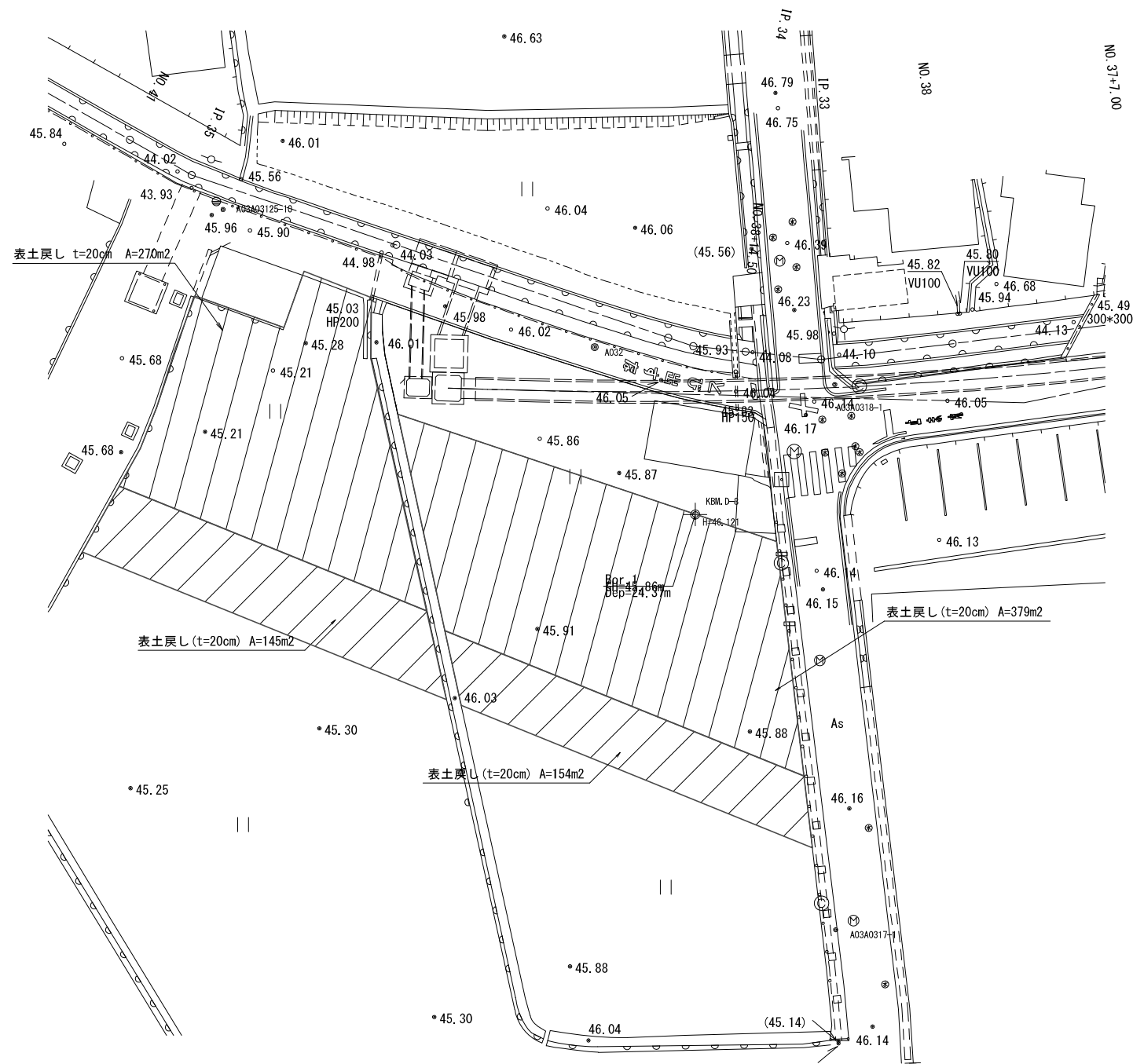
平面図
