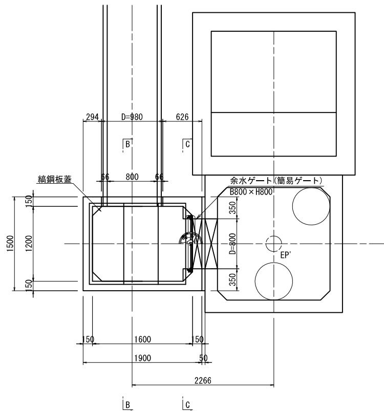
A-A平面図
