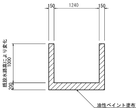
収縮継目断面図 S=1:30
