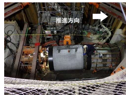
波分山崎排水路の推進工 (推進管：内径1,650mm)
