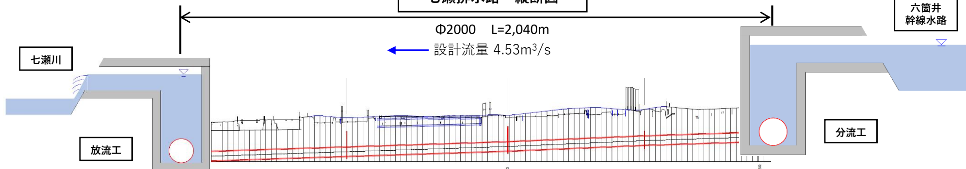
七瀬排水路 縦断面図
