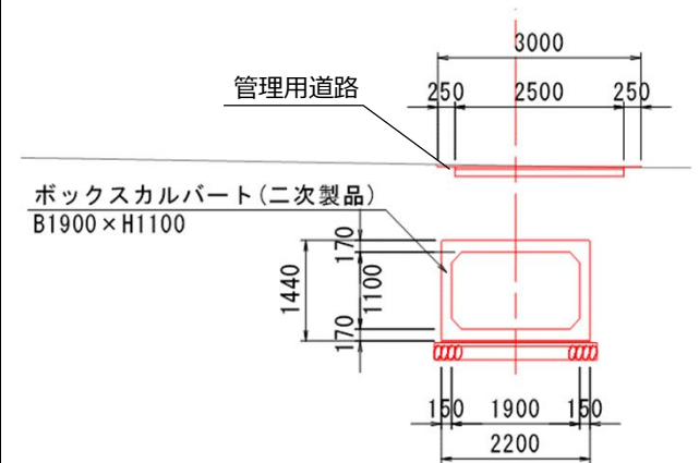
標準断面図 (小田井水路（烏子排水路）)
