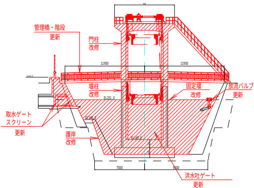
正面図 S=1:400
