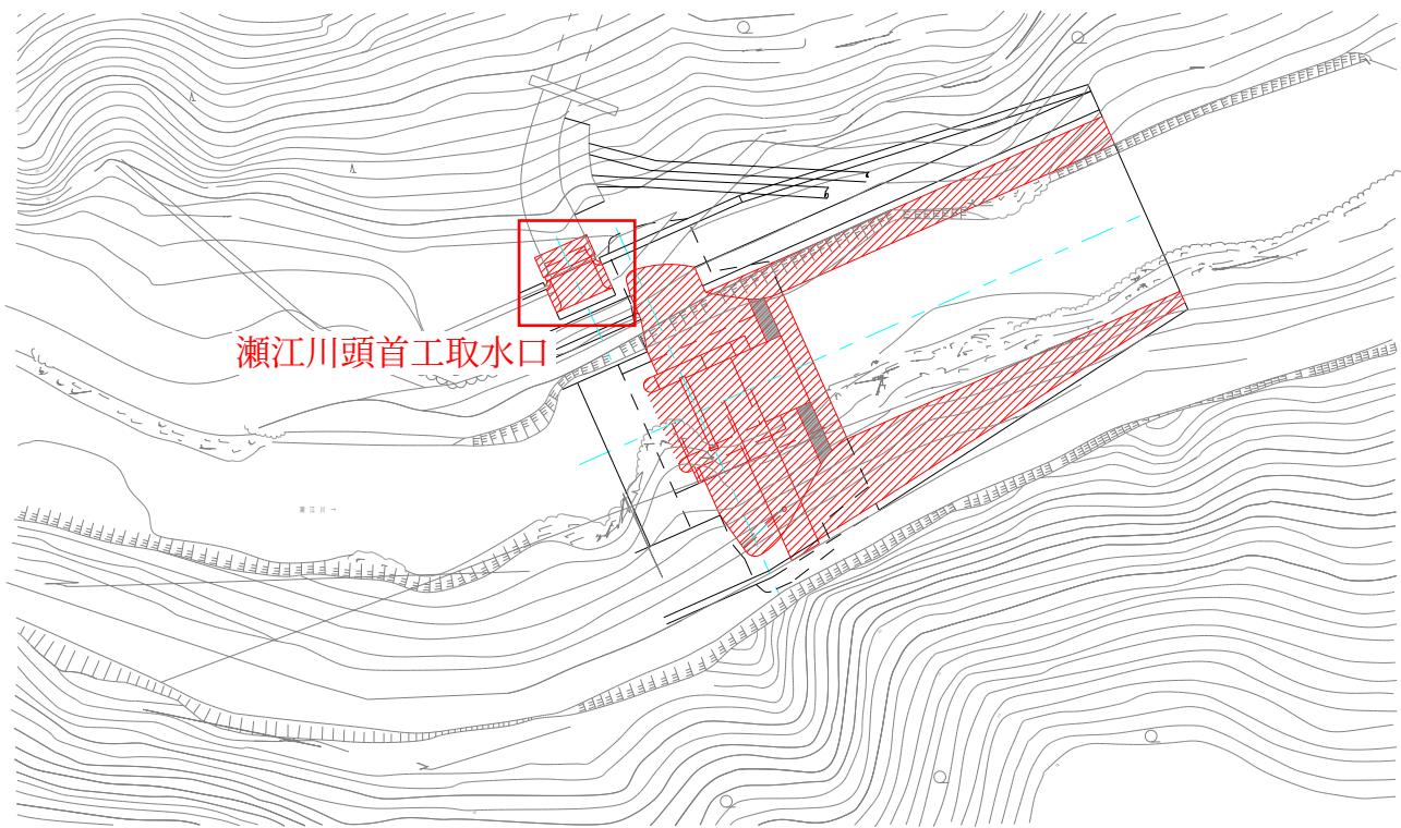
平面図 S=1:400
