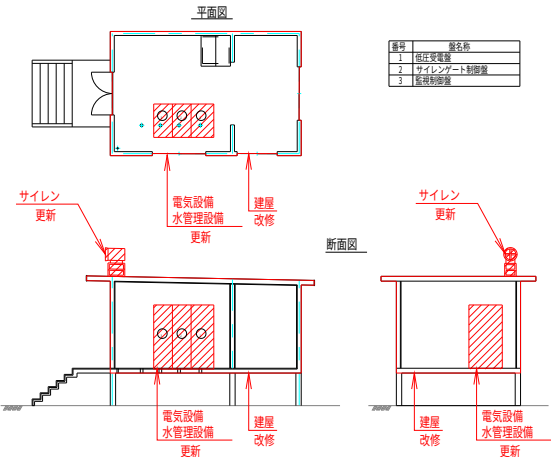
上屋内配線関係図 S=1:200
