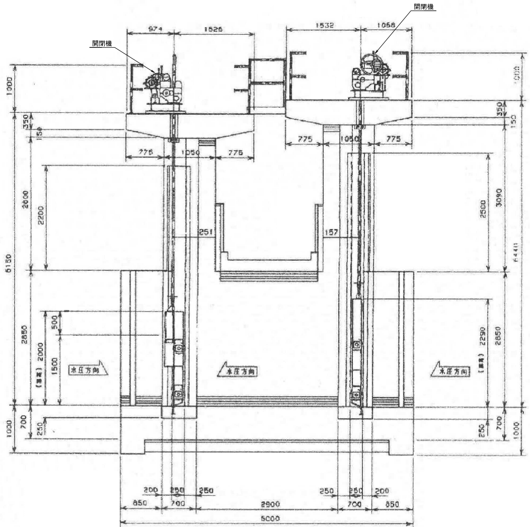
側面図
