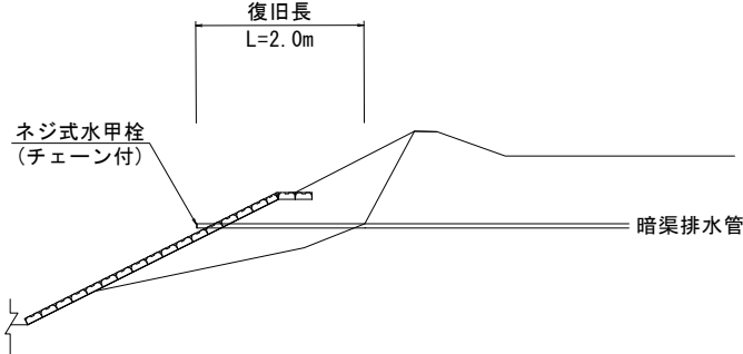
暗渠排水工復旧図
