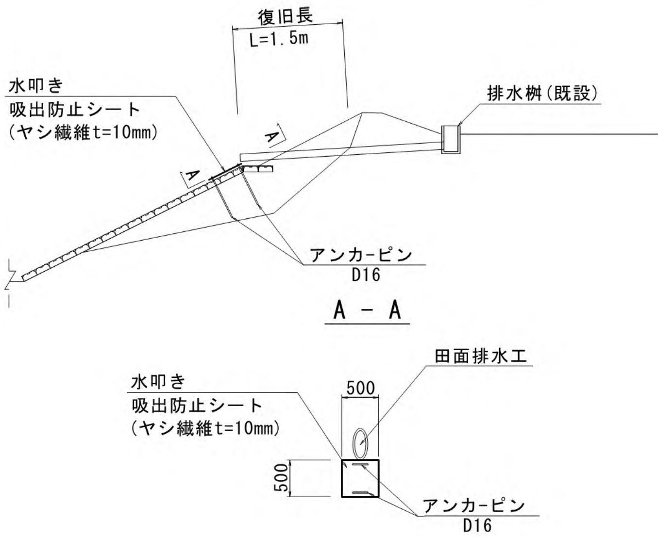
田面排水工復旧図
