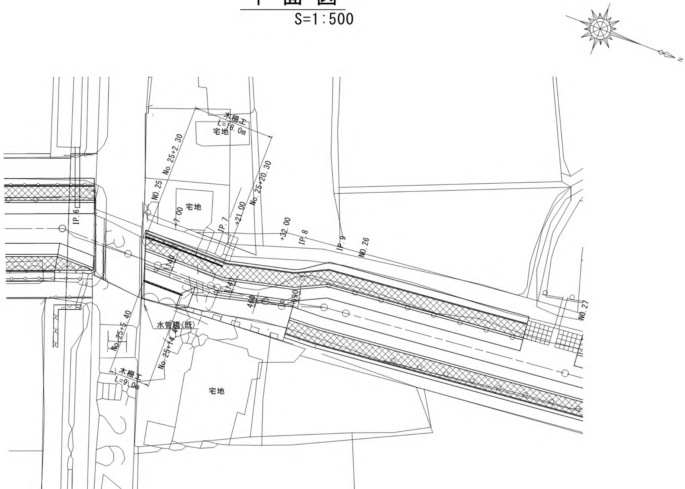
平 面 図
