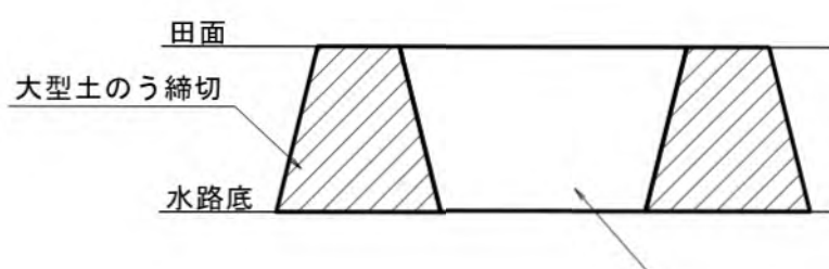
縦断面図
