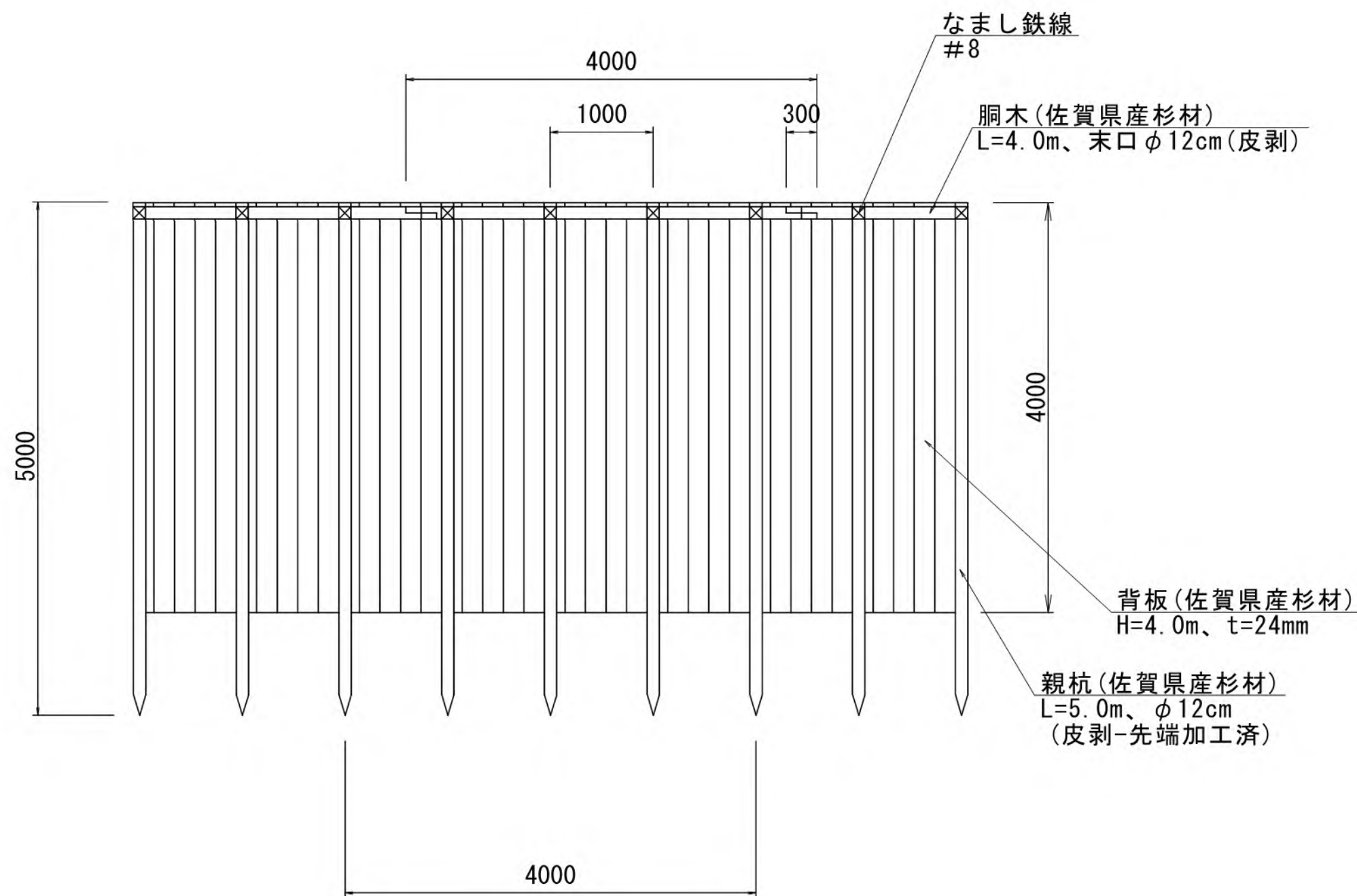
木柵工正面図
