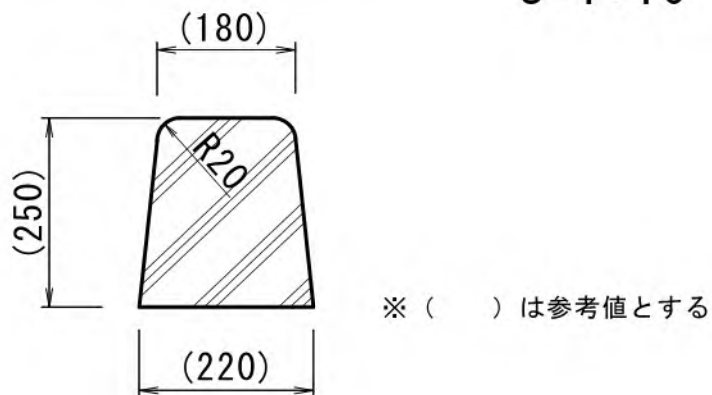
歩車道境界ブロック復旧図
