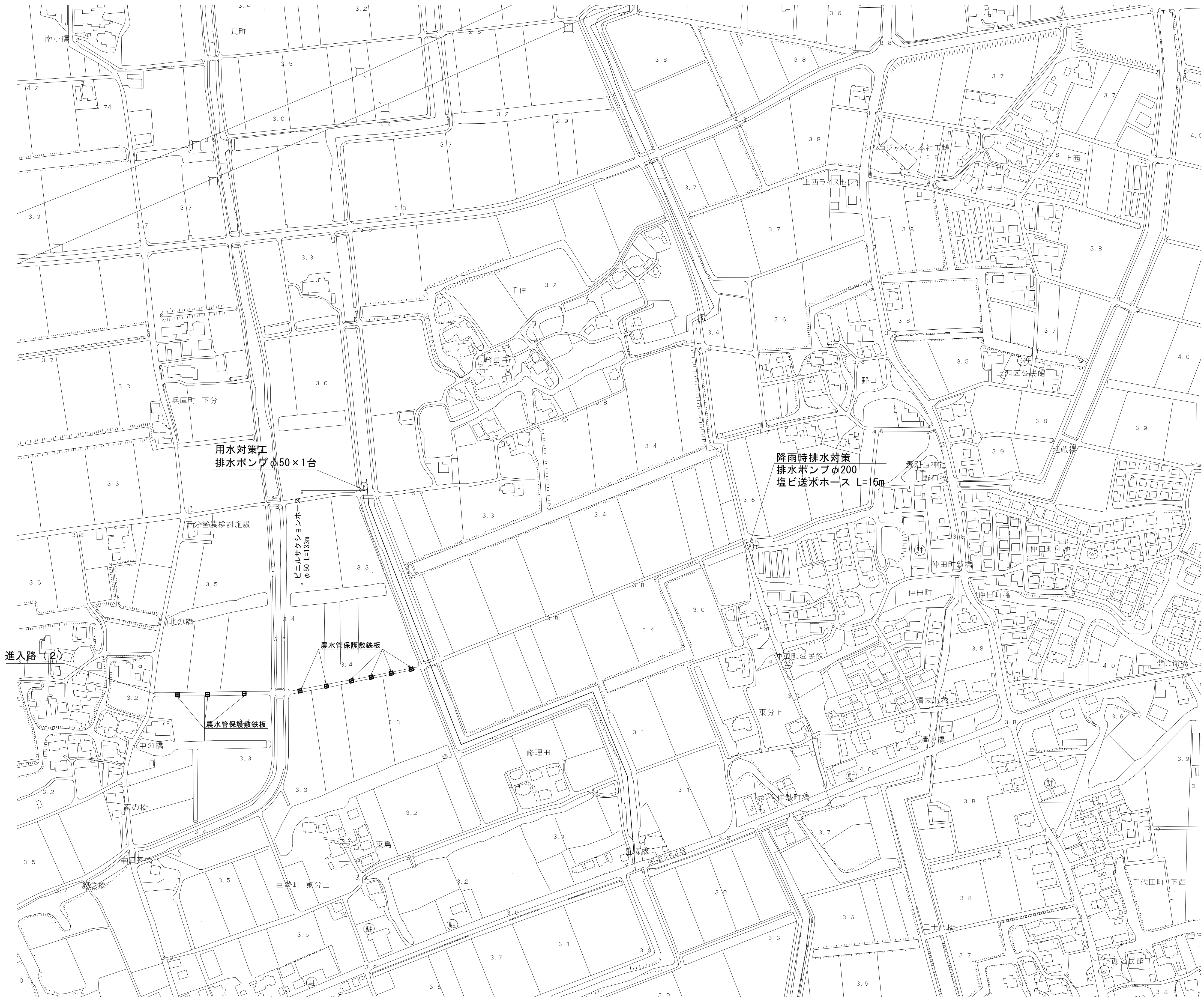
平面図 S=1:2500
