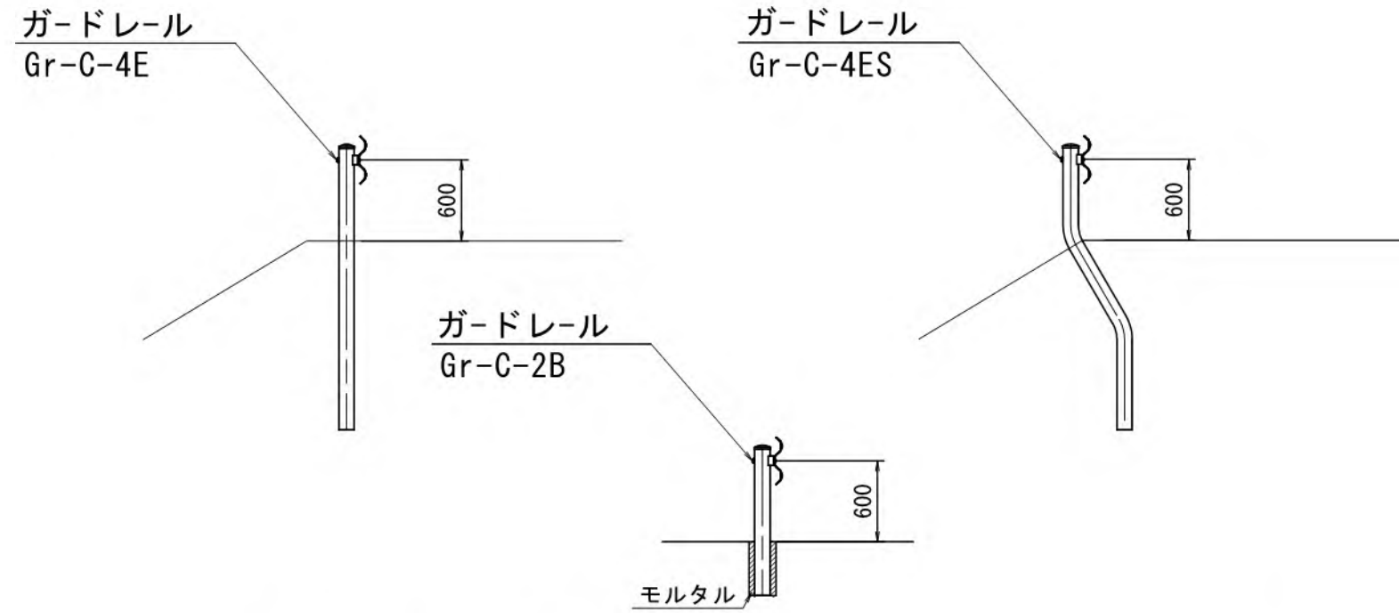
ガードレール復旧図
