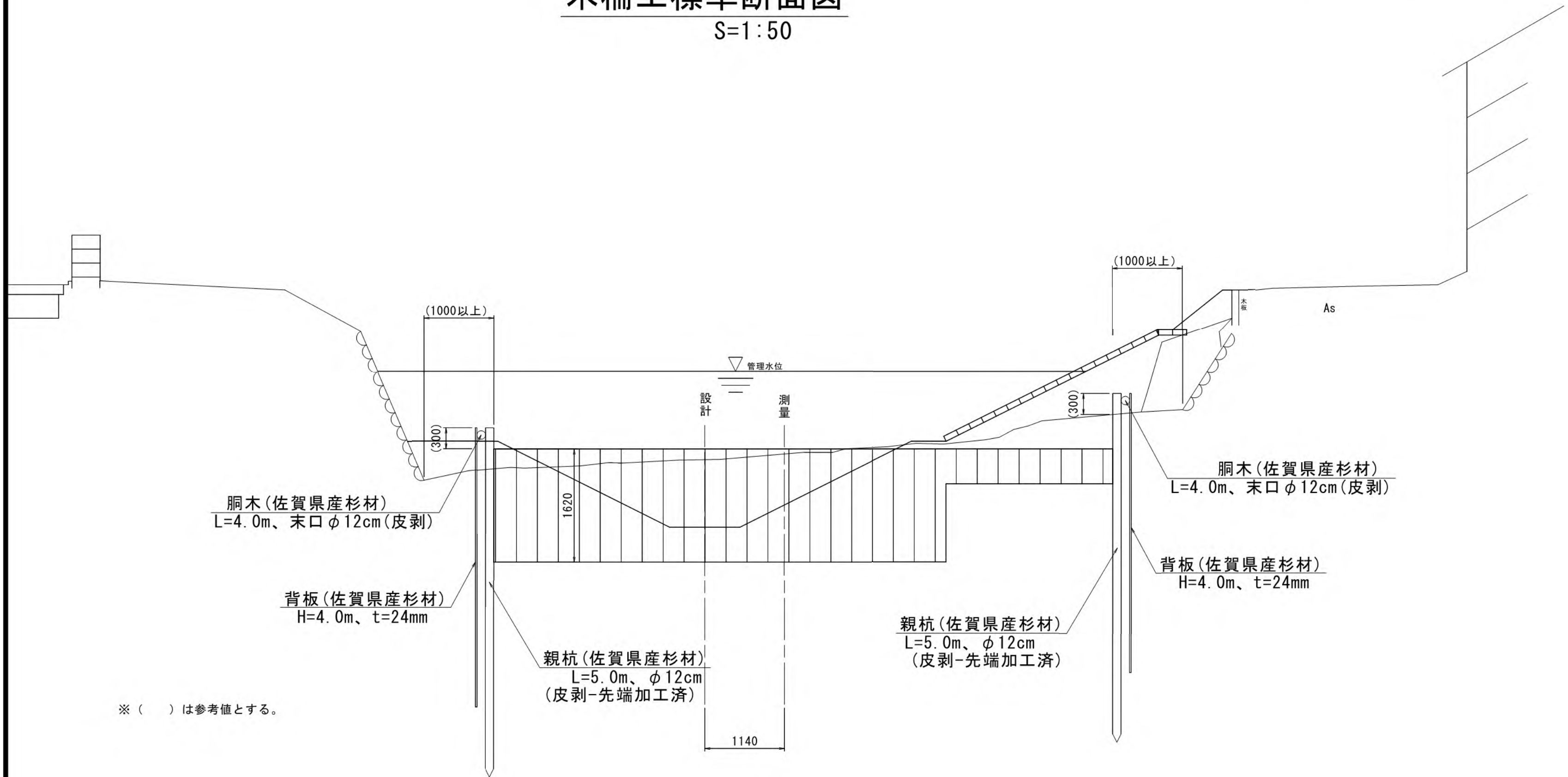
木柵工標準断面図
