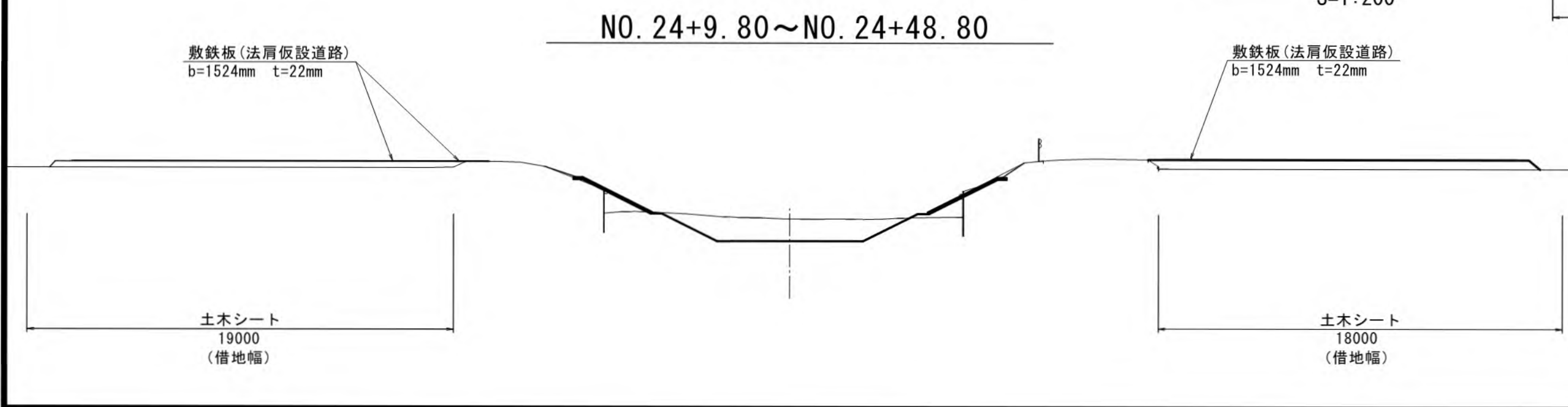
標準断面図 S=1:200
