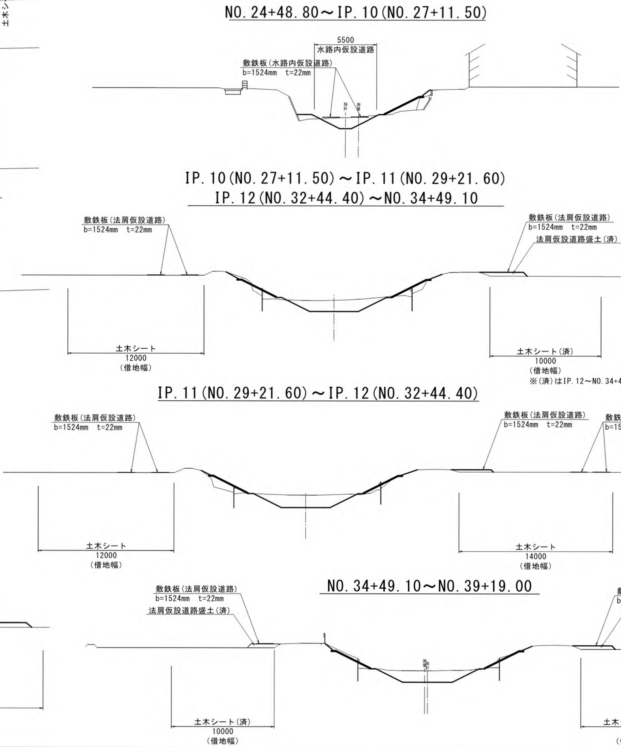
標準断面図 S=1:200
