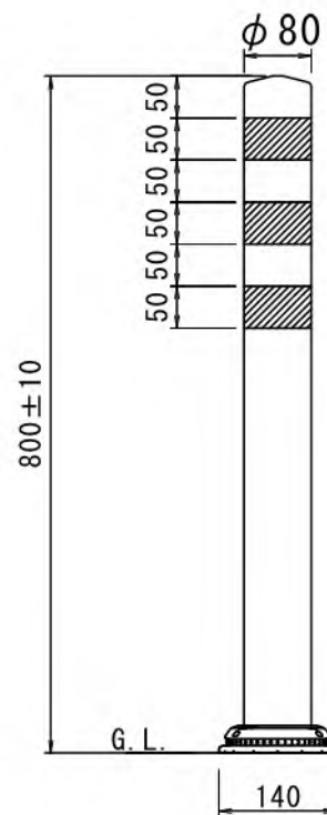
ラバーポール復旧図
