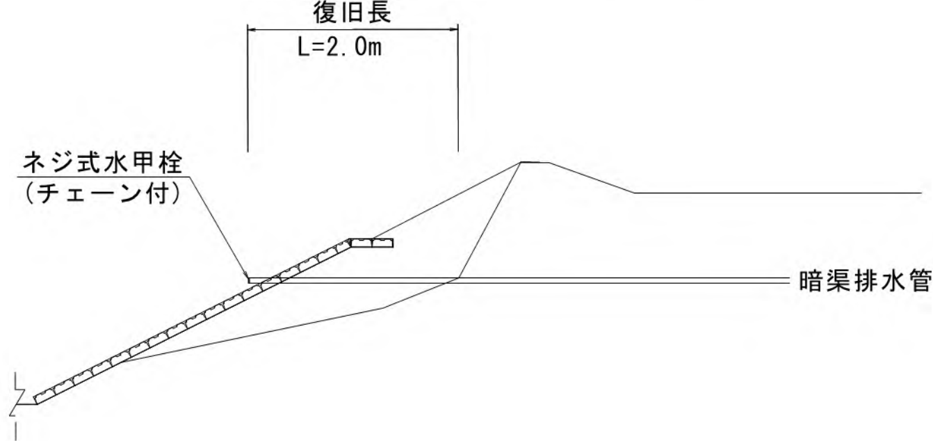
暗渠排水工復旧図
