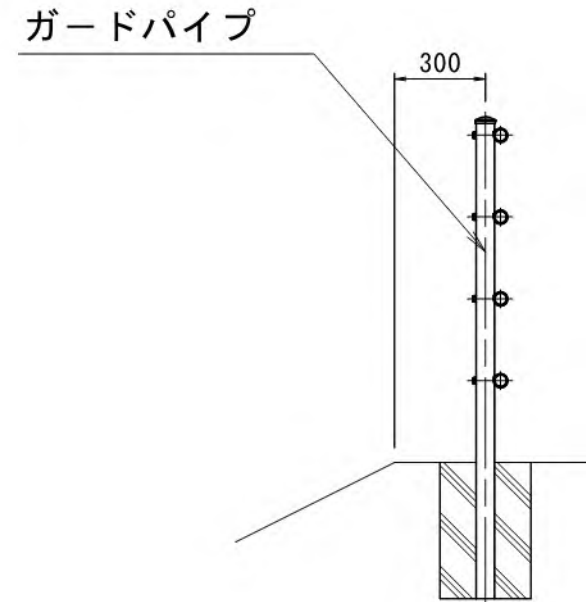
ガードパイプ復旧図
