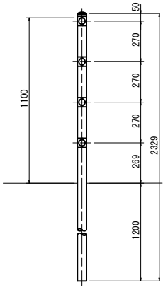
転落防止柵復旧図
