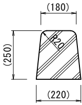
歩車道境界ブロック復旧図
