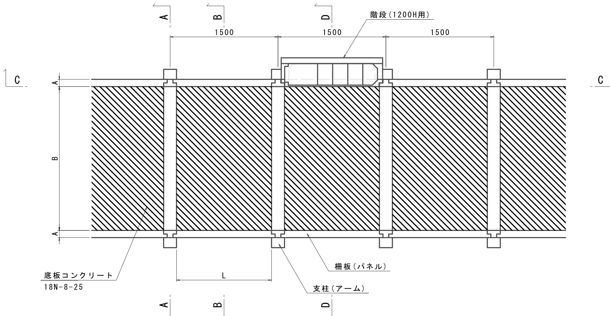
C-C 断面
