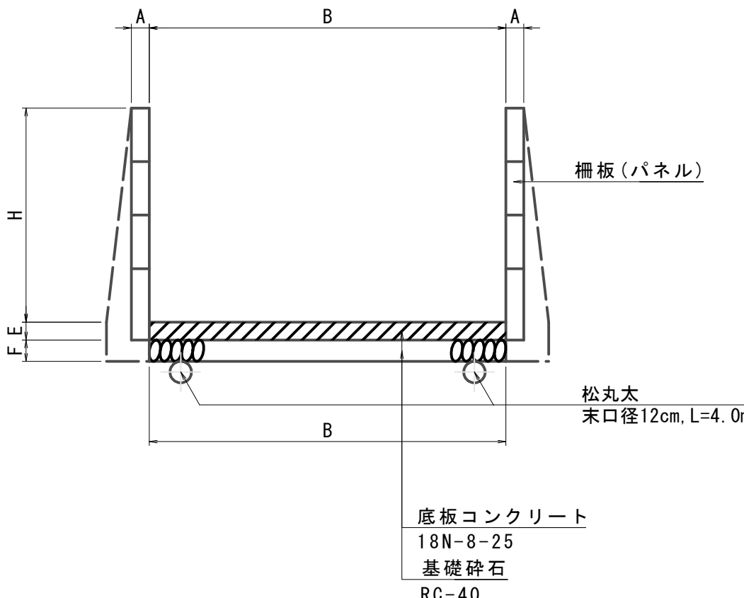
B-B 断面
