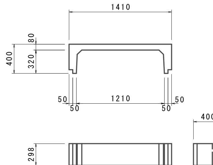
階段下板詳細図
