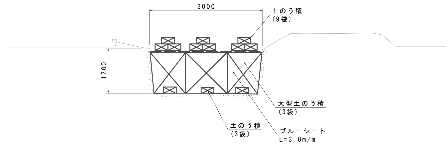
土のう締切標準図(5)
