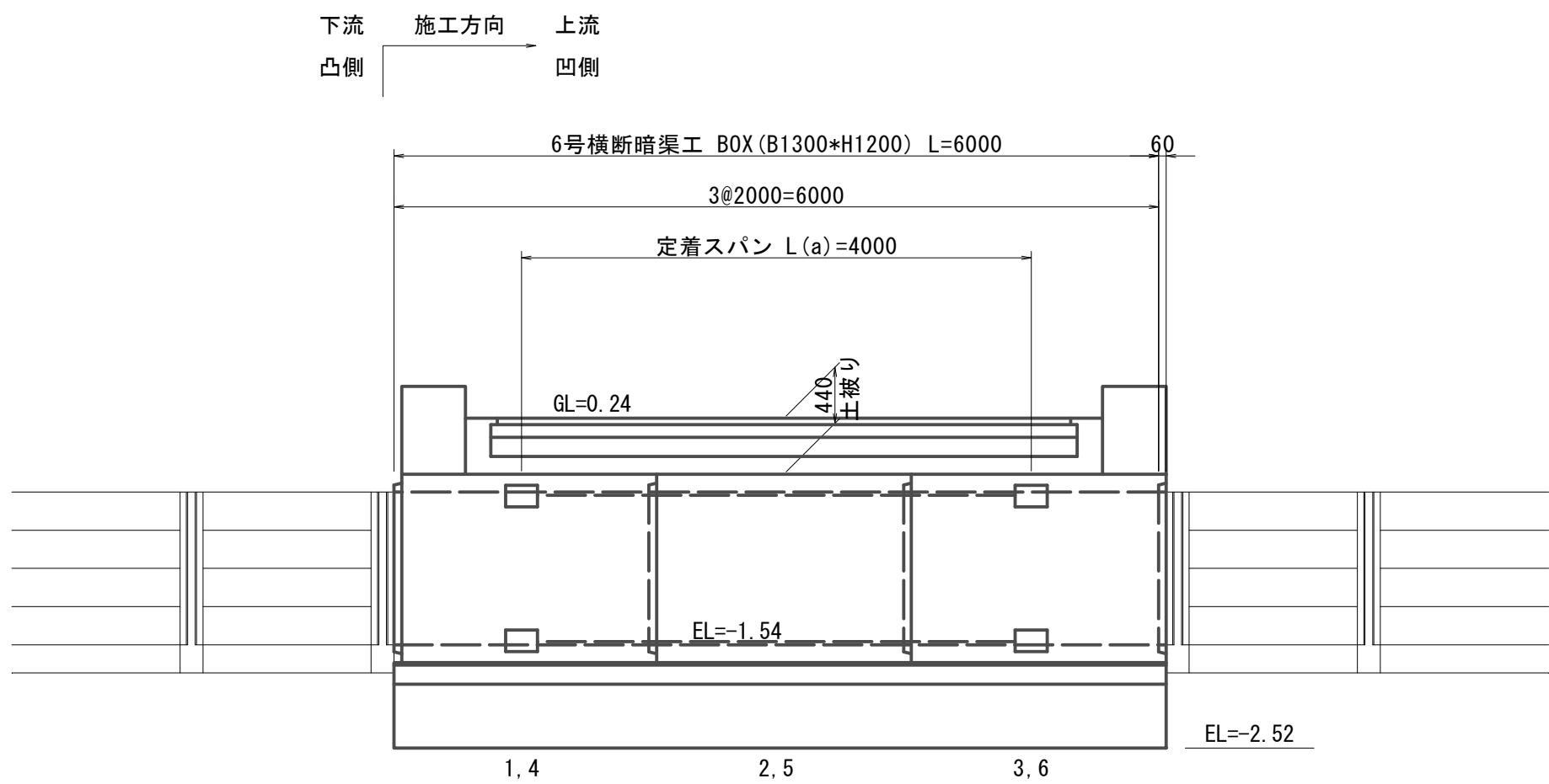
側面図 S=1:50
