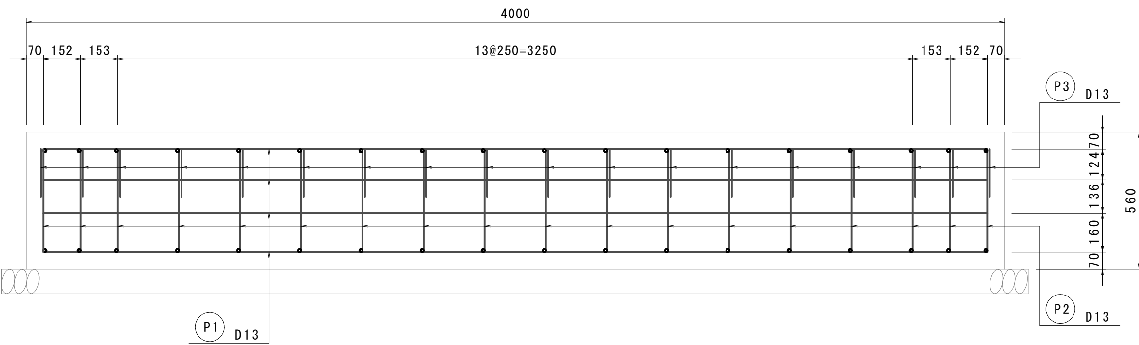
C-C断面図
