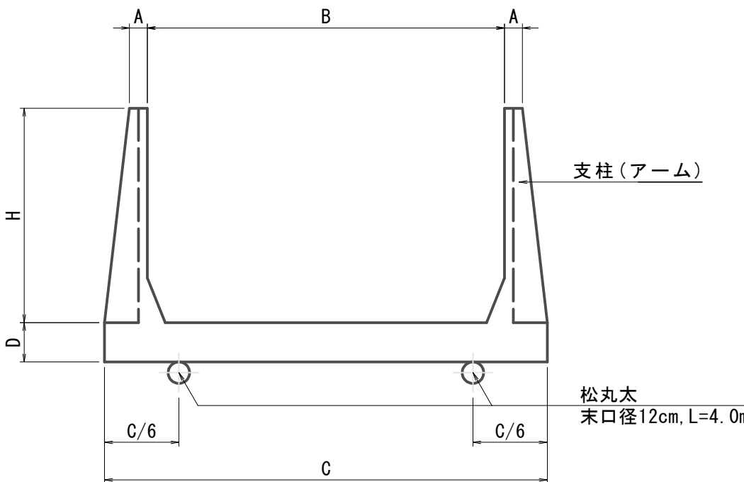
A-A 断面
