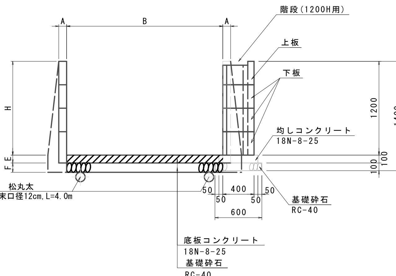
D-D 断面
