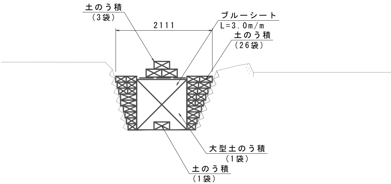
土のう締切標準図(7)
