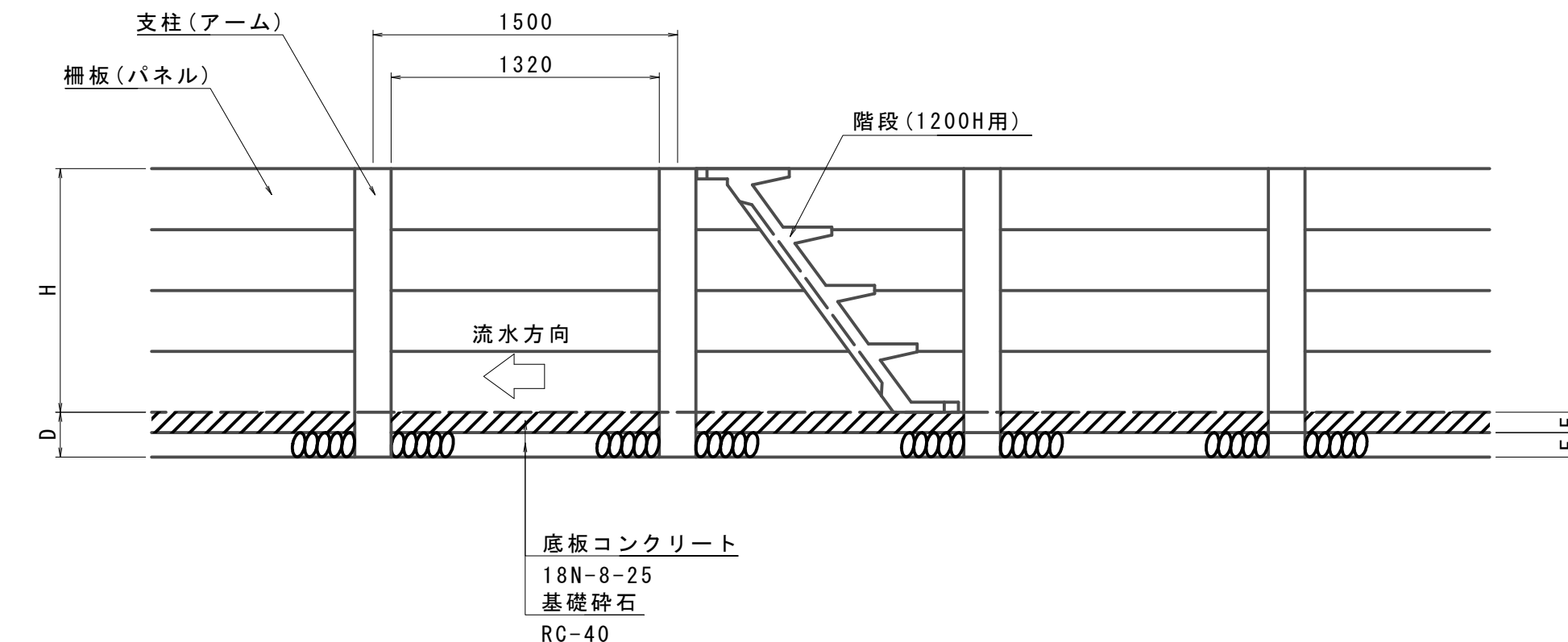
A-A 断面
