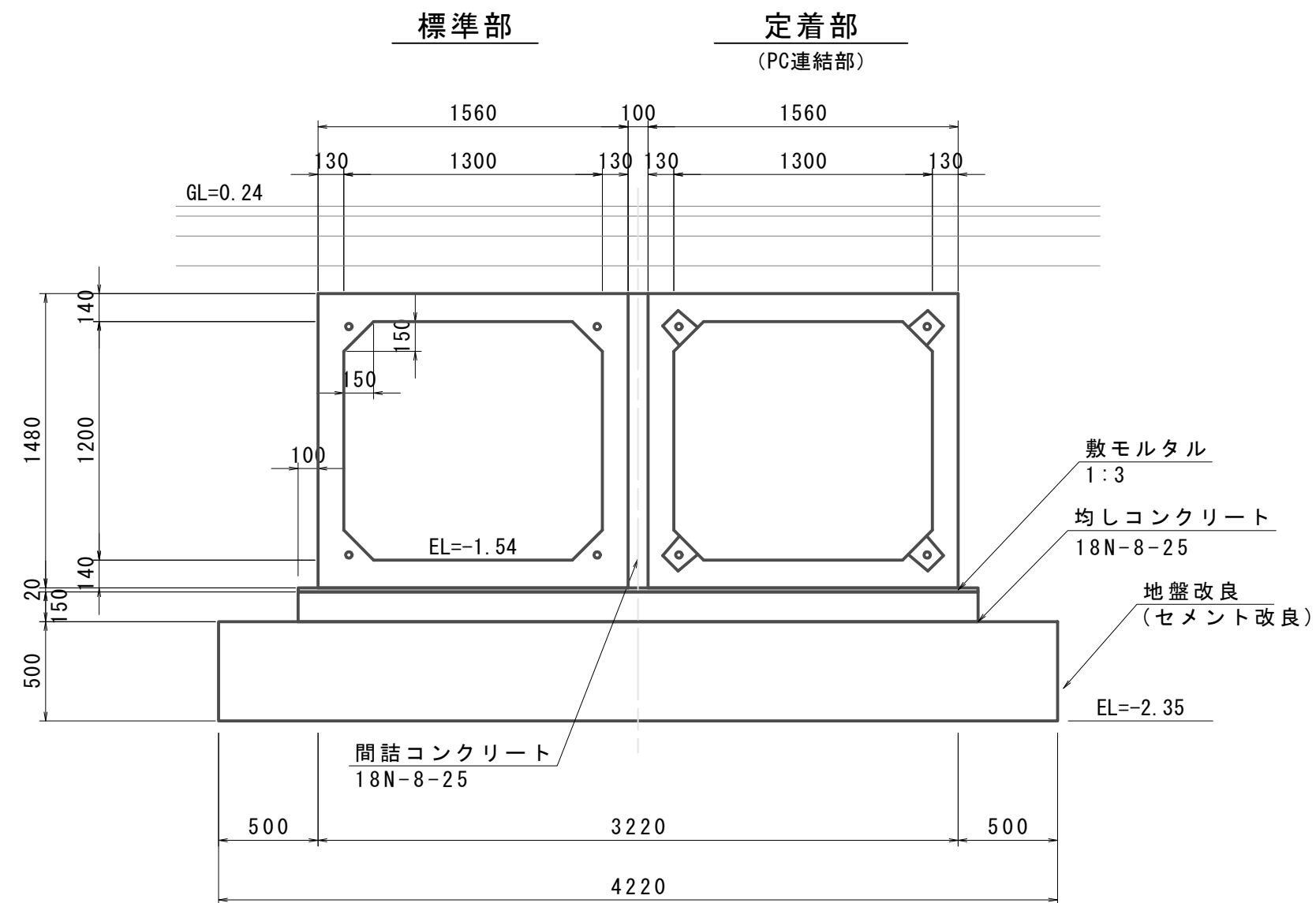
断面図 S=1:30
