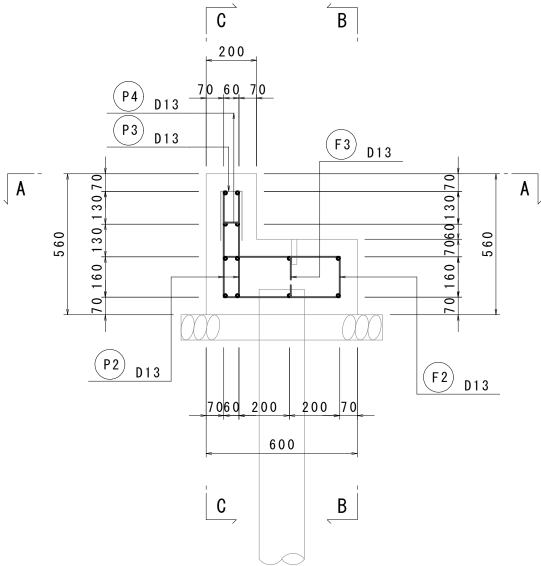
断面図
