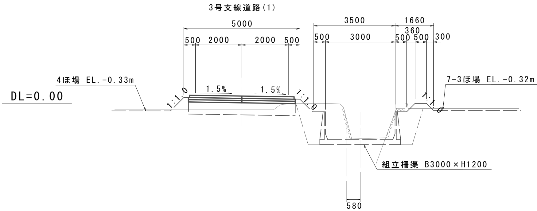
標準断面図 S=1:100
