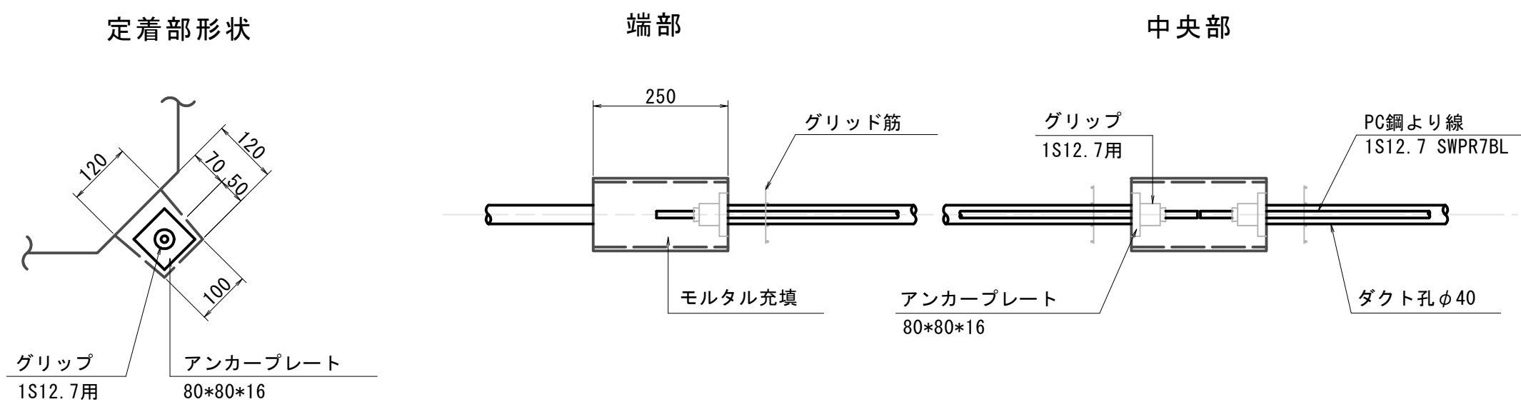
PC縦連結詳細図 S=1:10
