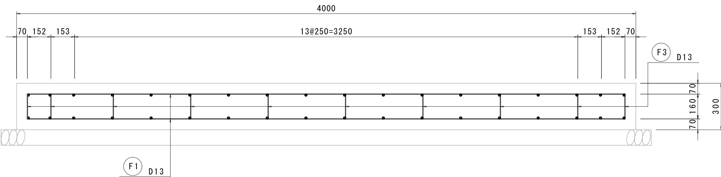
B-B断面図
