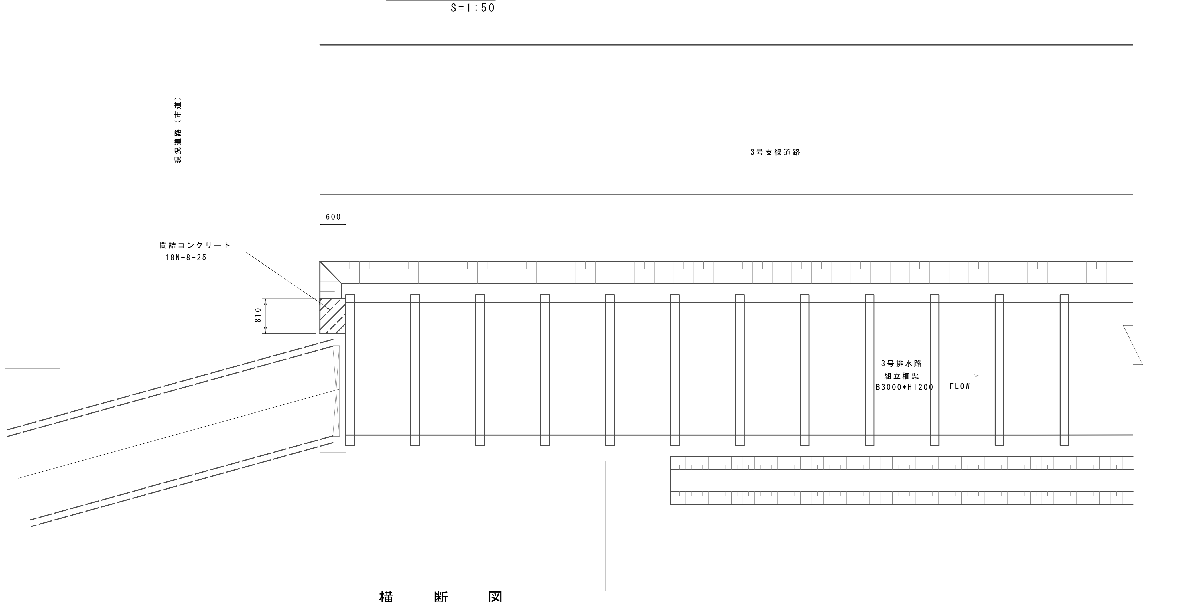
横 断 図 S=1:50
