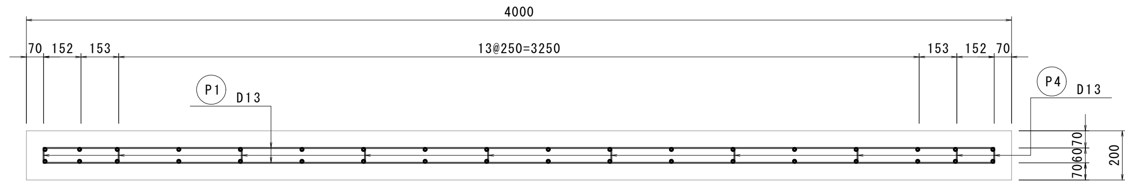
A-A断面図
