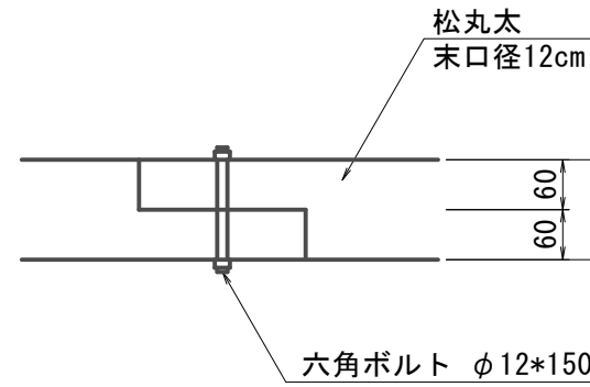
洞木継手詳細図
