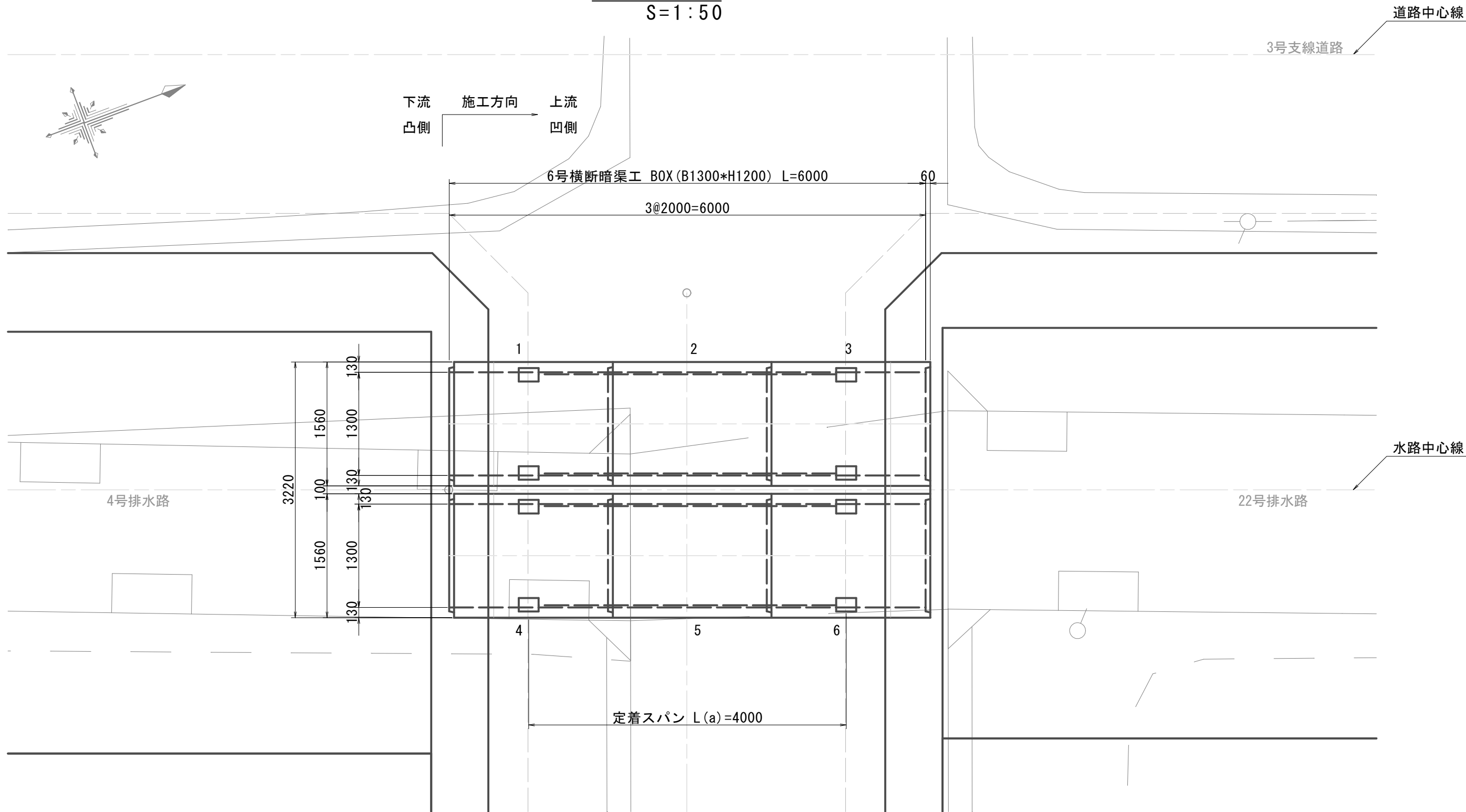
平面図 S=1:50
