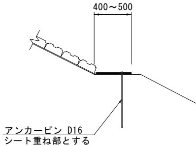
小段詳細図 S=1:20 (C)
