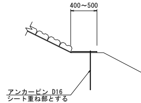
小段詳細図 S=1:20 (B)
