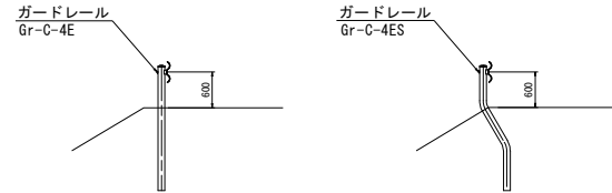
ガードレール復旧図
