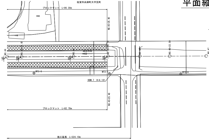
平面図 S=1:500
