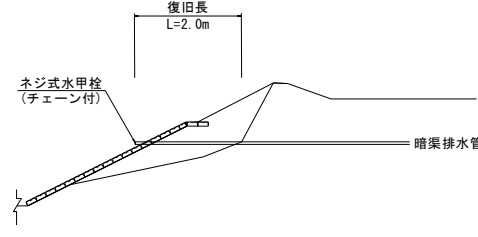
暗渠排水工復旧図
