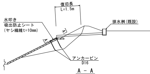
田面排水工復旧図
