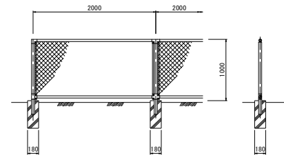
ネットフェンス復旧図
