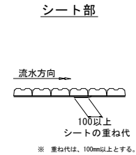
接続部詳細図 S=1:20
