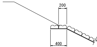
法肩詳細図 S=1:20 (A)
