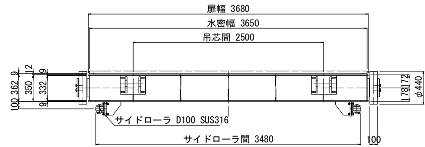
平面図
