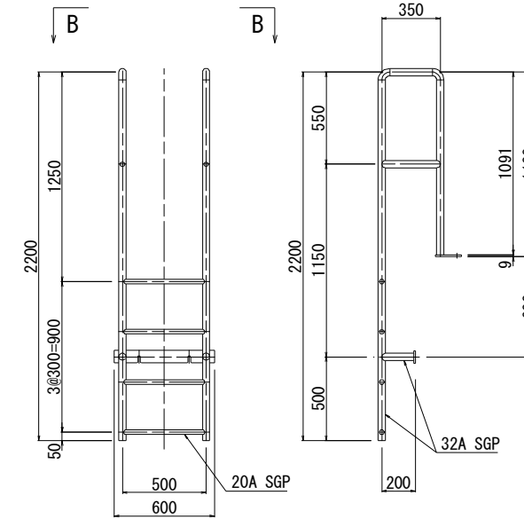
タラップ組立図 S=1:20
