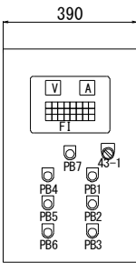
ゲート盤
