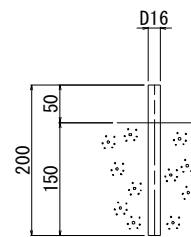
差筋施工図 S=1:5
