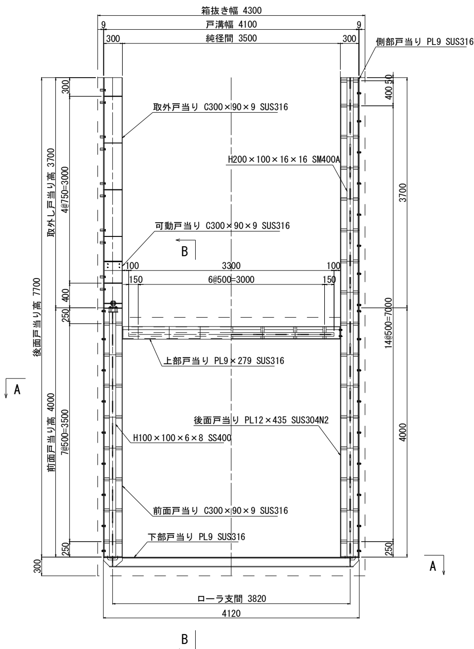
正面図
