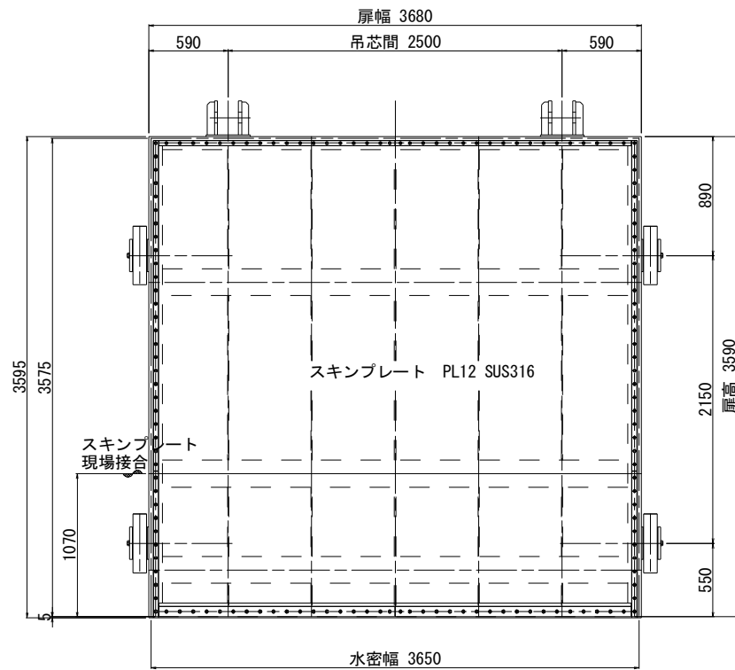
背面図
