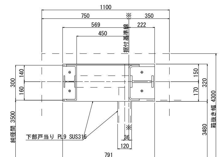
E - E_{\Sigma} \approx 1 \cdot 10^4
