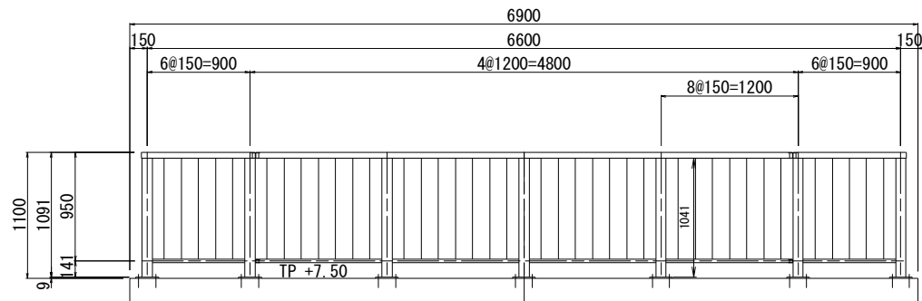
正面図 S=1:30
