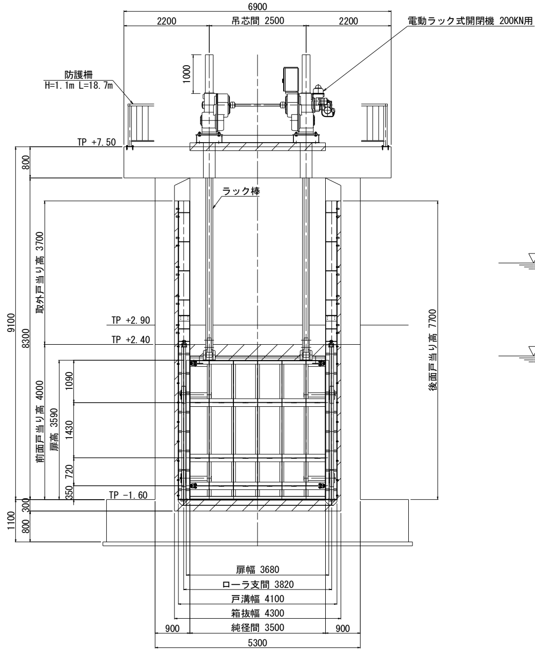
正面図
