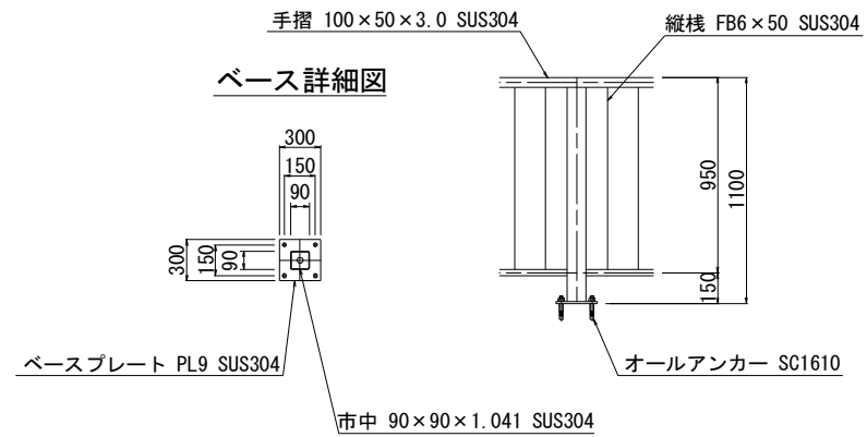
防護柵標準図 S=1:20
