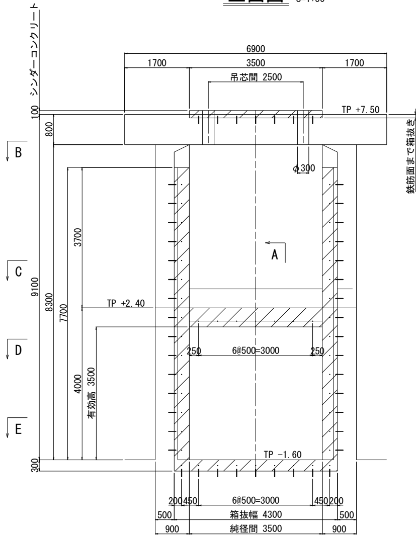
正面図 S=1:50
