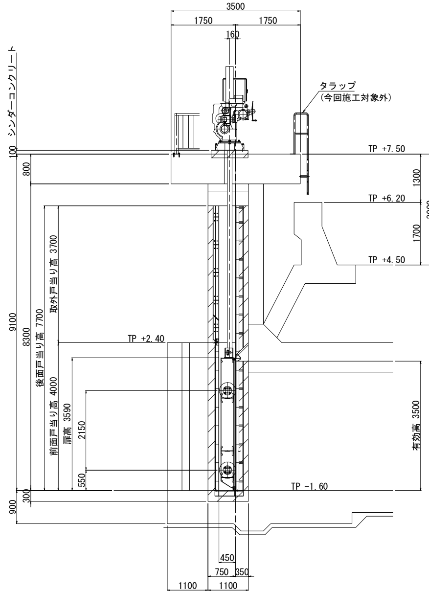
側面図
