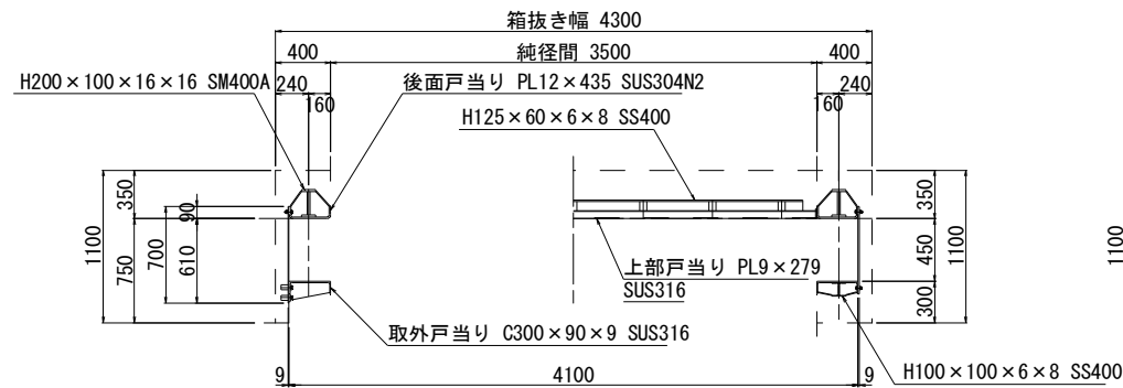
平面図 S=1:30
