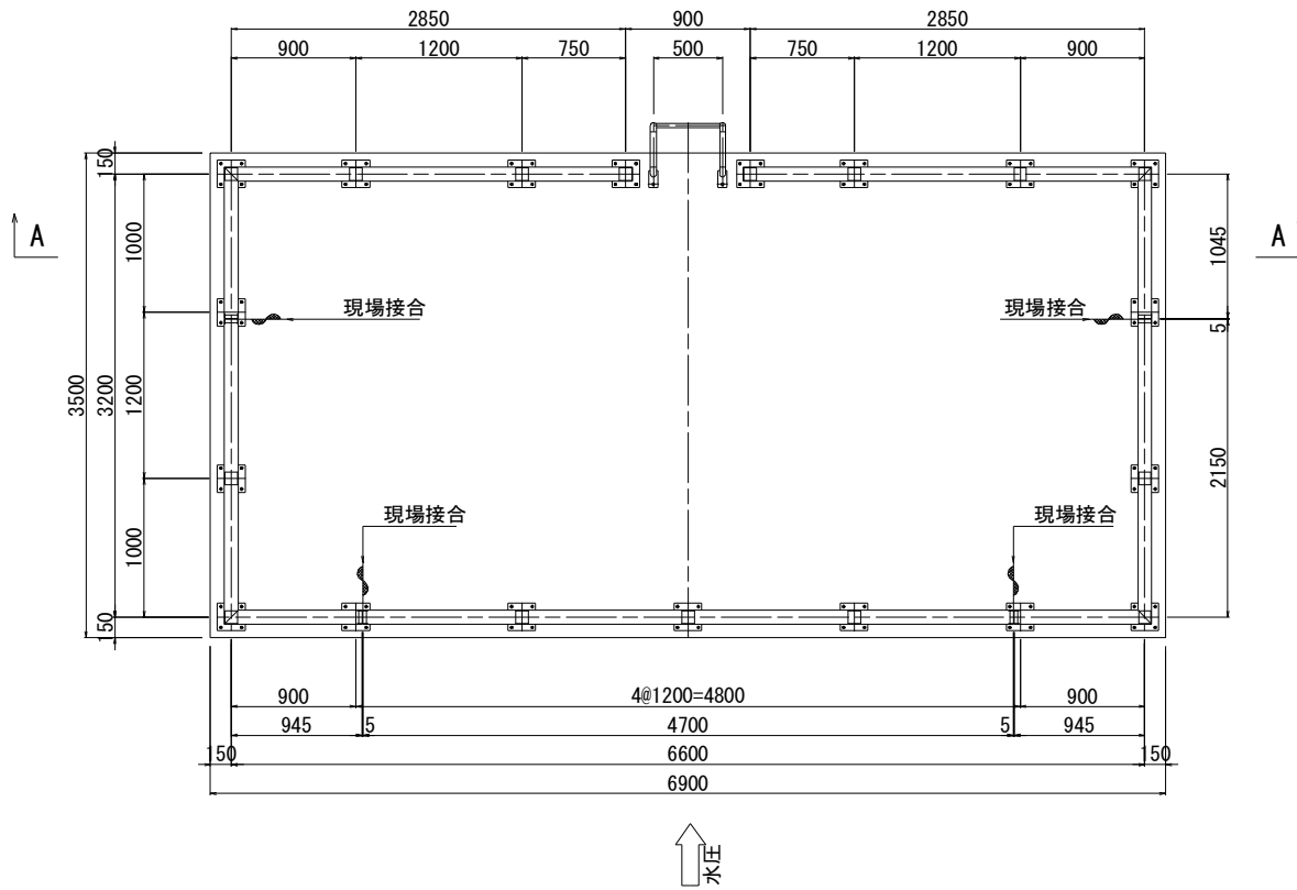
平面图 S=1:30
