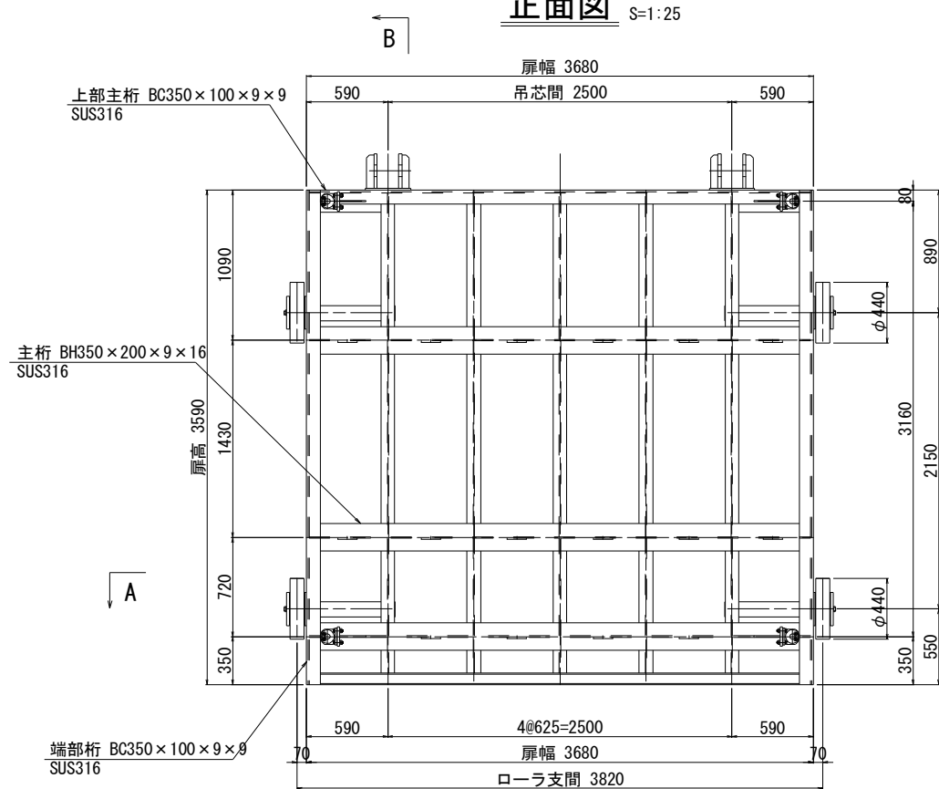
正面図
