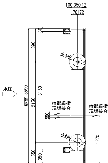
側面図
