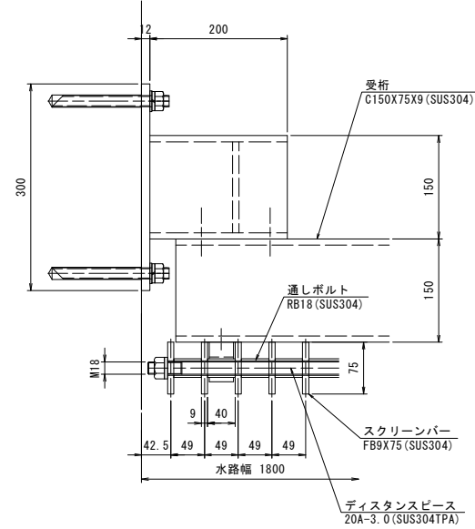
端部詳細図 S=1:5
