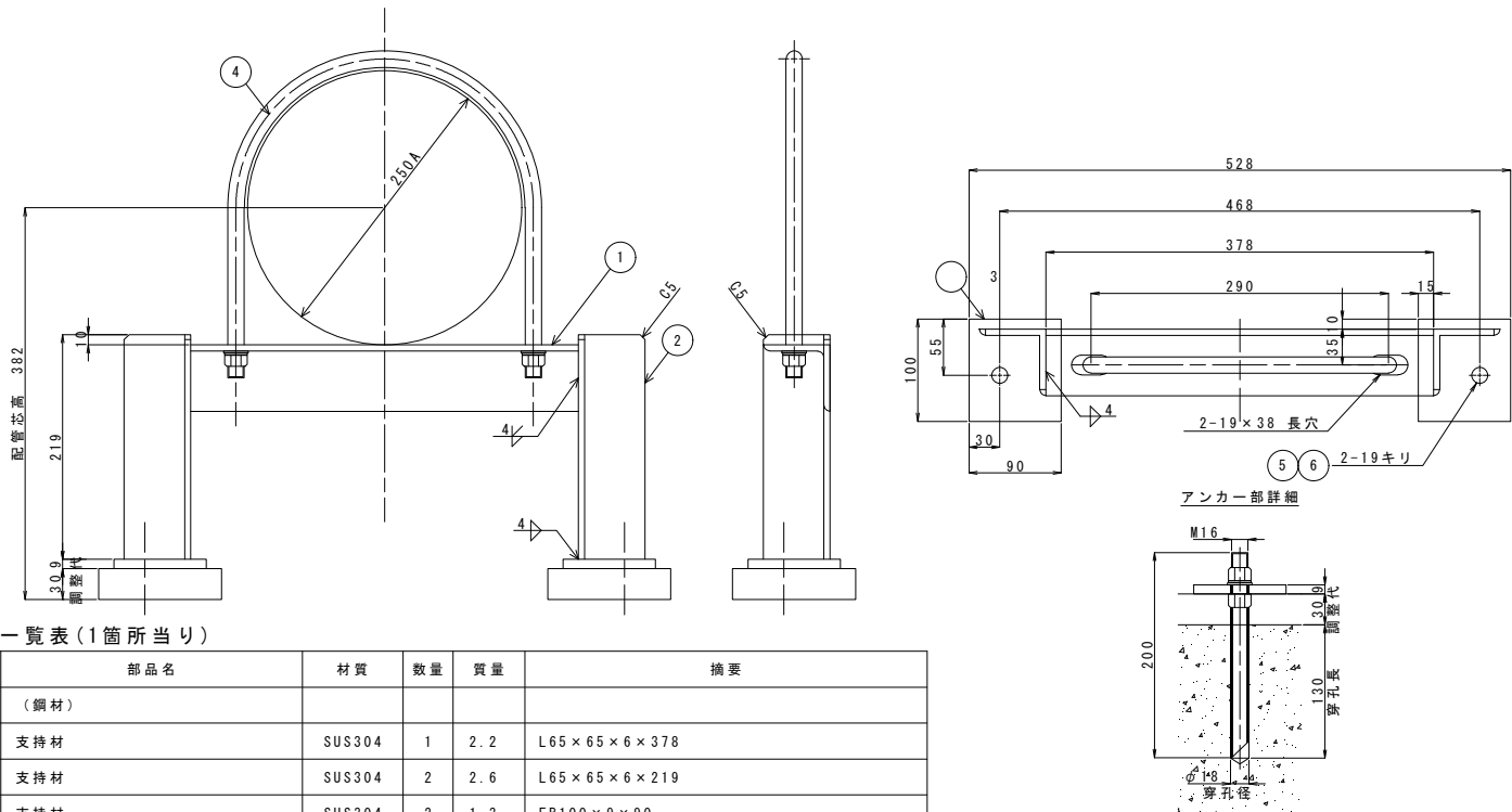
配管サポート③詳細図
