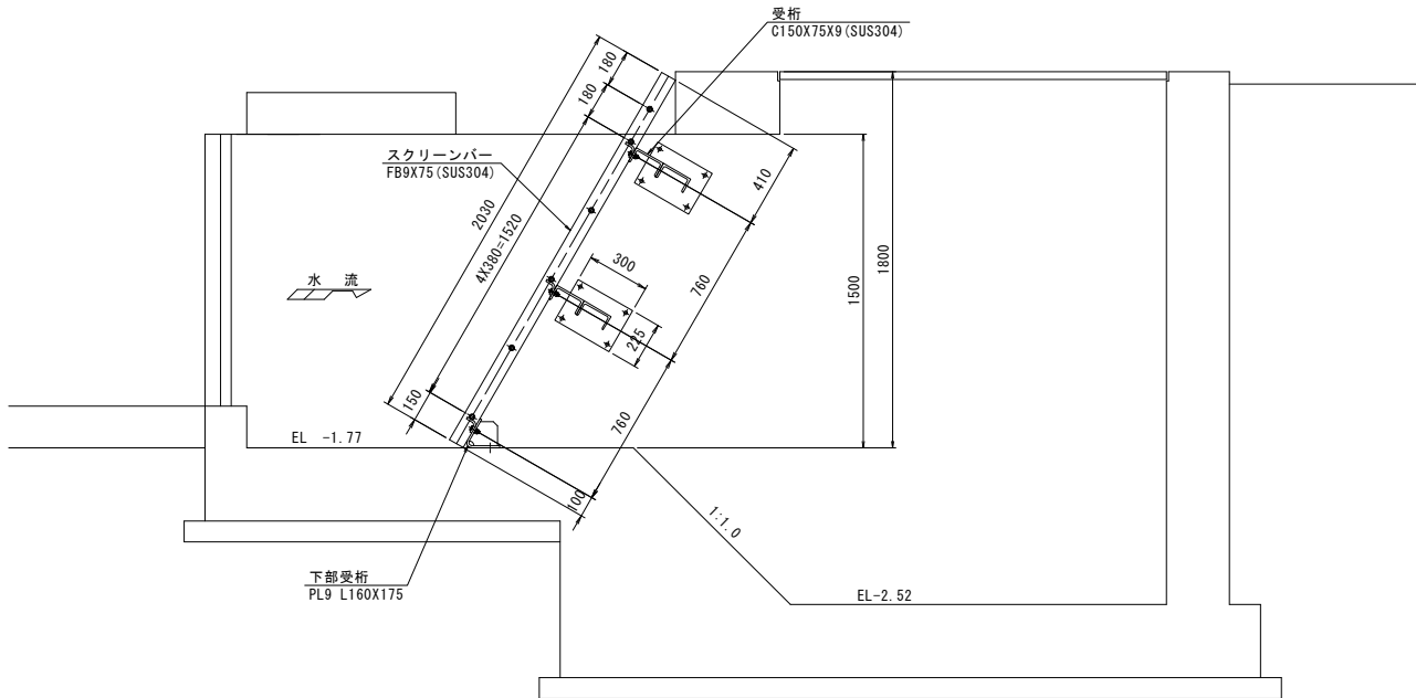
断面図 S=1:20
