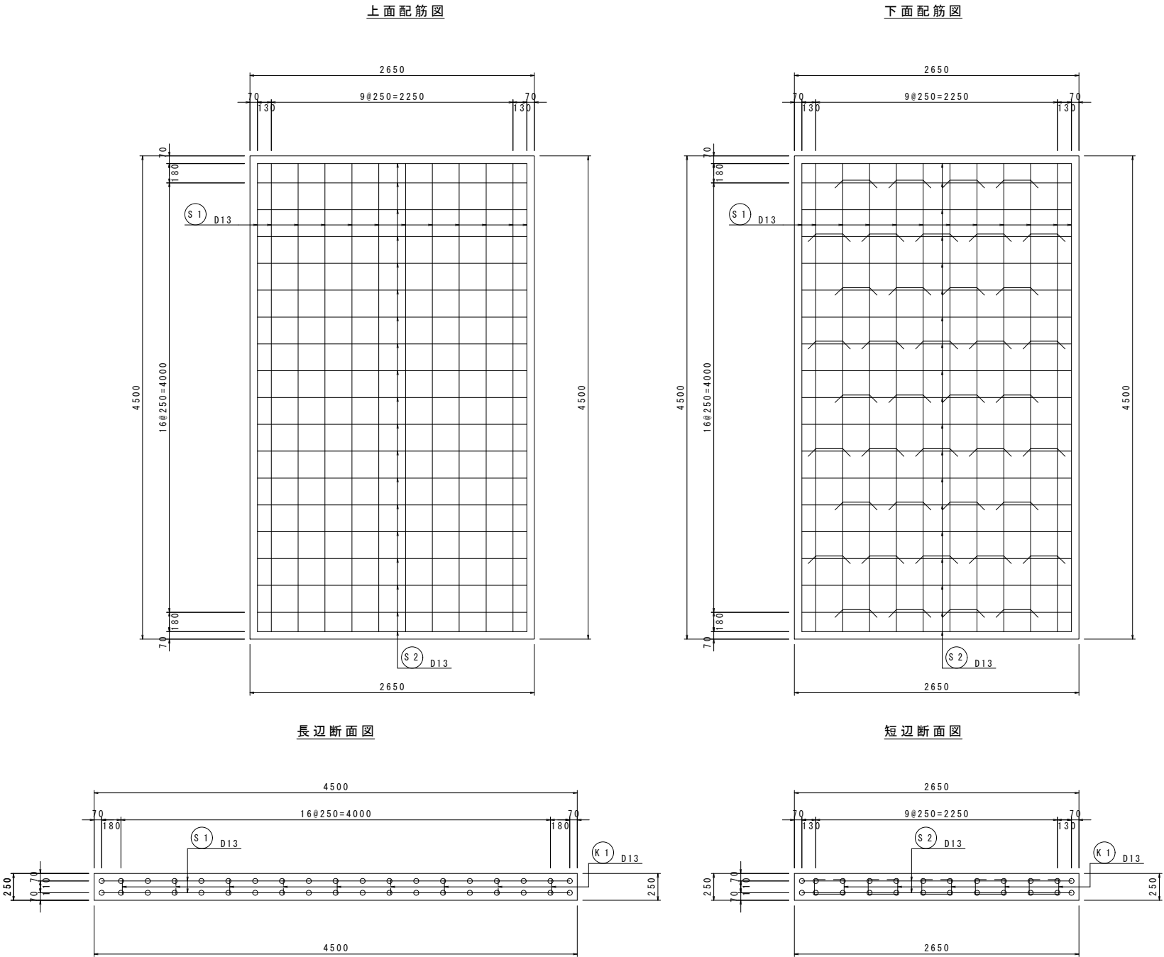
配管基礎部 加工図
