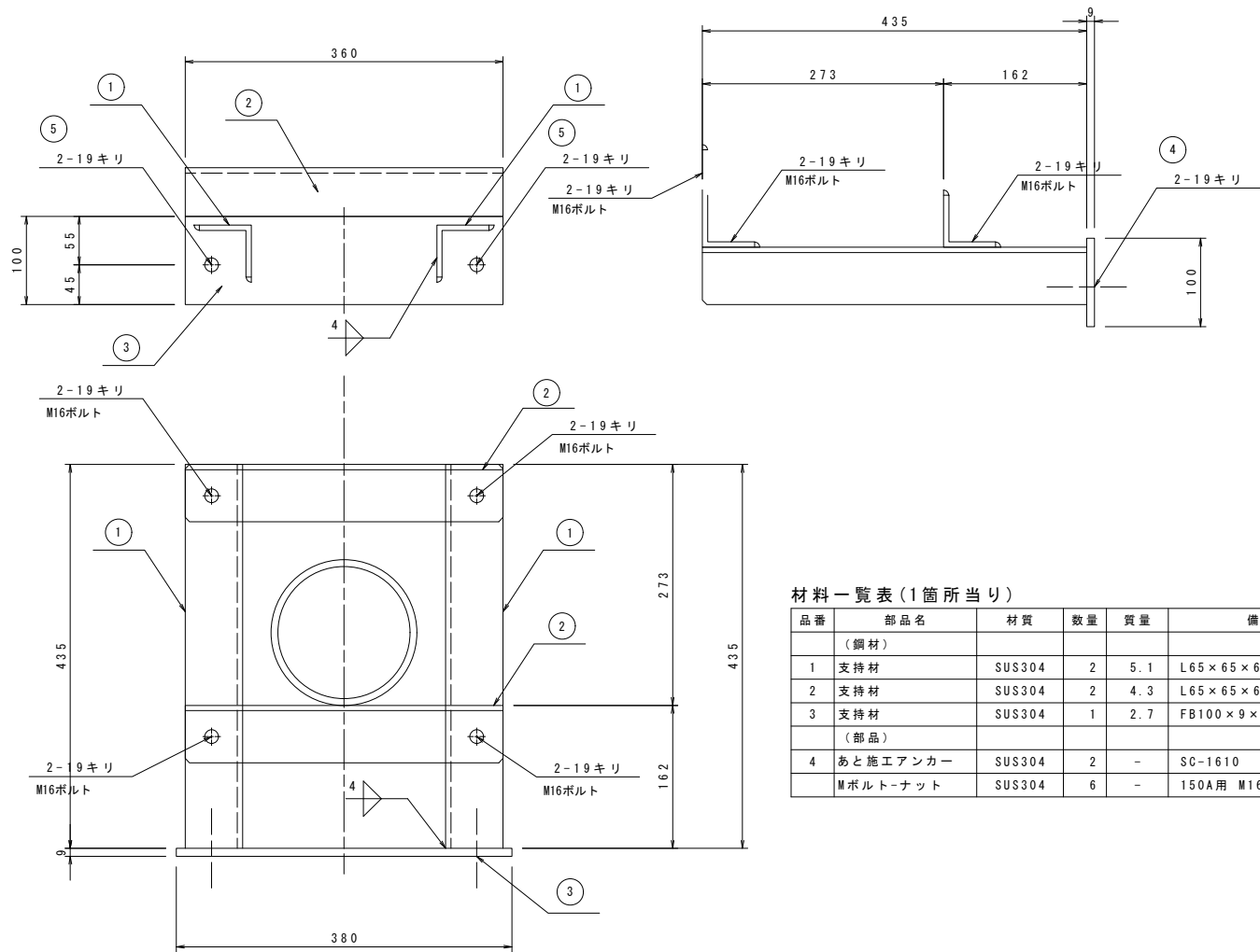
配管サポート②詳細図
