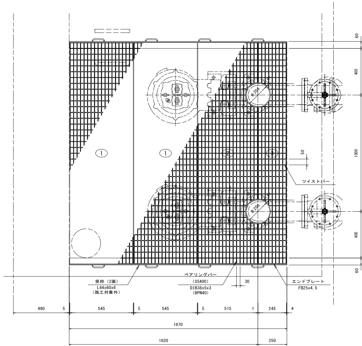
平面図
