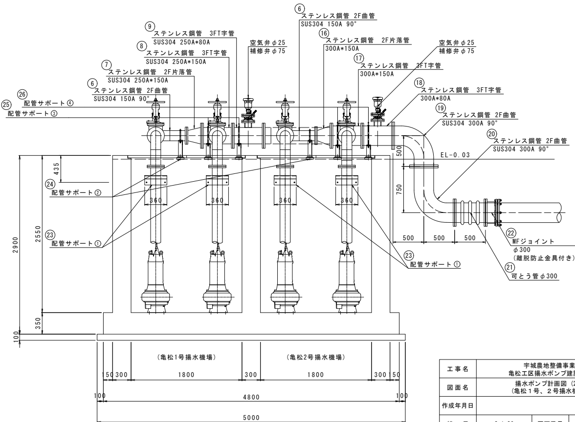
B-B断面図
