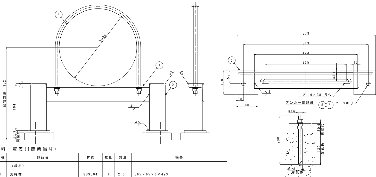
配管サポート④詳細図
