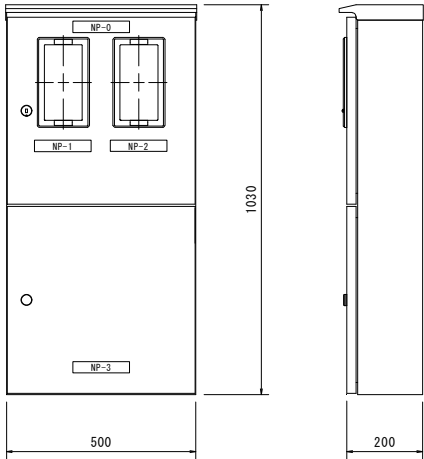
正面図
