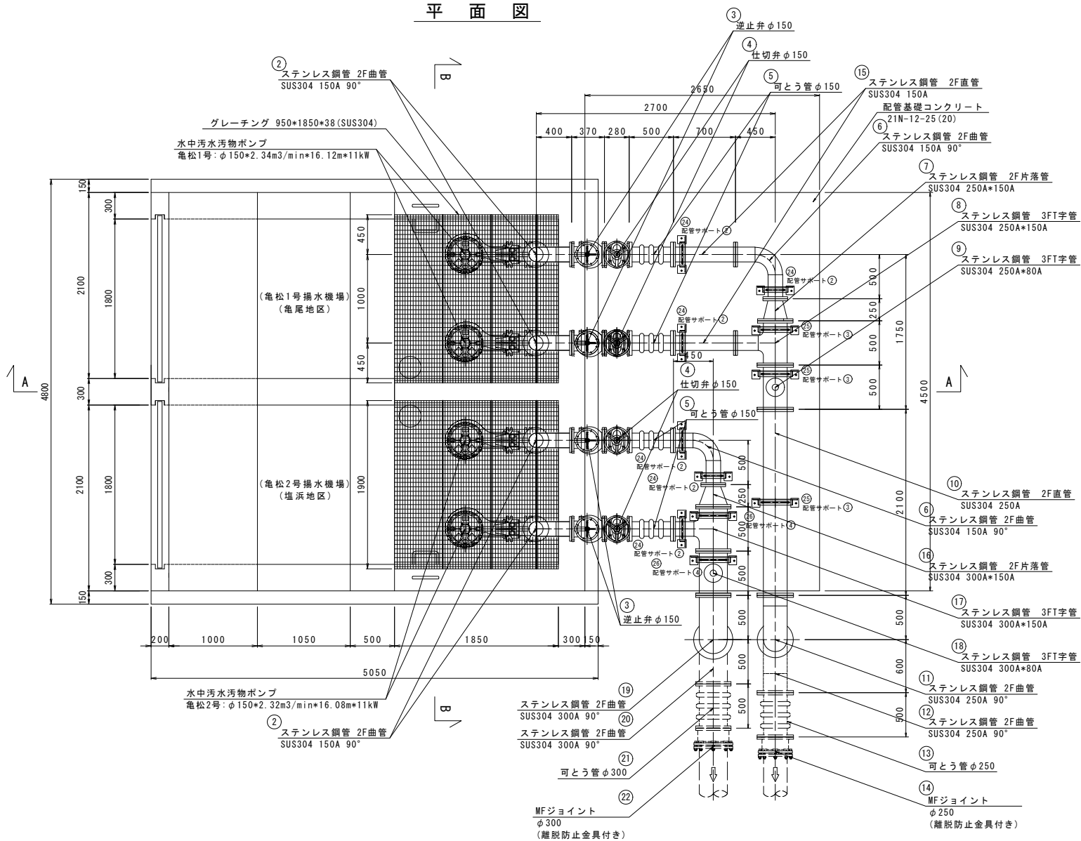
平面図
