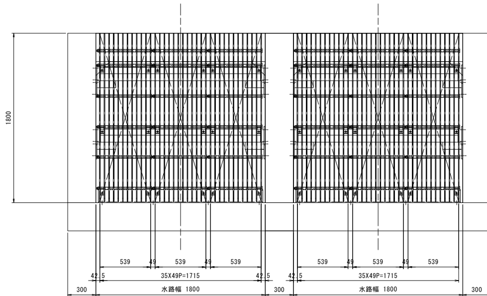
正面図 S=1:20
