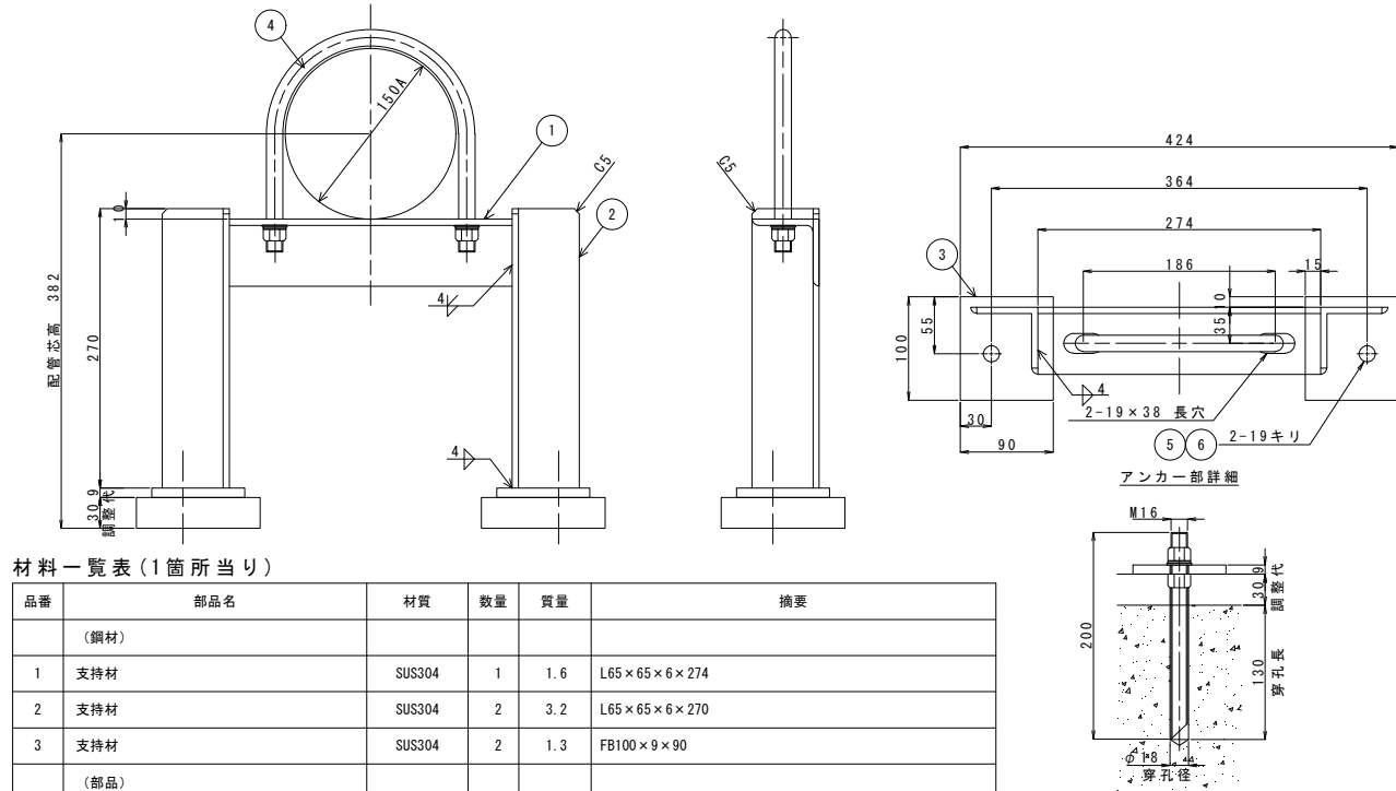
配管サポート②詳細図
