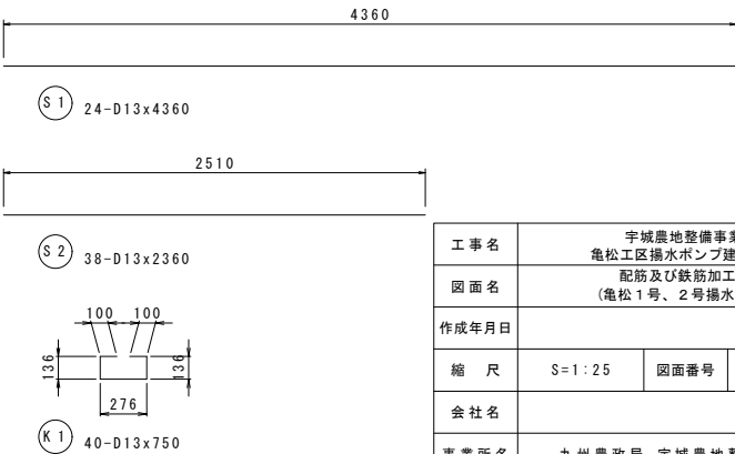
配管基礎部 加工図
