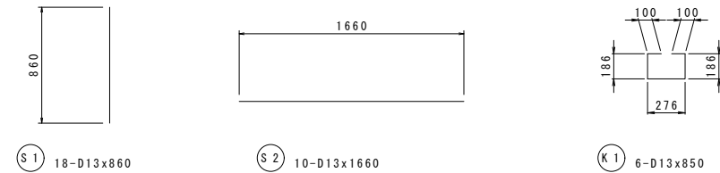
制御盤基礎部 加工図
