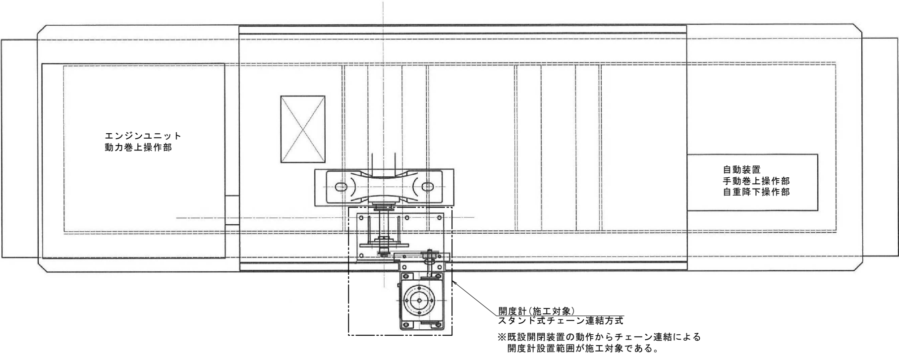
側面図
