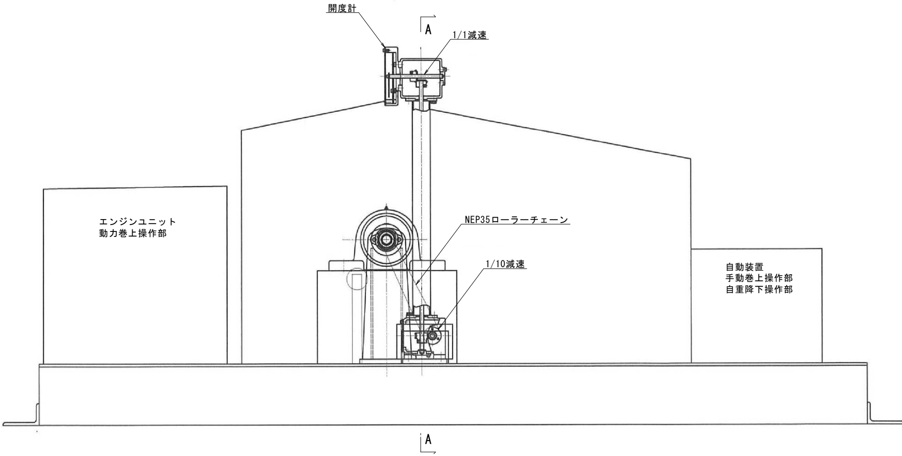
側面図
