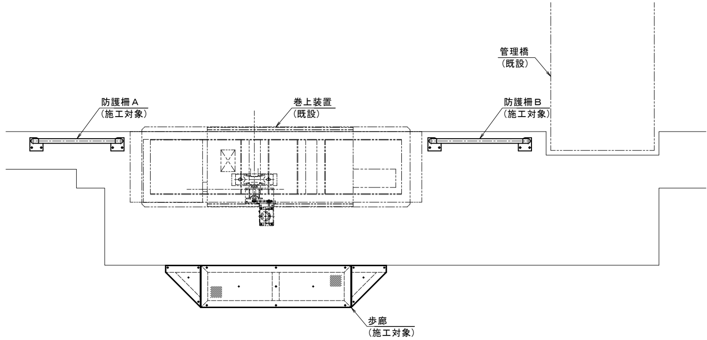
平面図
