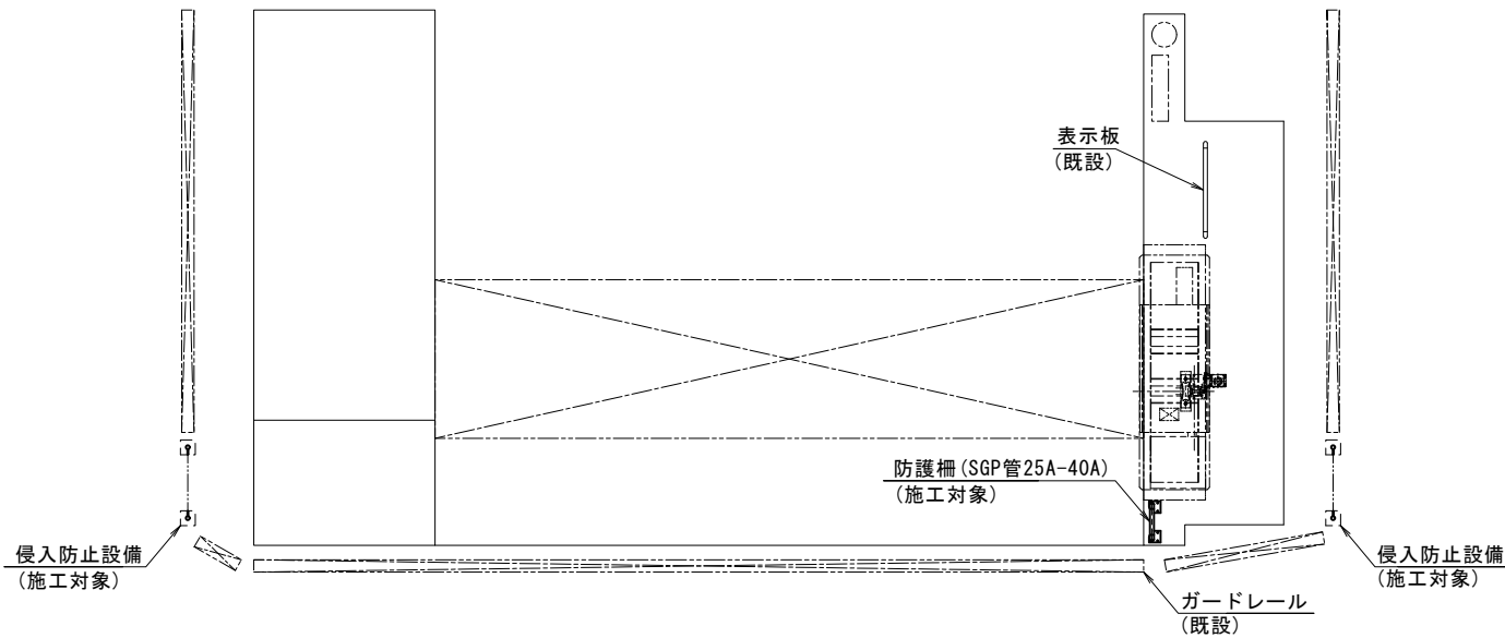
平面図 S=1:50
