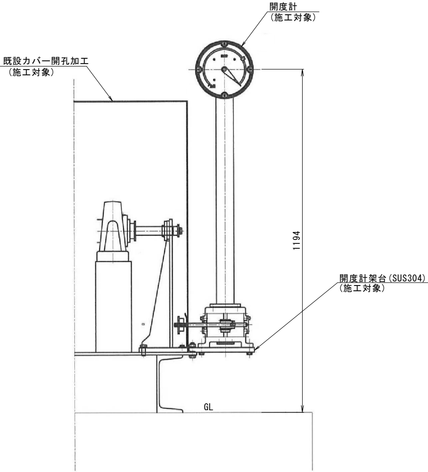
A-A断面
