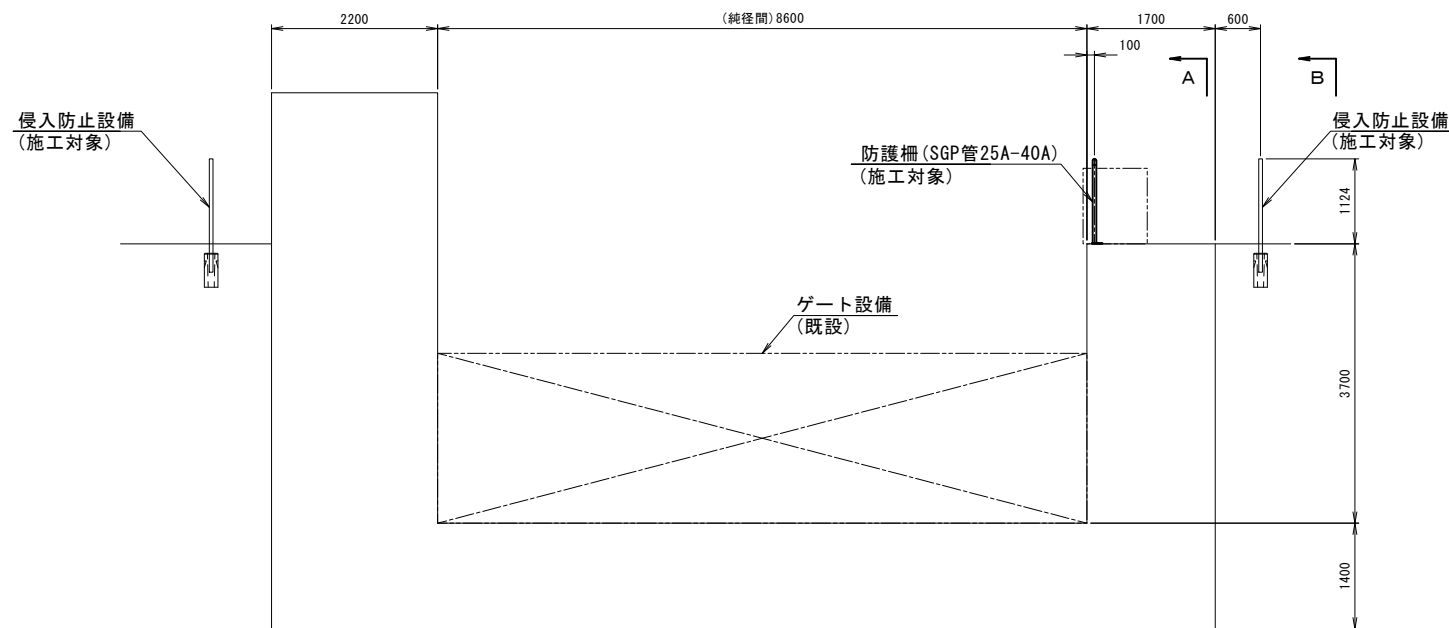
正面図 S=1:50
