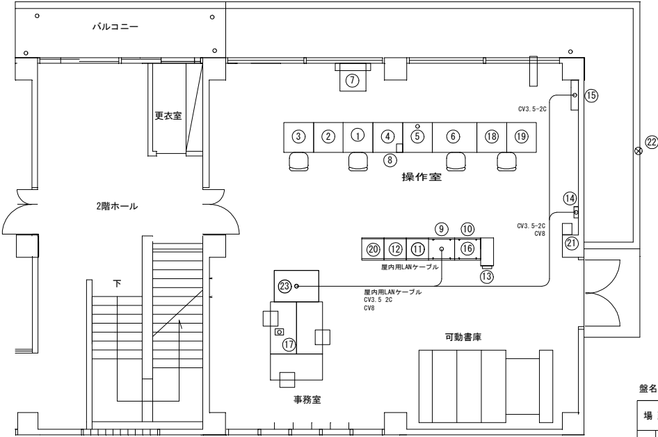
2階平面図
