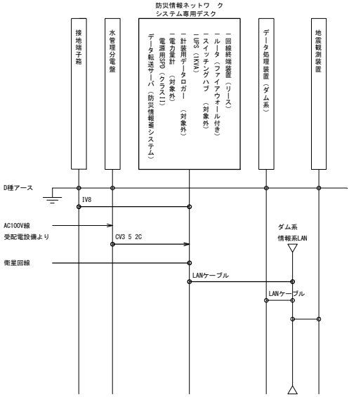
配線系統図
