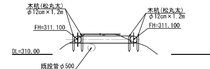
仮設配管時
