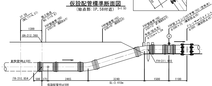
仮設配管標準断面図
