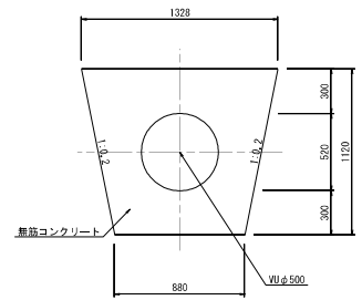
スラストブロック取壊し断面図 S=1:20
