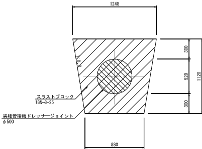
スラストブロック工構造図
