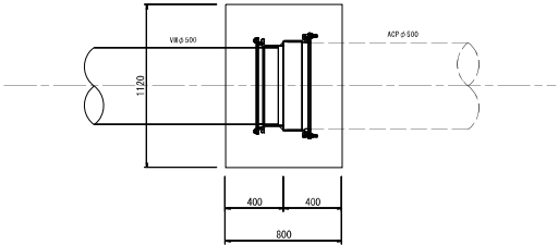
縦断図
