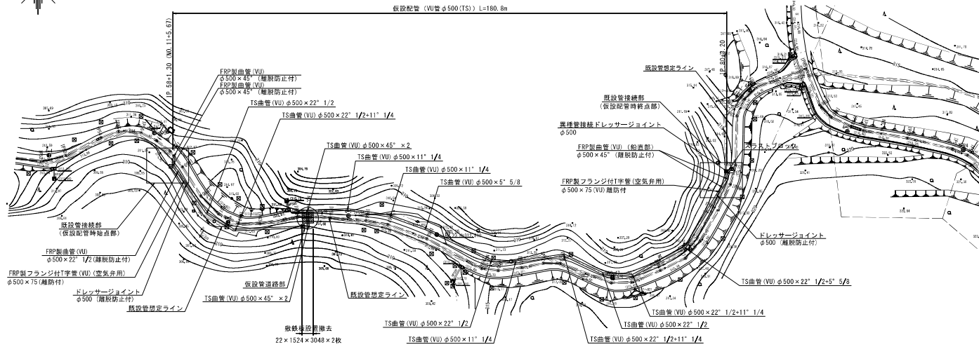
仮設配管平面図
