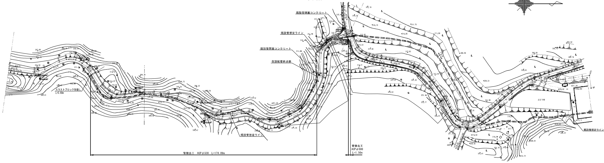
平面図 S=1:500
