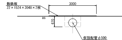
敷鉄板設置撤去標準断面図
