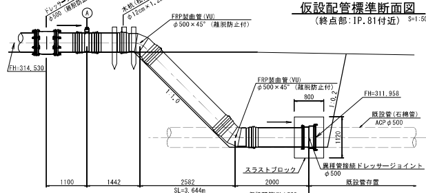
仮設配管標準断面図
