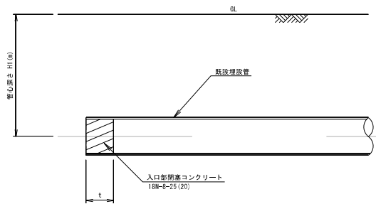
閉塞コンクリート詳細図 Non scale
