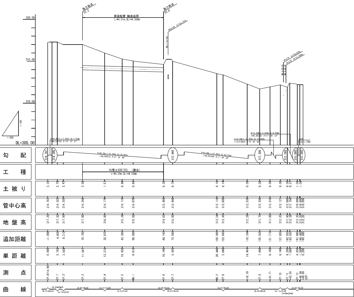
縦断面図 S=1:100(V) S=1:500(H)
