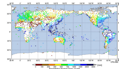
世界の年降水量の分布
