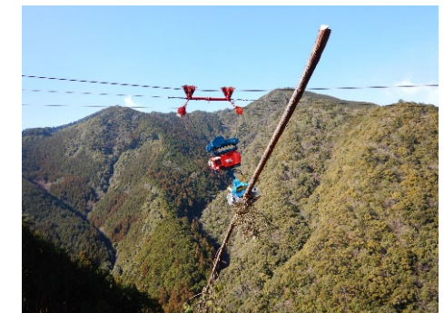
遠隔操作が可能な架線式グラップルと油圧集材機による「新たな架線集材システム」を開発
