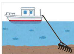
〔海底耕うん〕
